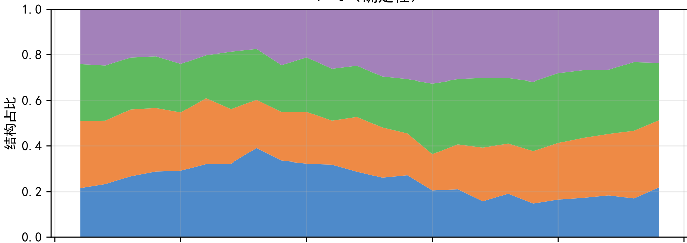
\Gamma=0 (确定性)
