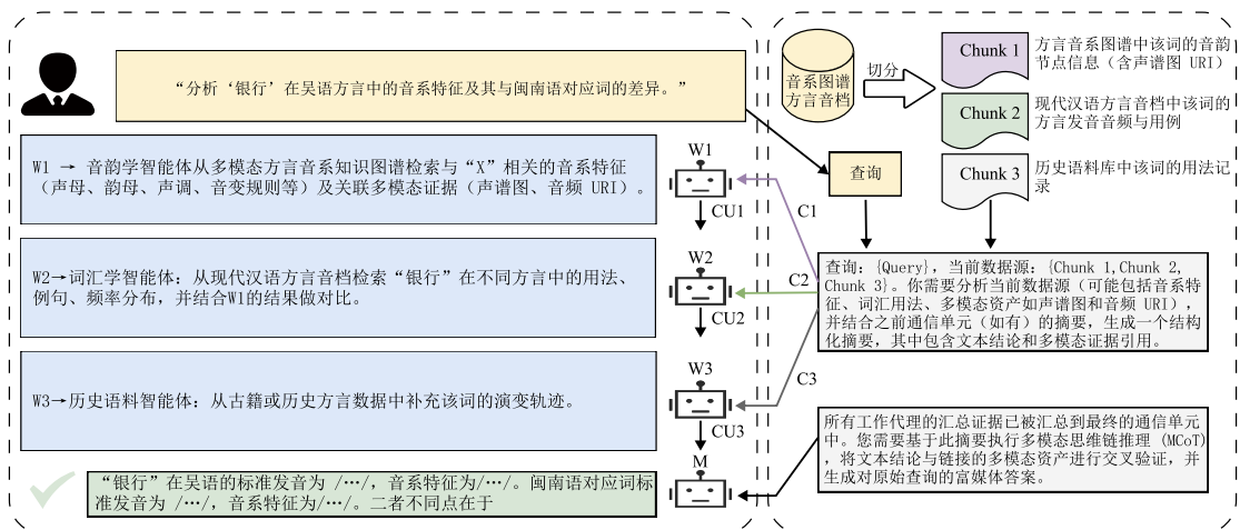
图 4.1 文脉智能体框架示意图
