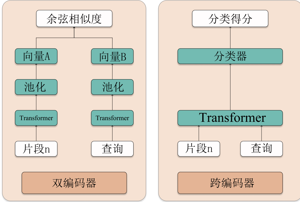
图 6.2 跨编码器与双编码器架构对比图
