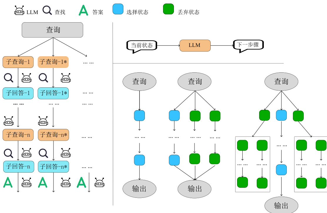
图 5.1 自适应多步检索生成概览图
