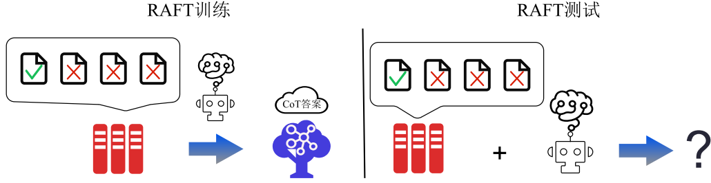
图 6.3 RAFT 概览
