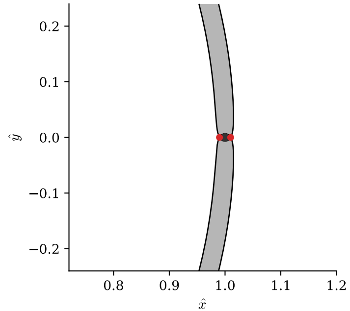
Sun-Earth \mu=3.004\text{e-}06 , JC=3.000889
