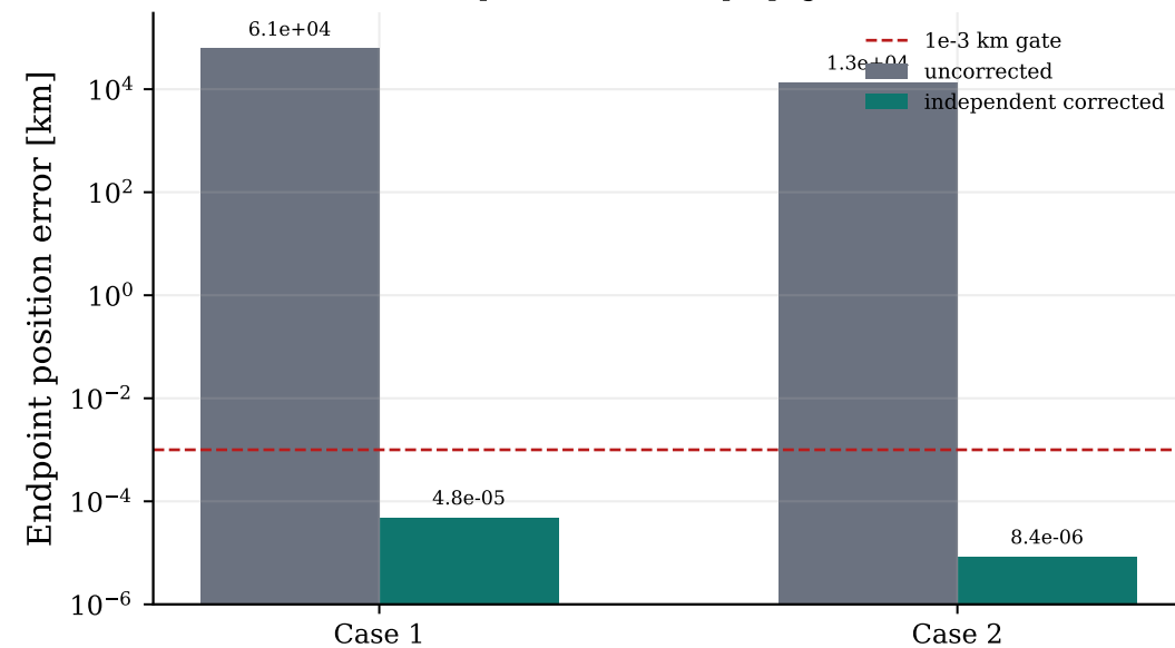
(d) Independent terminal propagation audit
