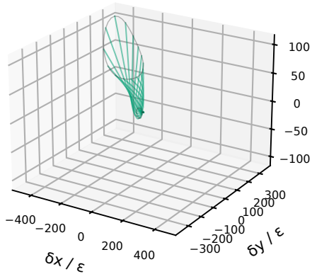
c QR/SVD cocycle
