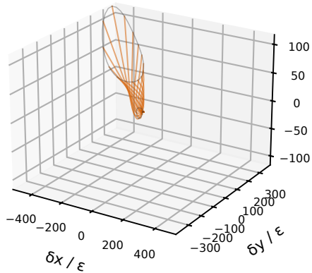
a Pointwise eig
