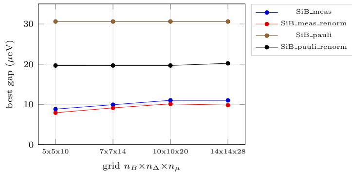
(d) hole-platform optimizer-grid convergence
