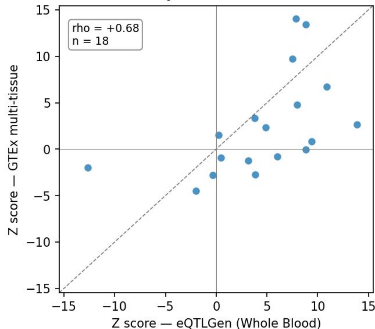
A. Source axis (HK) eQTLGen vs GTEx
