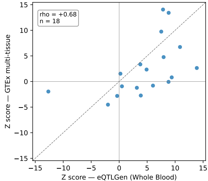
A. Source axis (HK) eQTLGen vs GTEx
