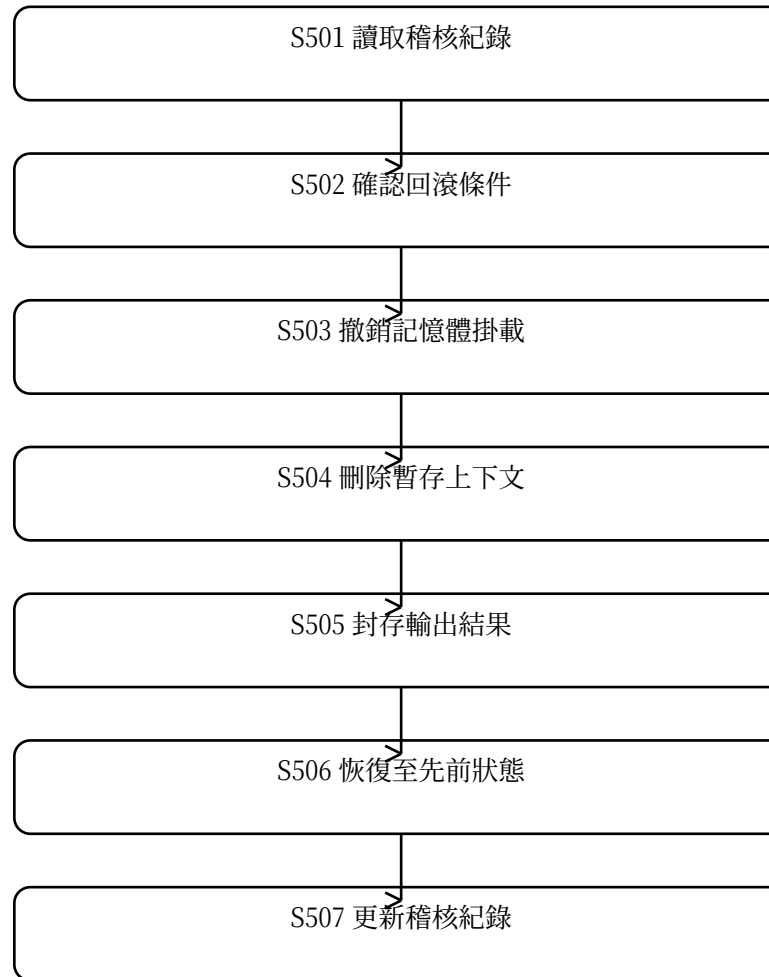
稽核紀錄與回滾流程示意圖
