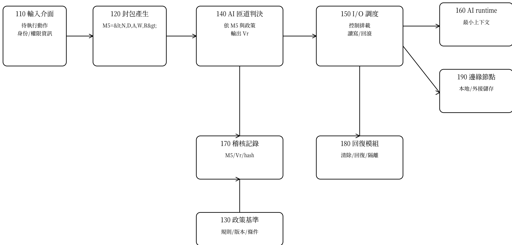
系統架構方塊圖
