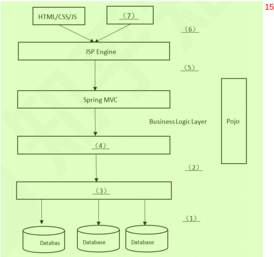
图 5-1 SSM 框架工作流程图 16
