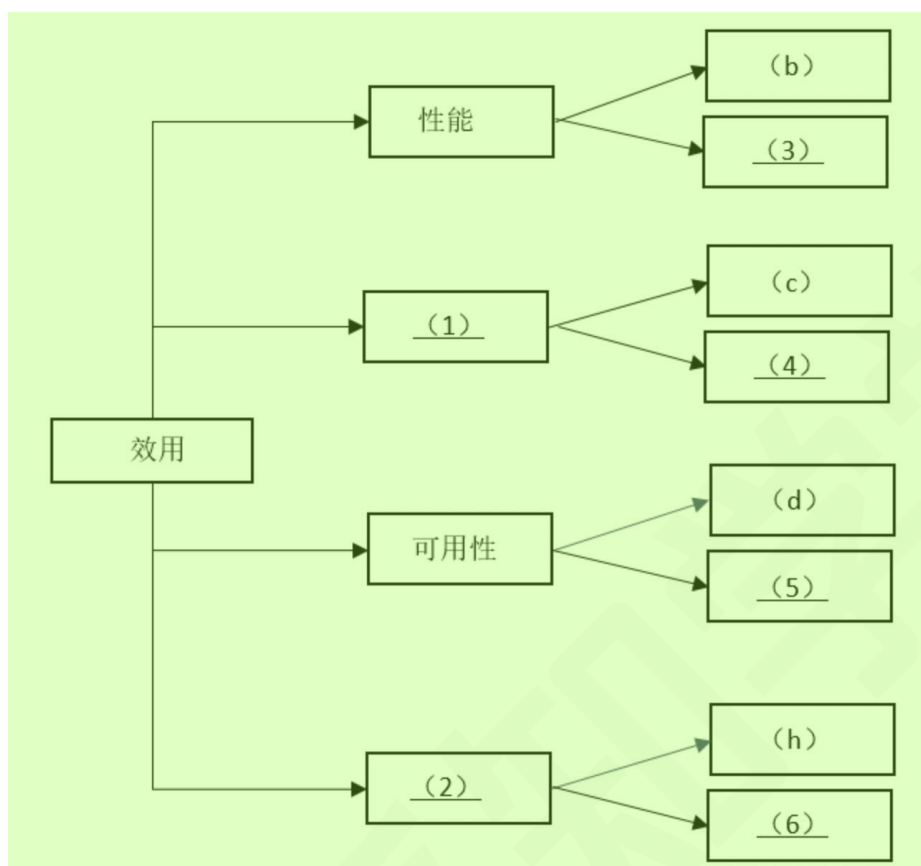
图 1-2 效用树
