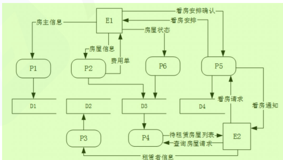
图 2-1 房屋租赁服务系统顶层 DFD 12
