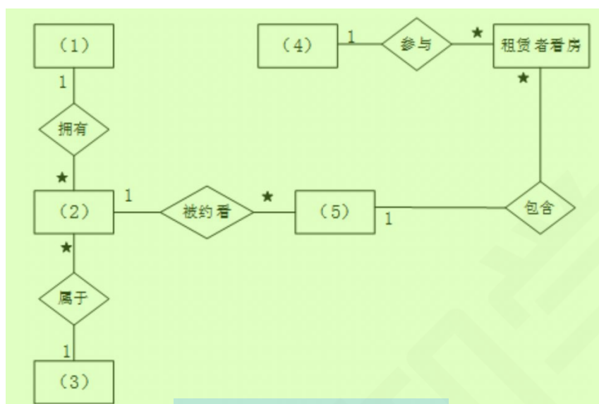
图 2-2 房屋租赁服务系统 ERD 4
