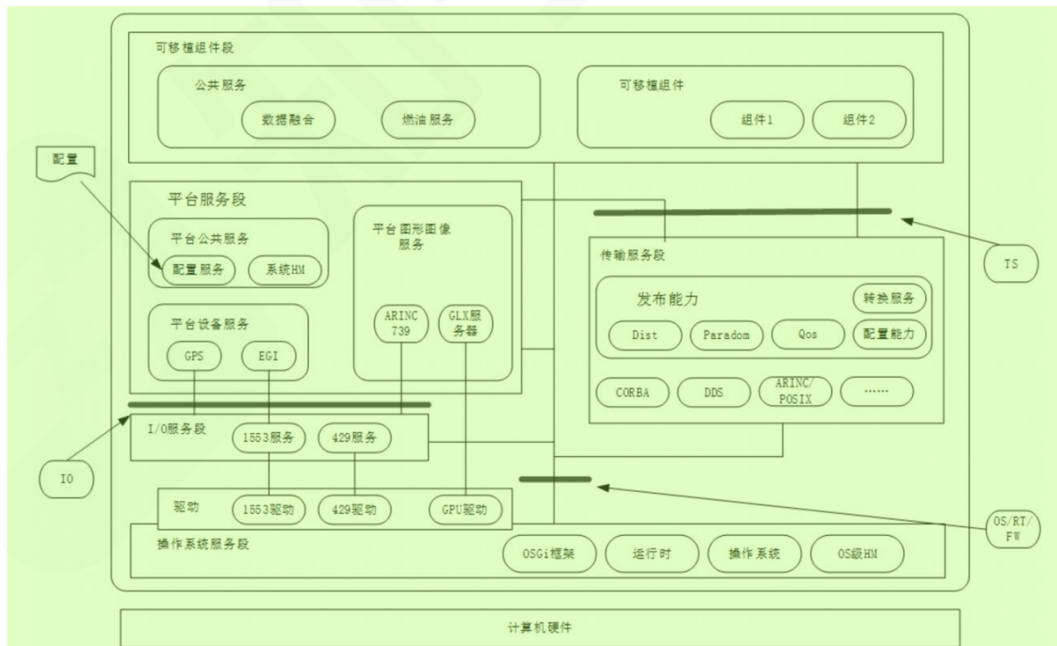
图 3-1 FACE 架构 12
