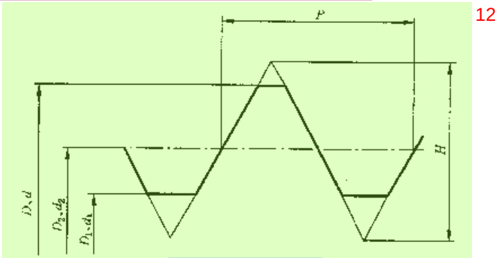
图 1 基本尺寸 13
