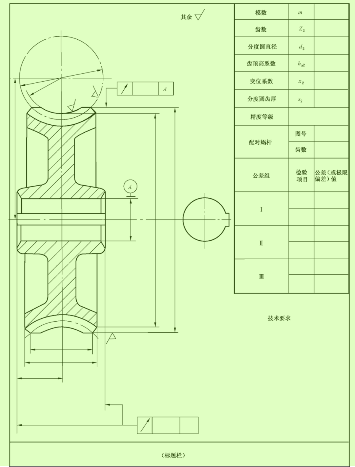
图 A.4 蜗轮图样格式示例 3
