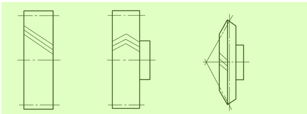
图 8 齿线的表示法 3
