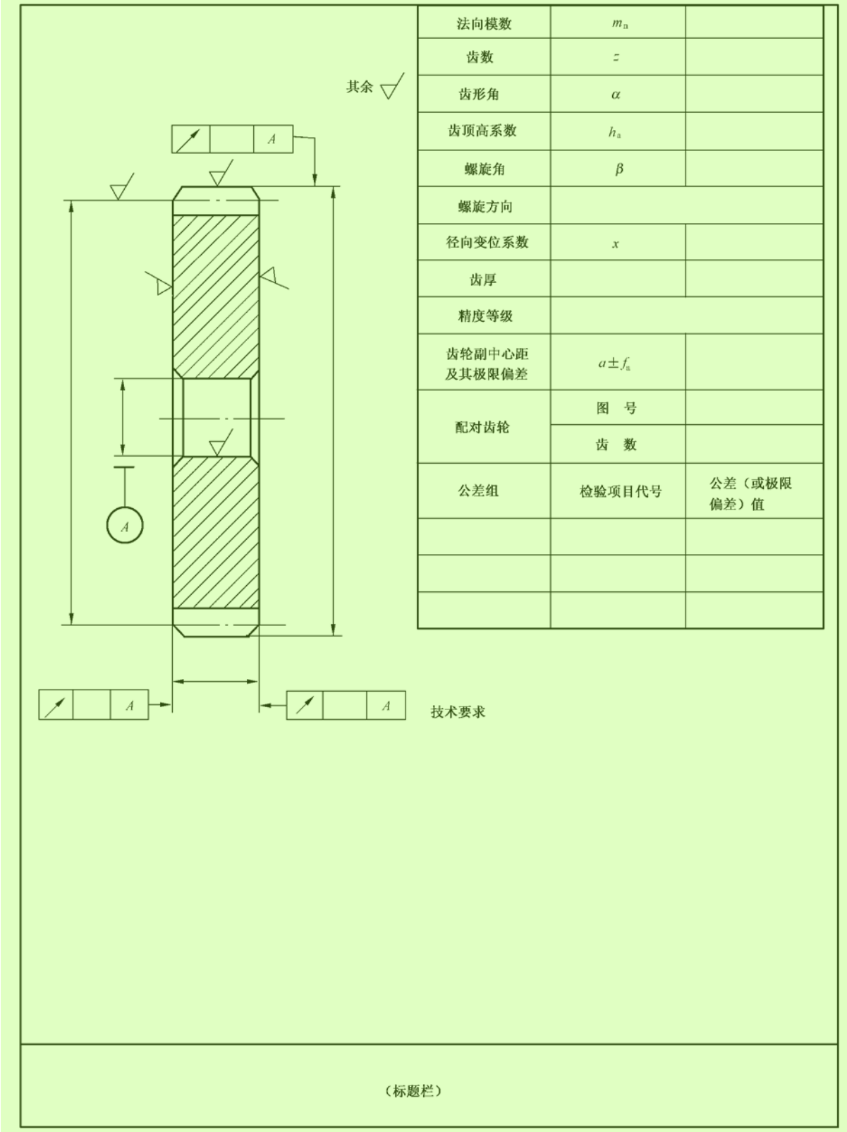
图 A.1 渐开线圆柱齿轮图样格式示例3
