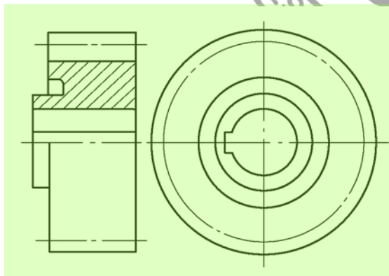
图 1 圆柱齿轮画法 18
