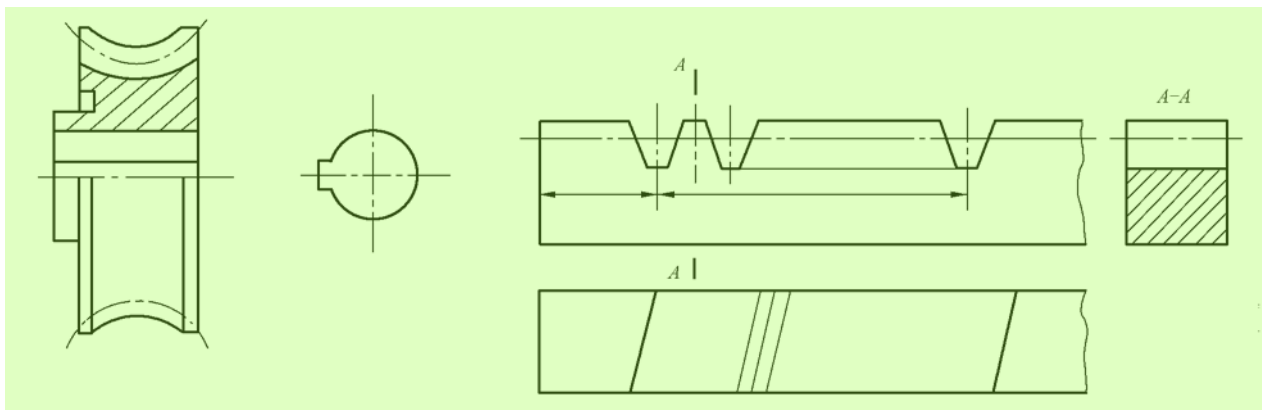
图 3 蜗轮画法 2
