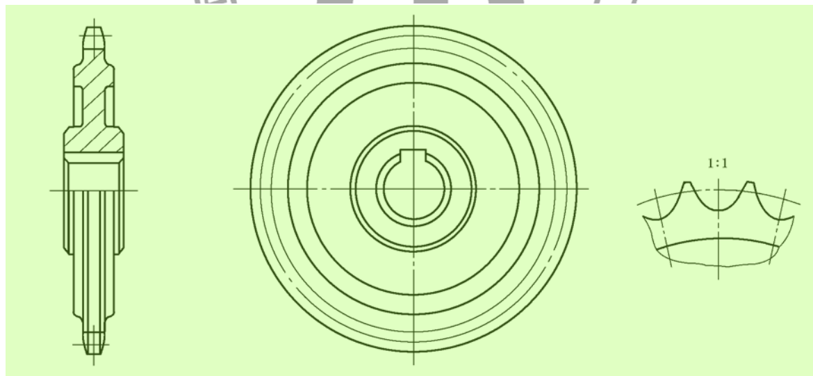
图 7 链轮画法 7
