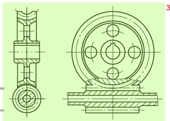
图 22 圆柱蜗杆副的啮合画法(二)
