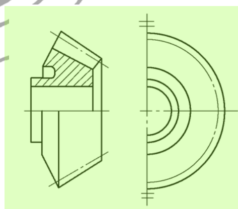
图 2 锥齿轮画法 20
