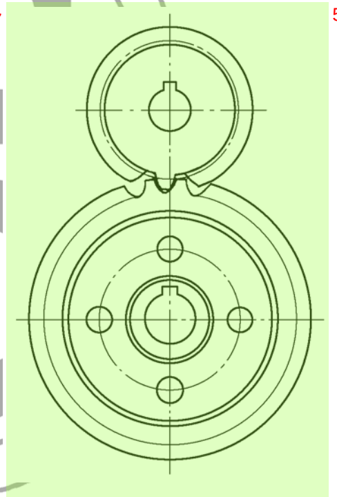
图 24 圆弧齿轮副的啮合画法
