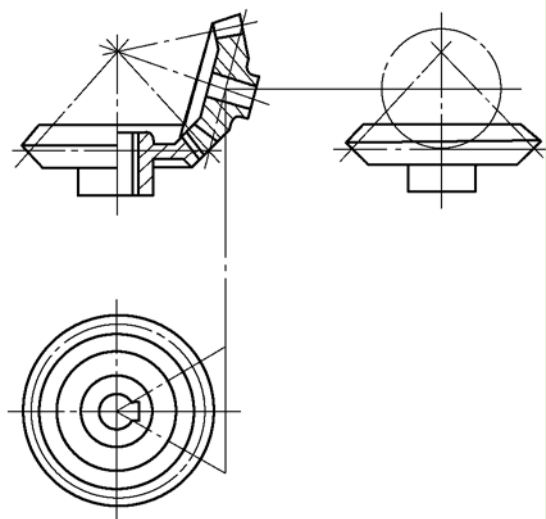
图 17 轴线斜交的锥齿轮副的啮合画法 6
