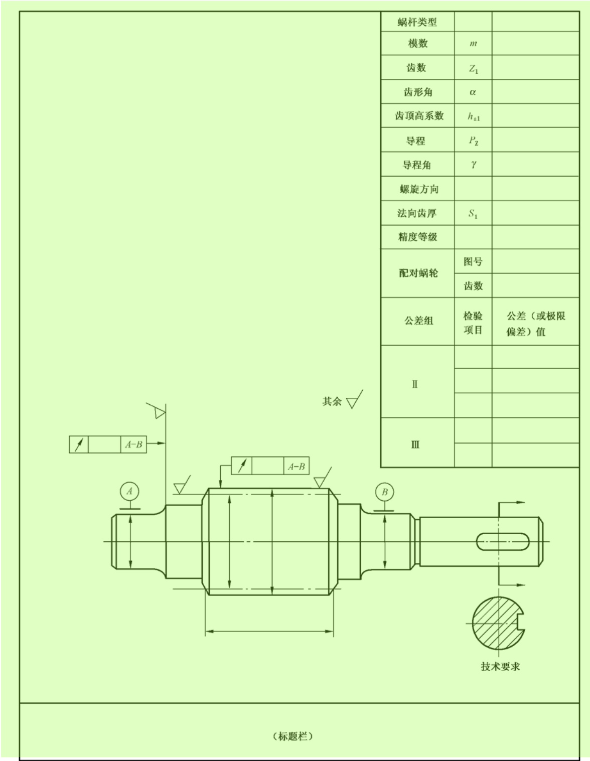
图 A.3 蜗杆图样格式示例 3
