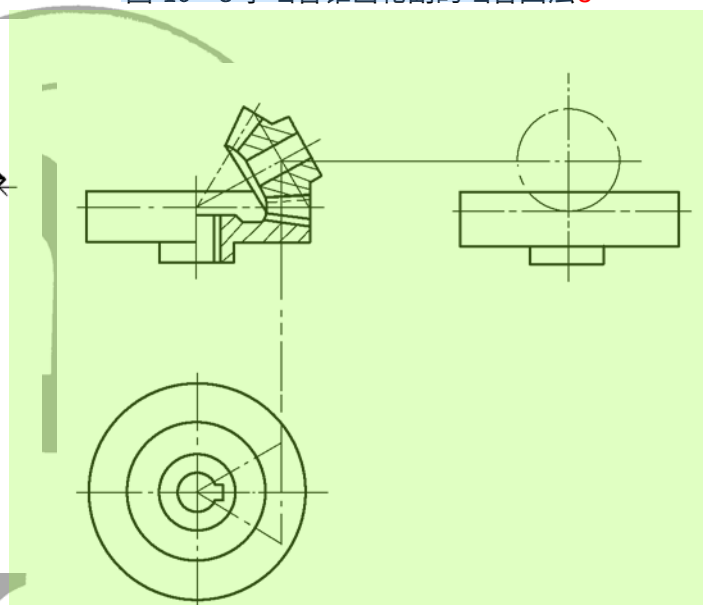
图 18 轴线斜交的平面齿轮与锥齿轮的啮合画法 5
