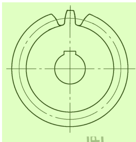
图 5 表明齿形的圆柱齿轮画法 4
