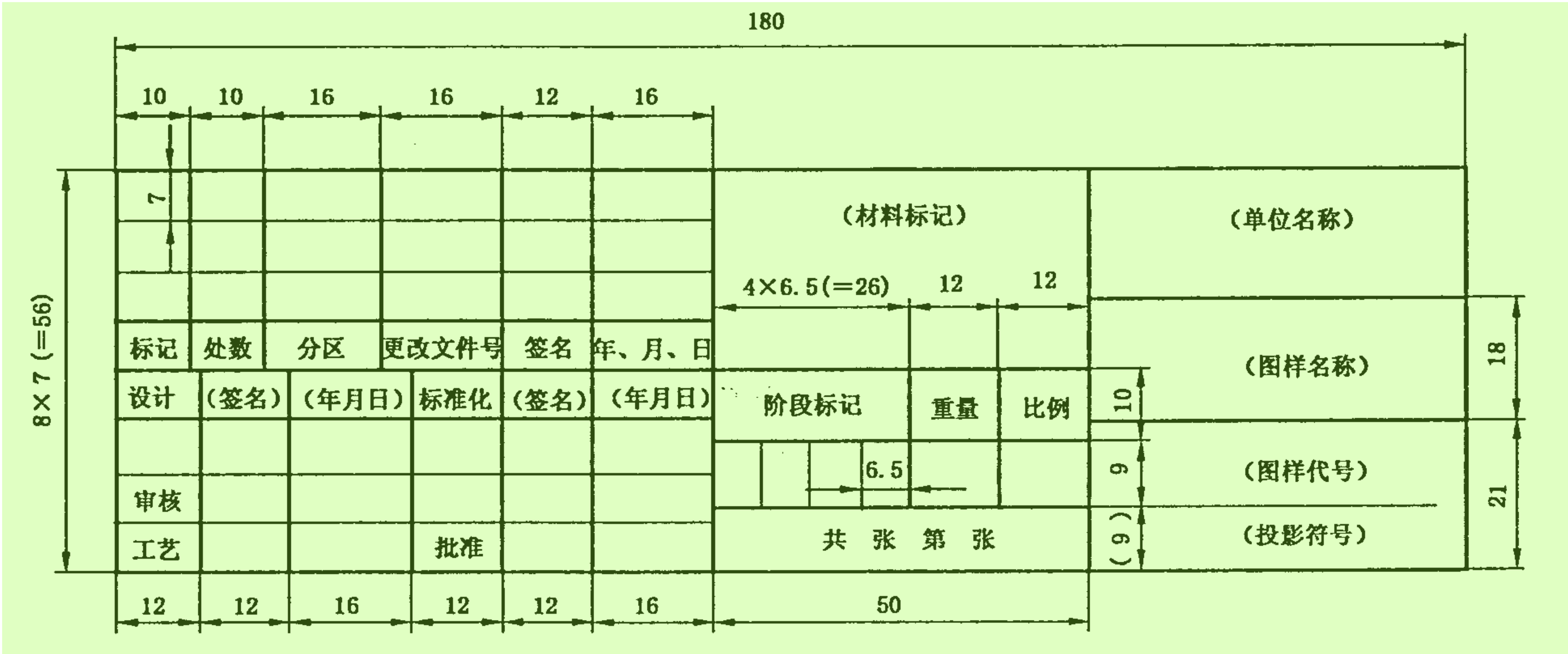
图 A. 1 标题栏的格式
