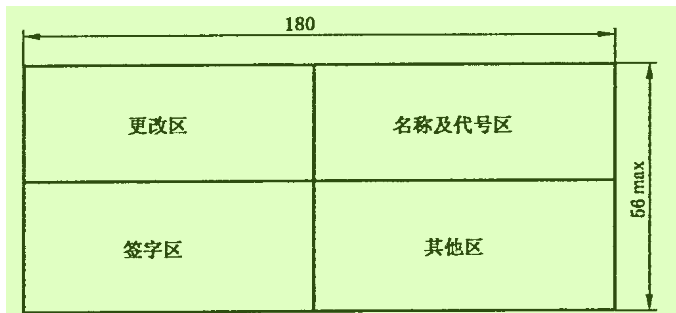
图 3 标题栏的分区(二) 24
