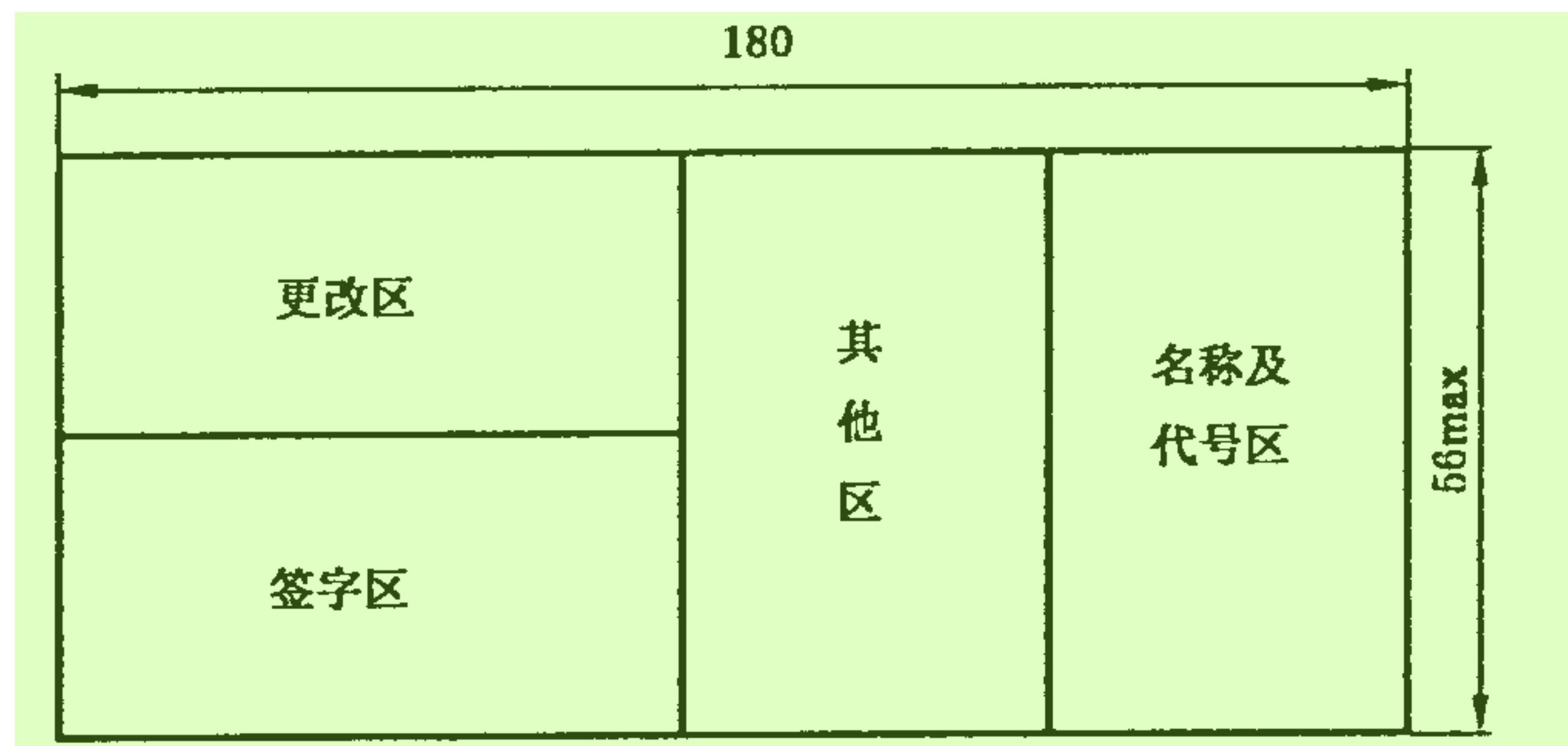
图 2 标题栏的分区(一) 22
