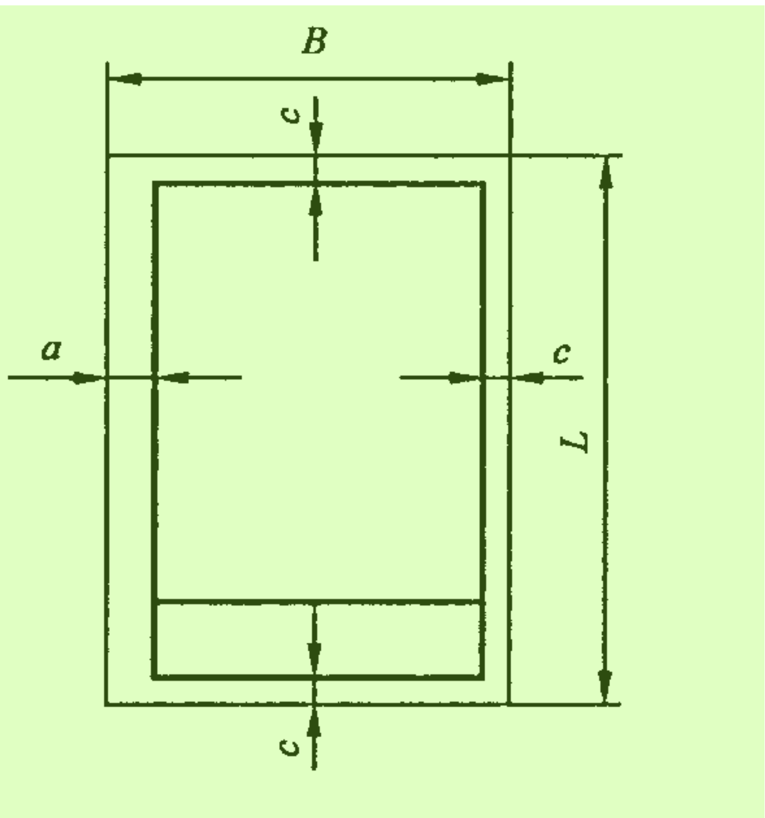
图 5 有装订边图纸(Y 型)的图框格式
