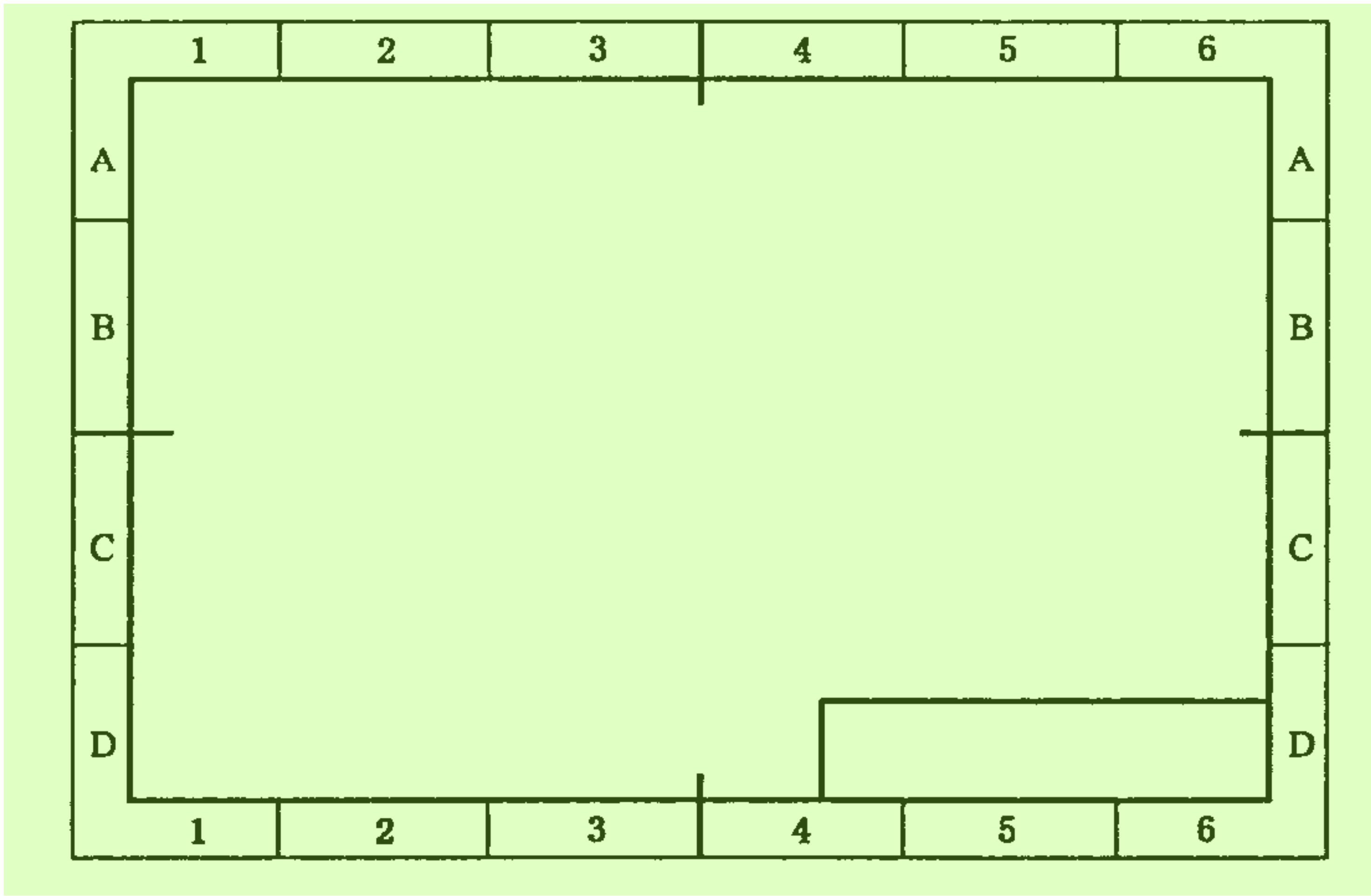
图 13 图幅分区(一)
