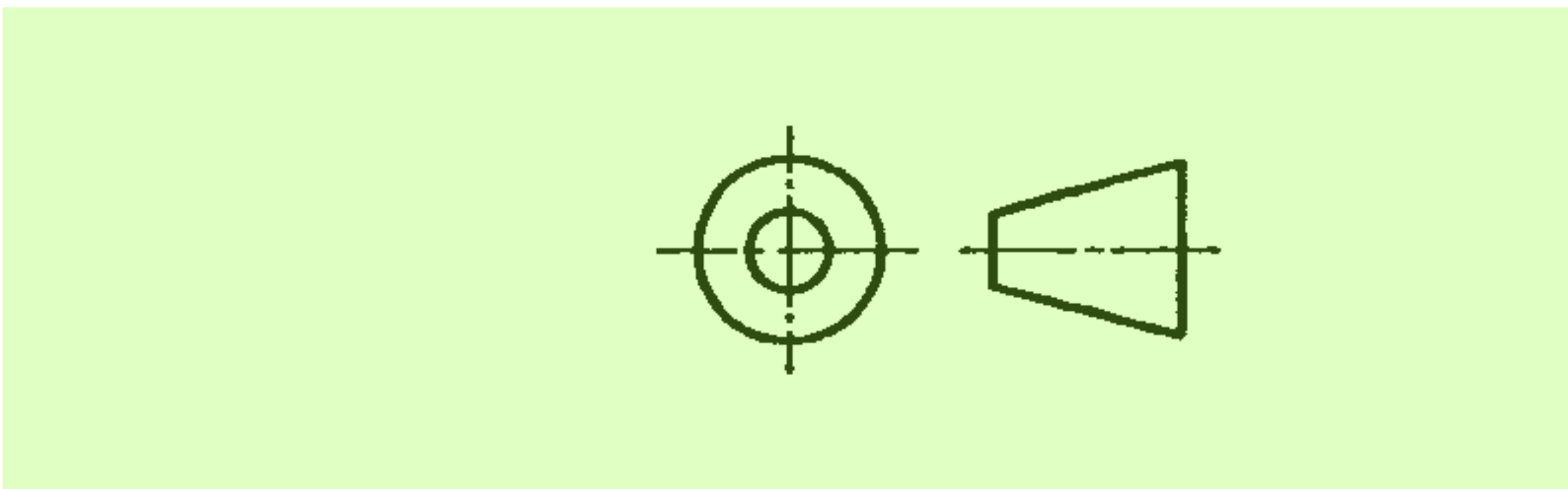
图 12 第三角画法的投影识别符号
