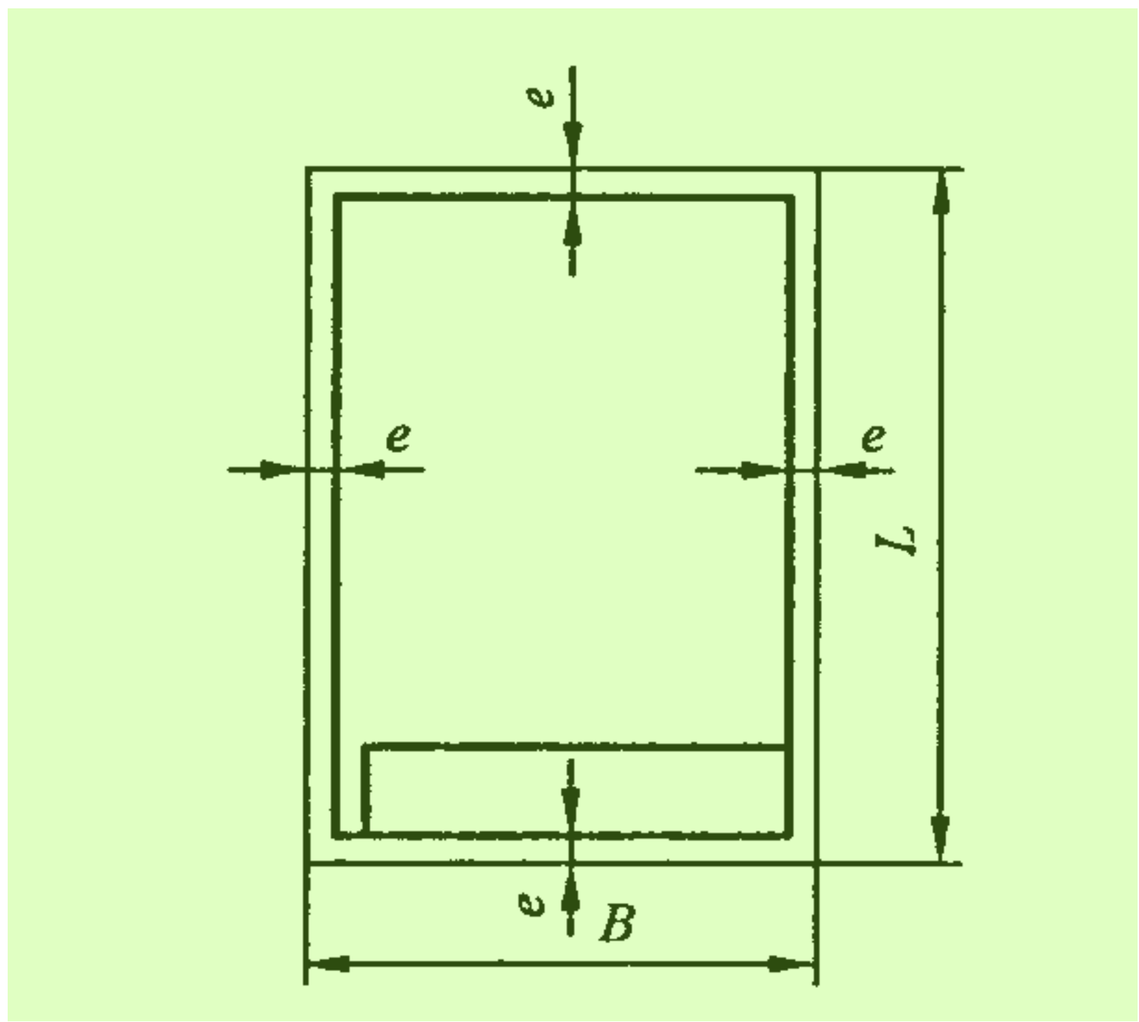
图 3 无装订边图纸(Y 型)的图框格式
