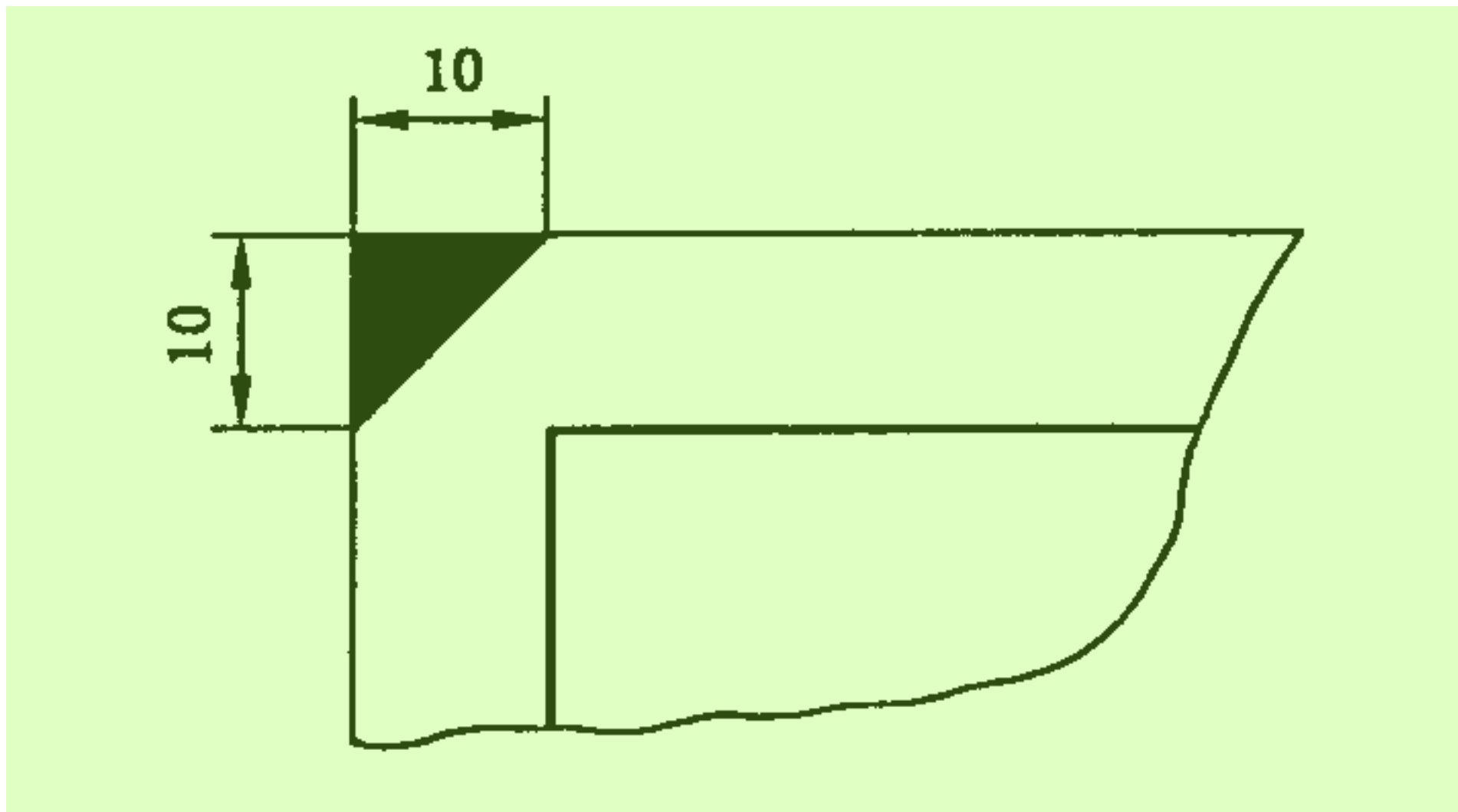
图 9 剪切符号(一)
