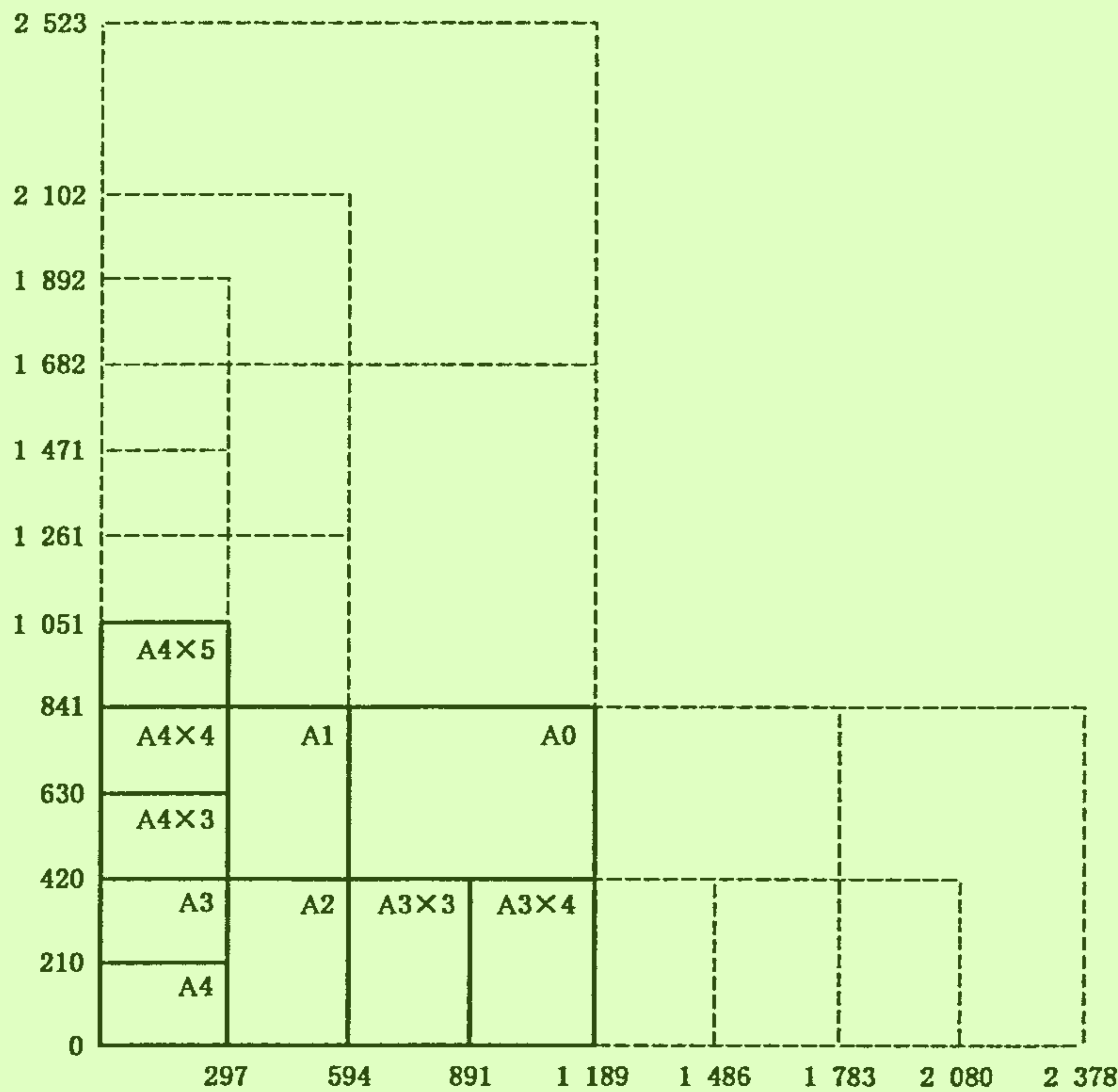
图 1 图纸的幅面尺寸 3
