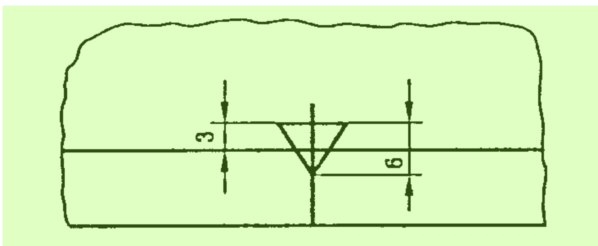
图 8 方向符号的尺寸和位置
