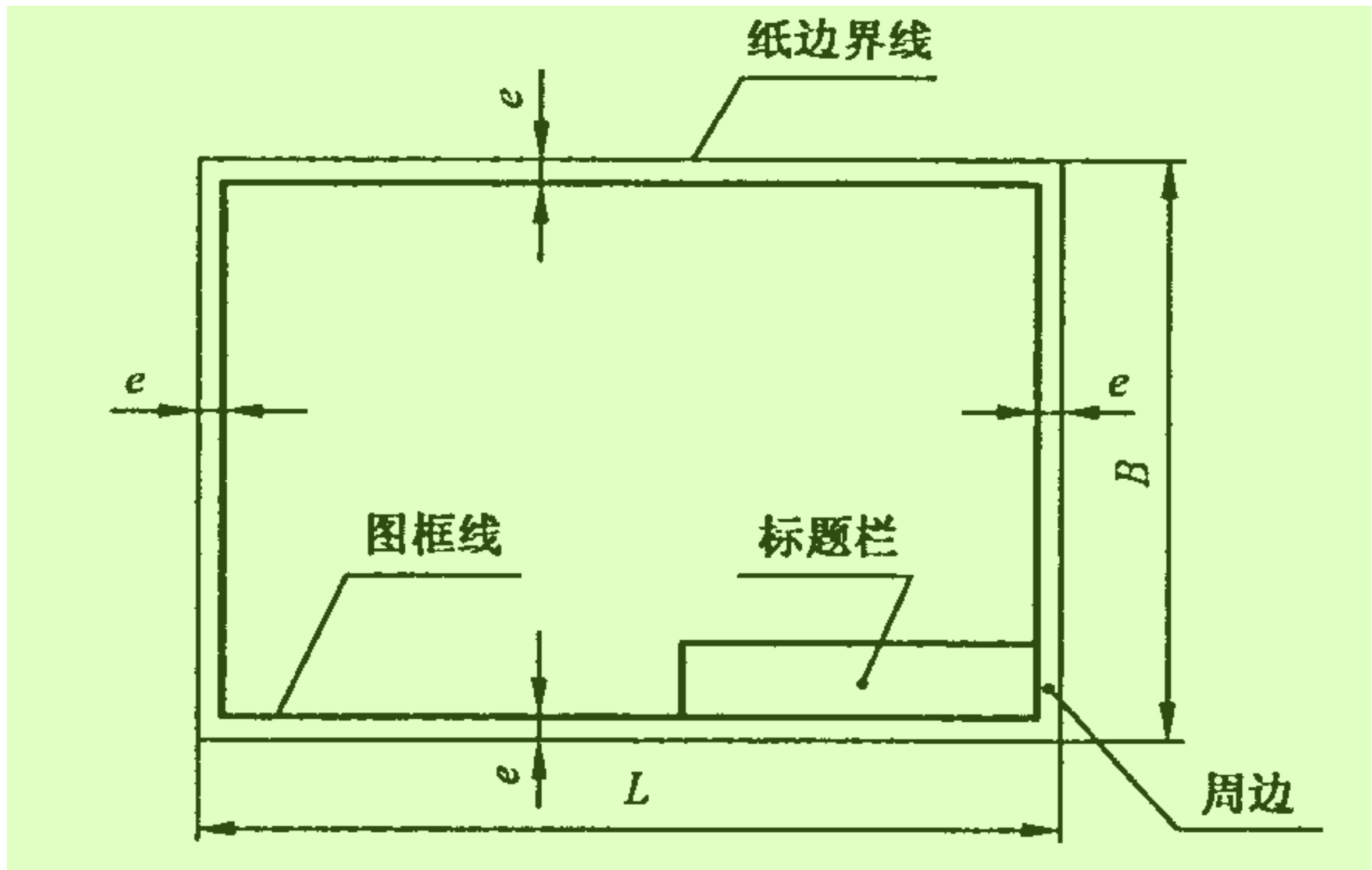
图 2 无装订边图纸(X 型)的图框格式
