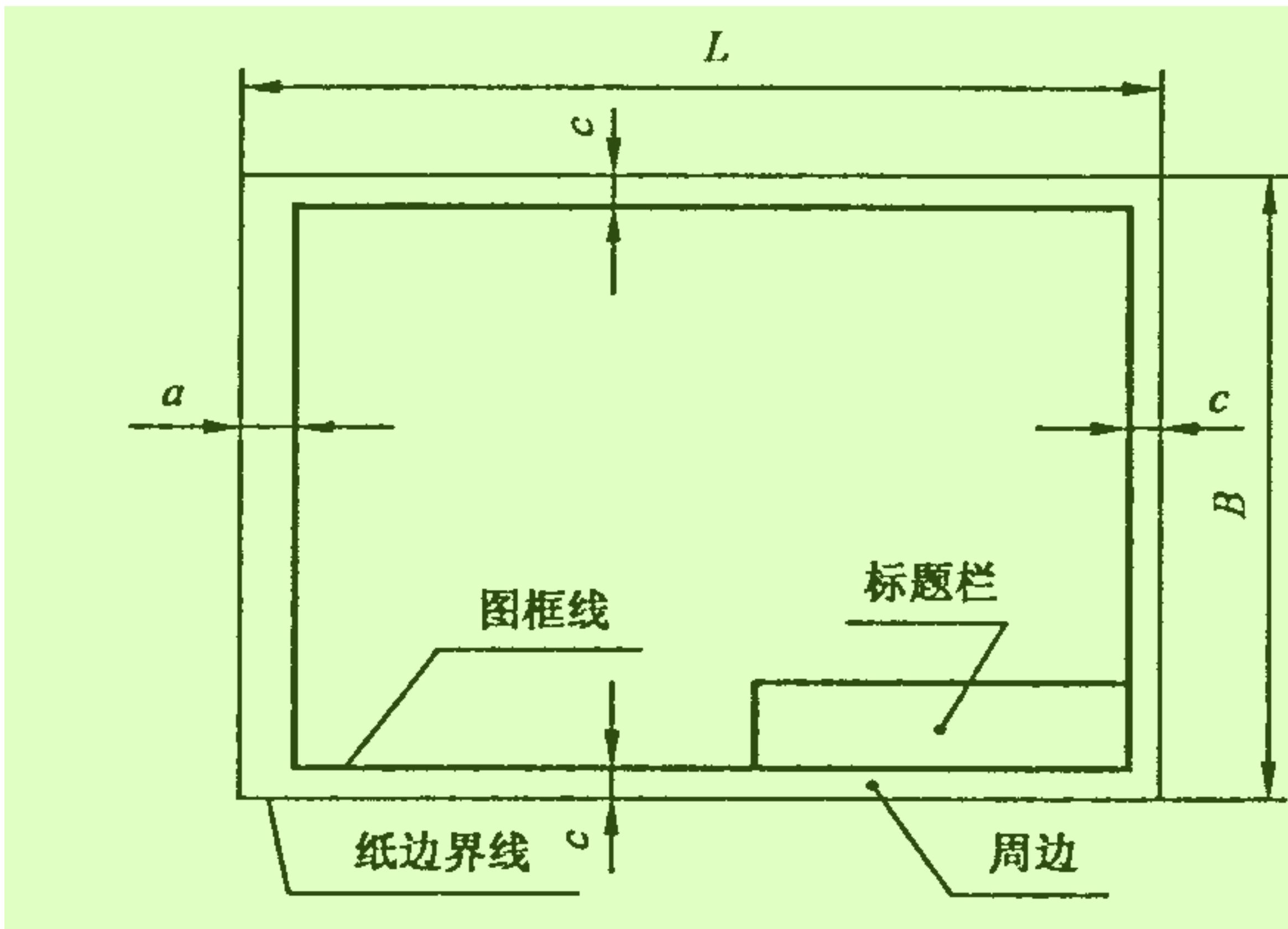
图 4 有装订边图纸(X 型)的图框格式
