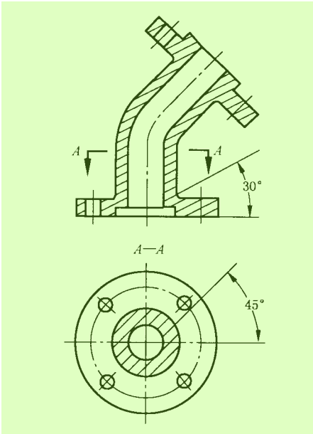
图 2 与主要轮廓线成适当角度剖面线的应用示例
