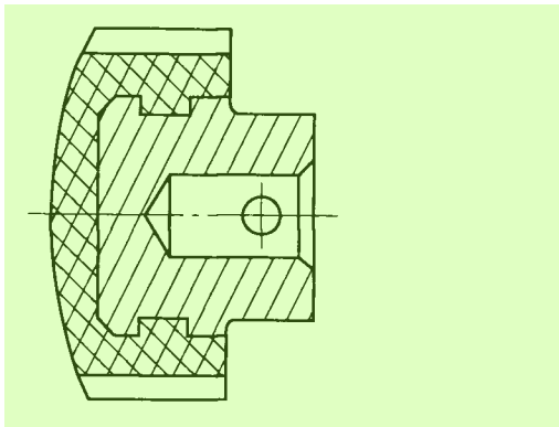
图 8 接合件图中各零件的剖面符号绘制方法(二) 2
