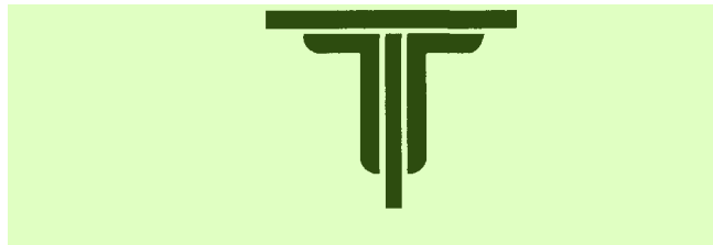
图 12 两邻接剖面区域均涂黑时的画法 4
