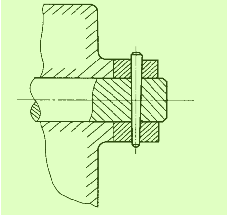
图 4 剖面区域较大时可以只沿轮廓的周边画出剖面符号
