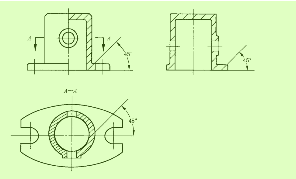
图 1 与主要轮廓线成 45°剖面线的应用示例 6
