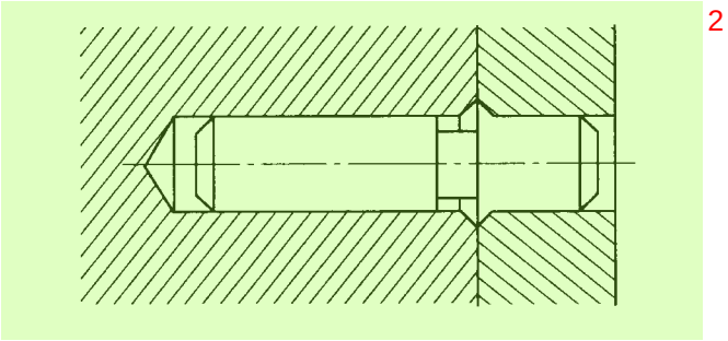
图 5 被剖区域无断裂边界线时的剖面线画法
