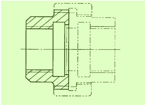
图 3 相邻辅助零件(或部件)不画剖面符号
