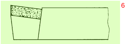
图 6 剖面符号画在工件外形作为材料的标志
