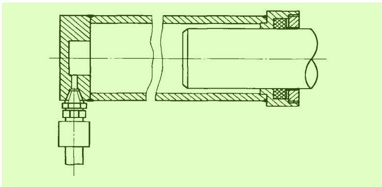
图 10 绘制接合件与其他零件的装配图时剖面符号绘制方法 7
