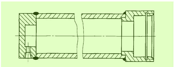
图 9 接合件图中各零件的剖面符号绘制方法(三) 4
