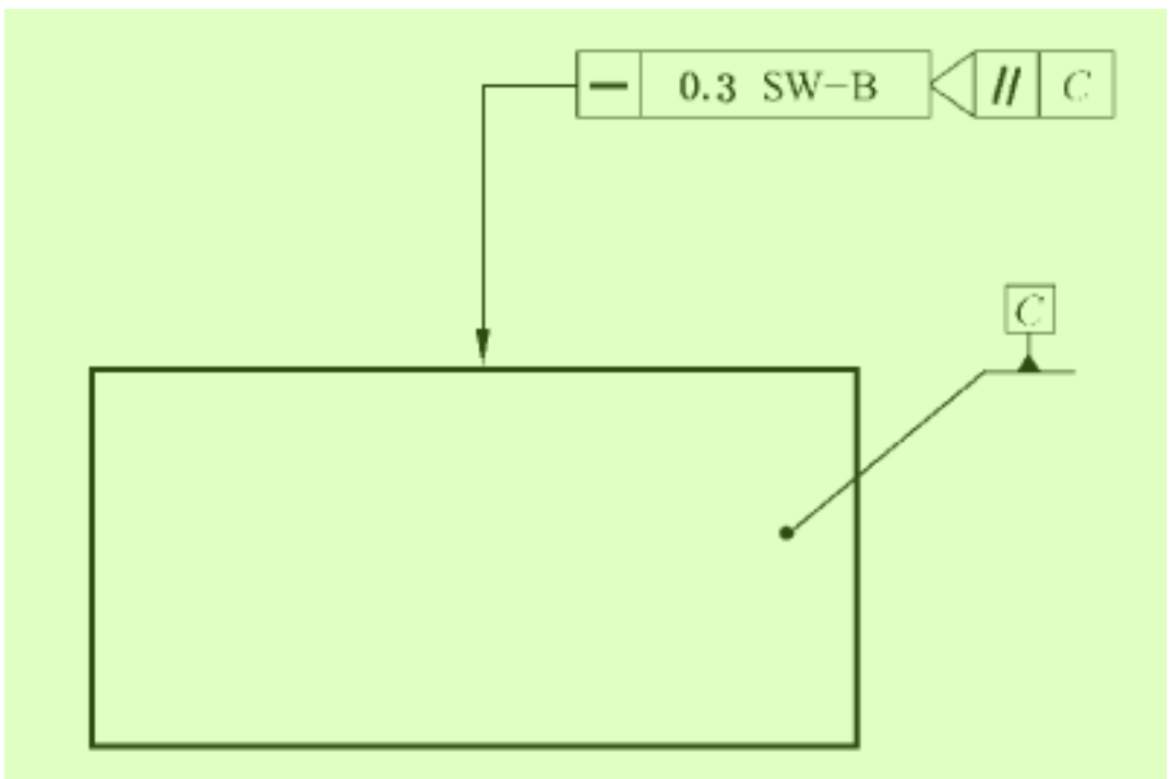
图 E.10 使用短波通滤波器的直线度公差示例
