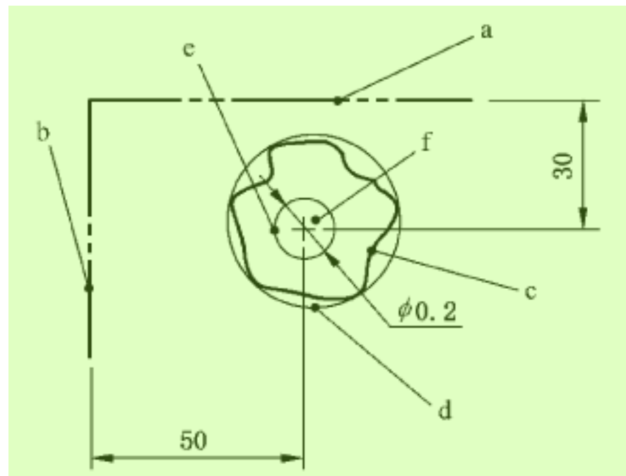
图 29 最小外接拟合被测要素——图样标注
