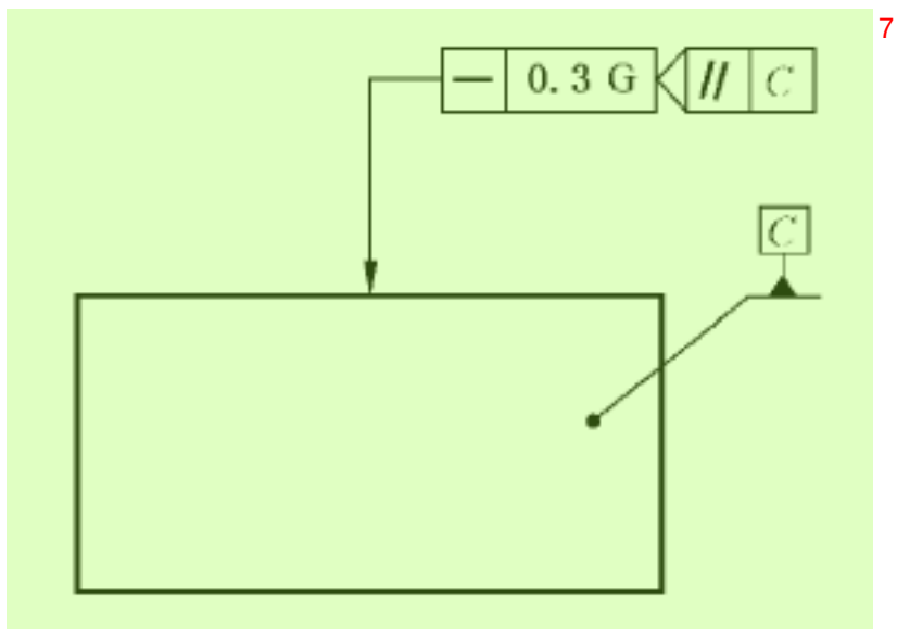
图 41 使用最小二乘(高斯)参照要素规范的规范 8
