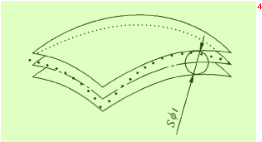
图 109 面轮廓度公差带的定义
