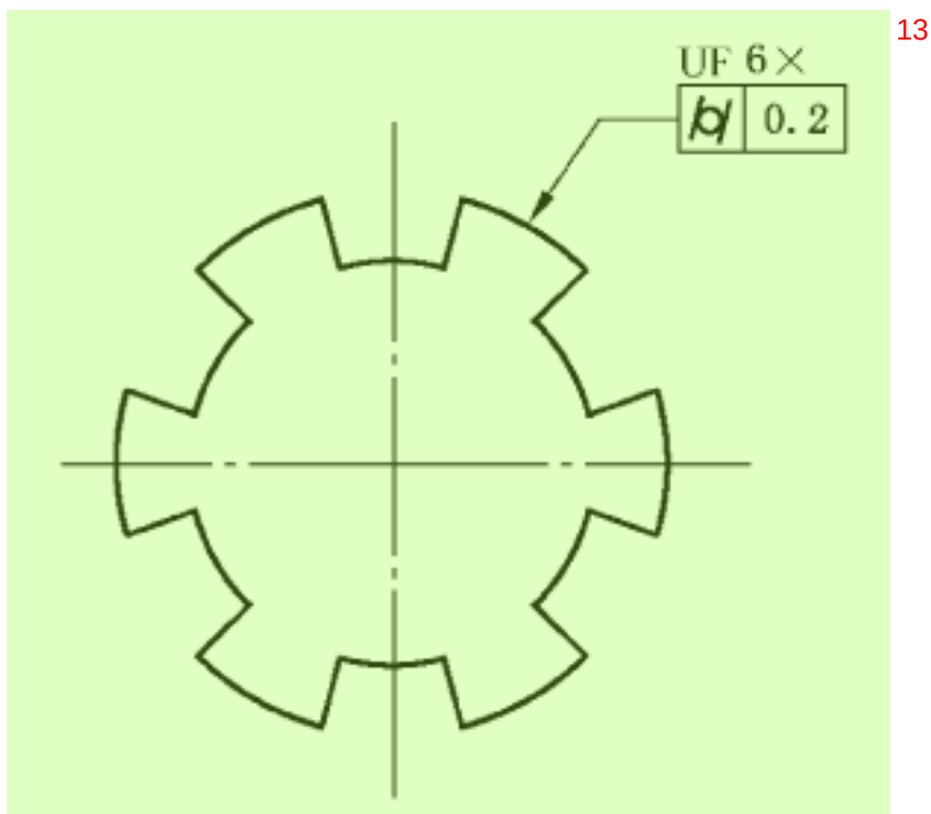
图 48 应用于联合要素的规范标注 12
