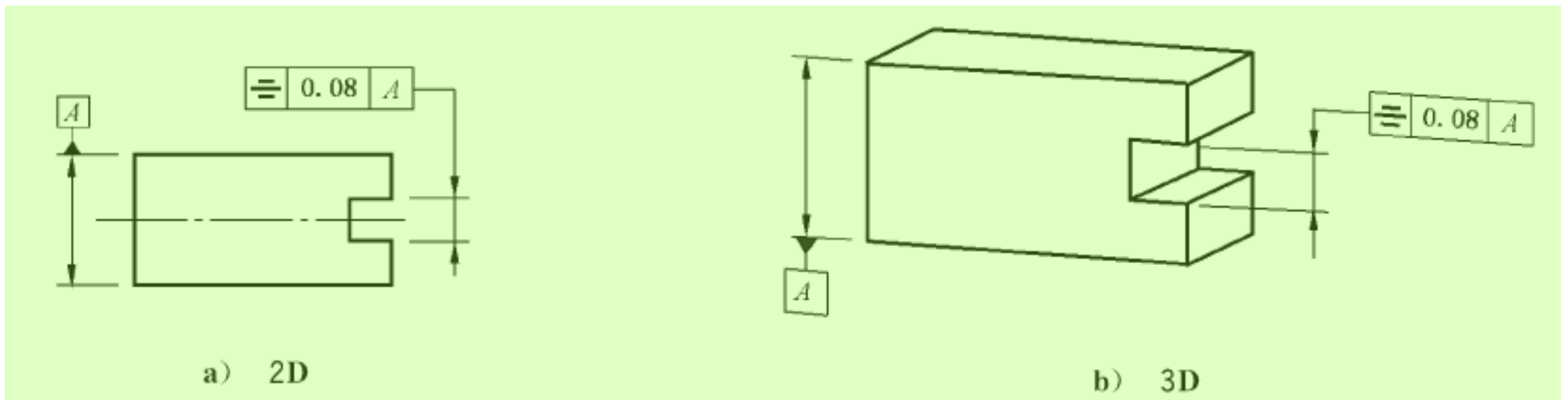
图 169 对称度标注 8
