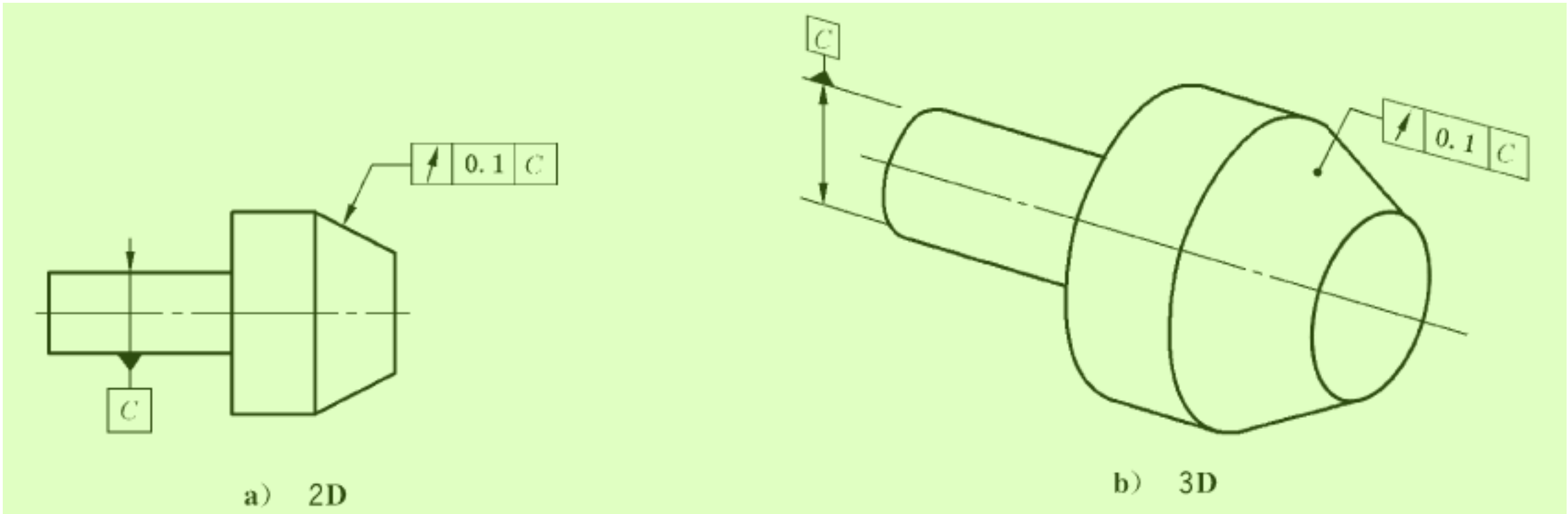
图 179 圆跳动标注 9
