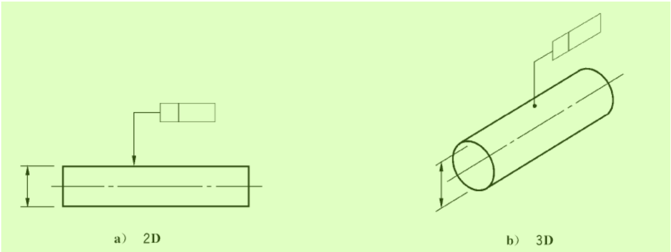
图 2 组成要素的标注
