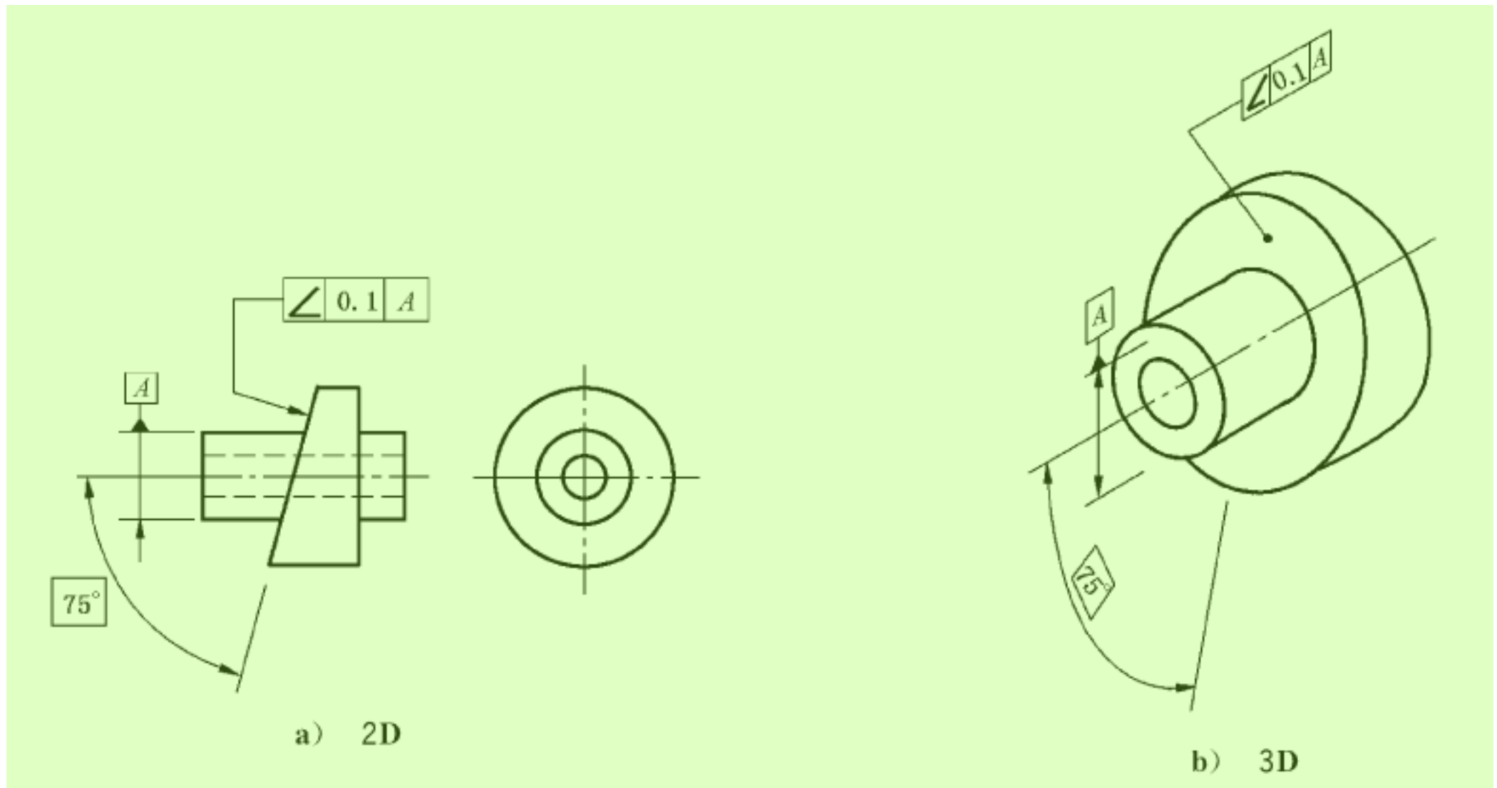
图 146 倾斜度标注
