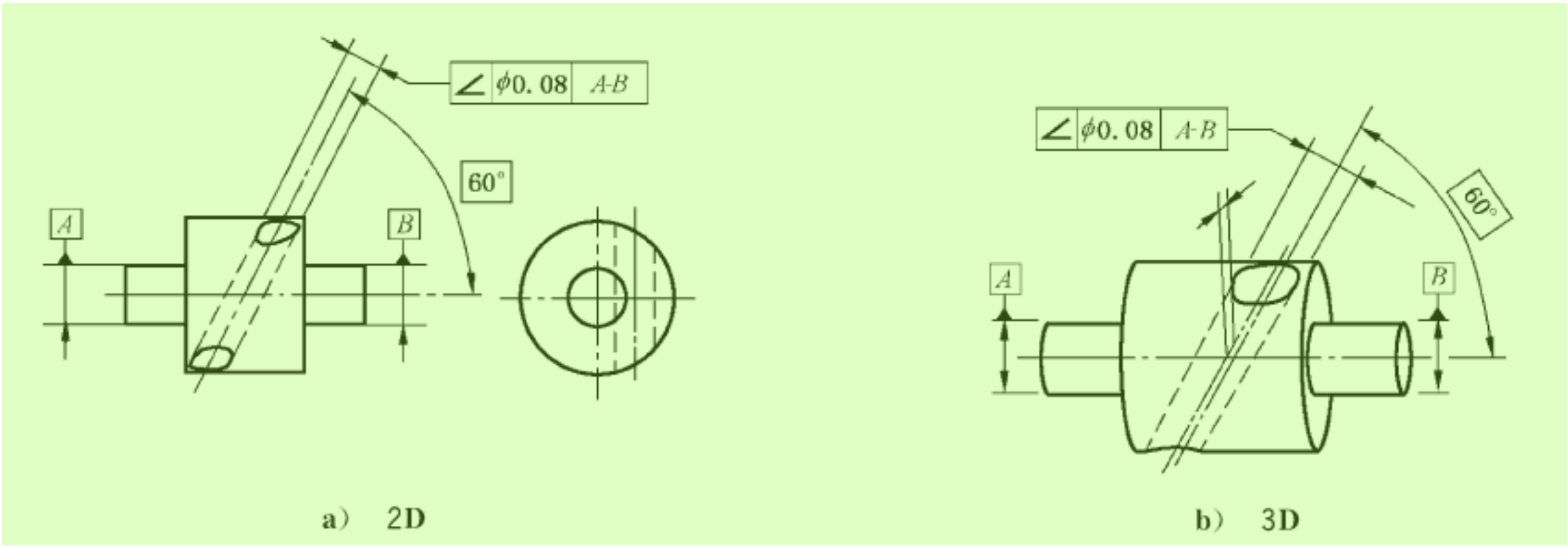
图 140 倾斜度标注 5
