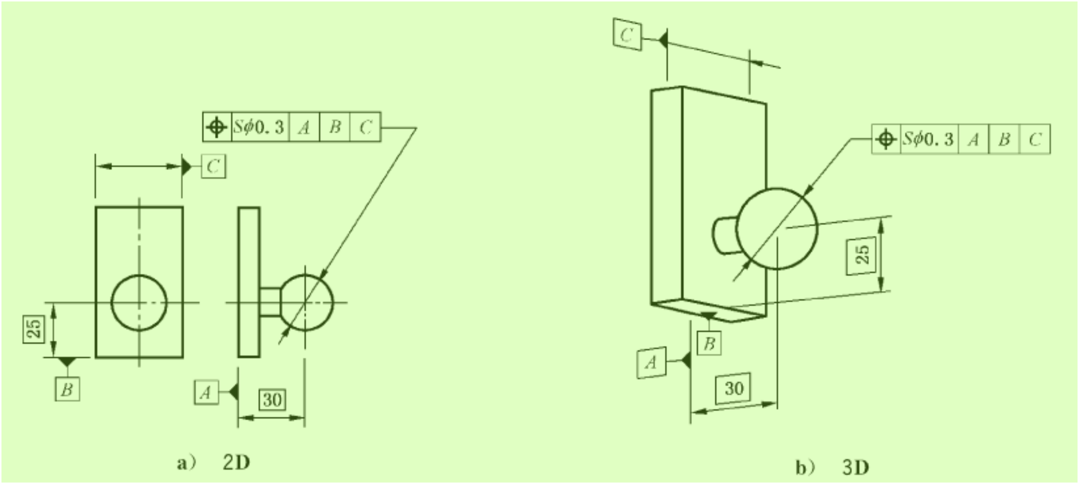
图 150 位置度标注 8
