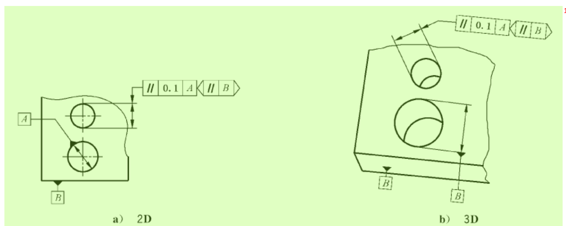
图 112 平行度标注
