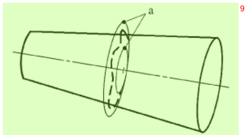
图 101 圆度公差带的定义 10
