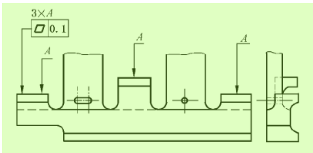
图 18 适用于多个单独要素的规范
