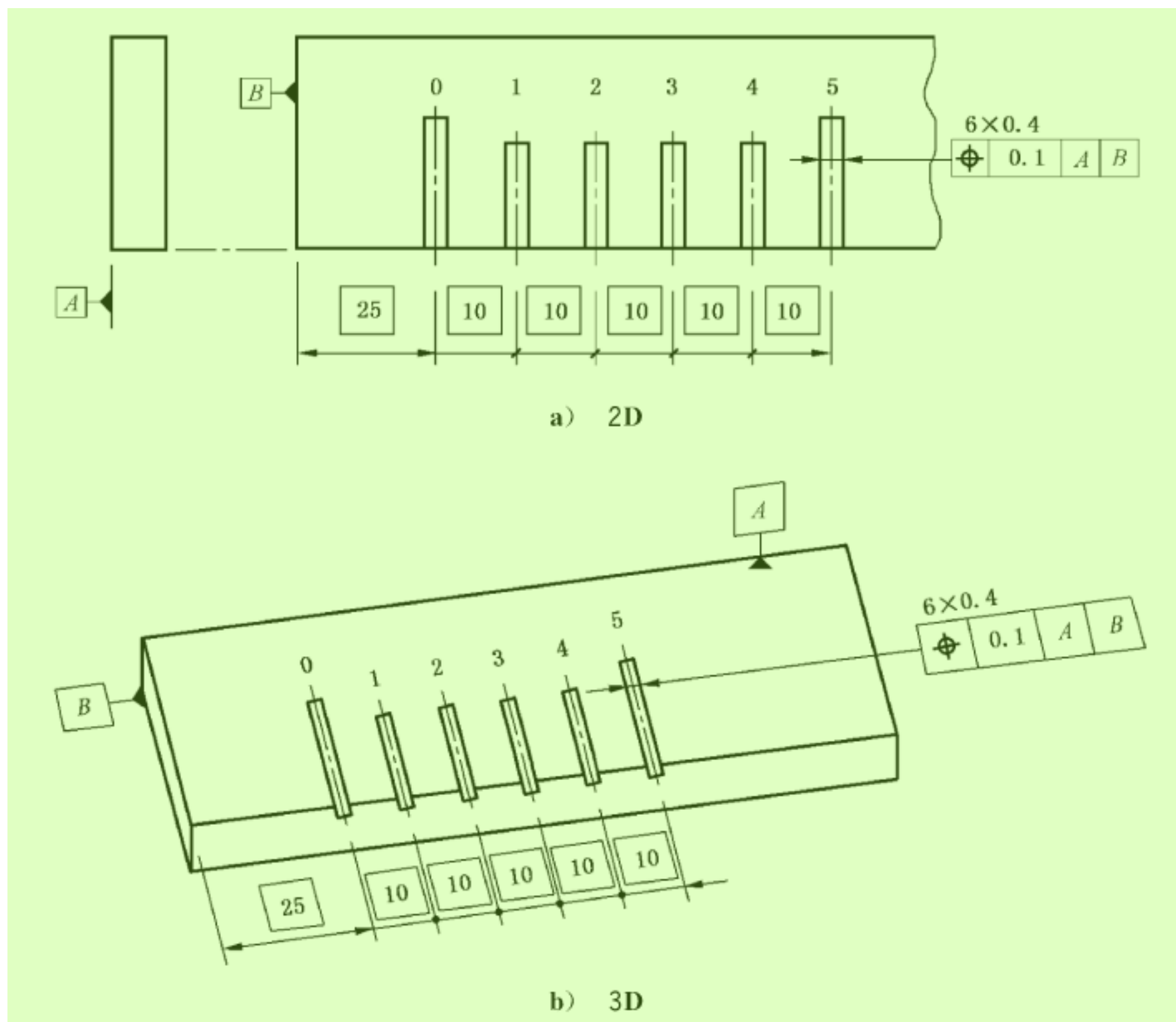
图 157 位置度标注
