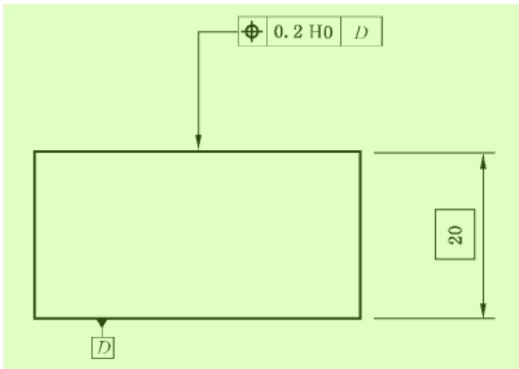
图 E.18 位置度公差示例
