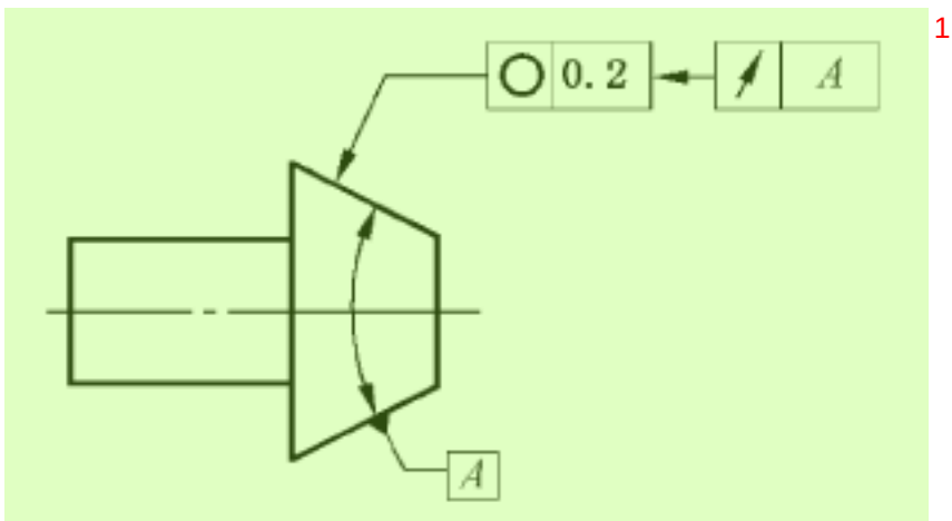
图 88 与被测要素的面要素垂直的圆度公差标注 2
