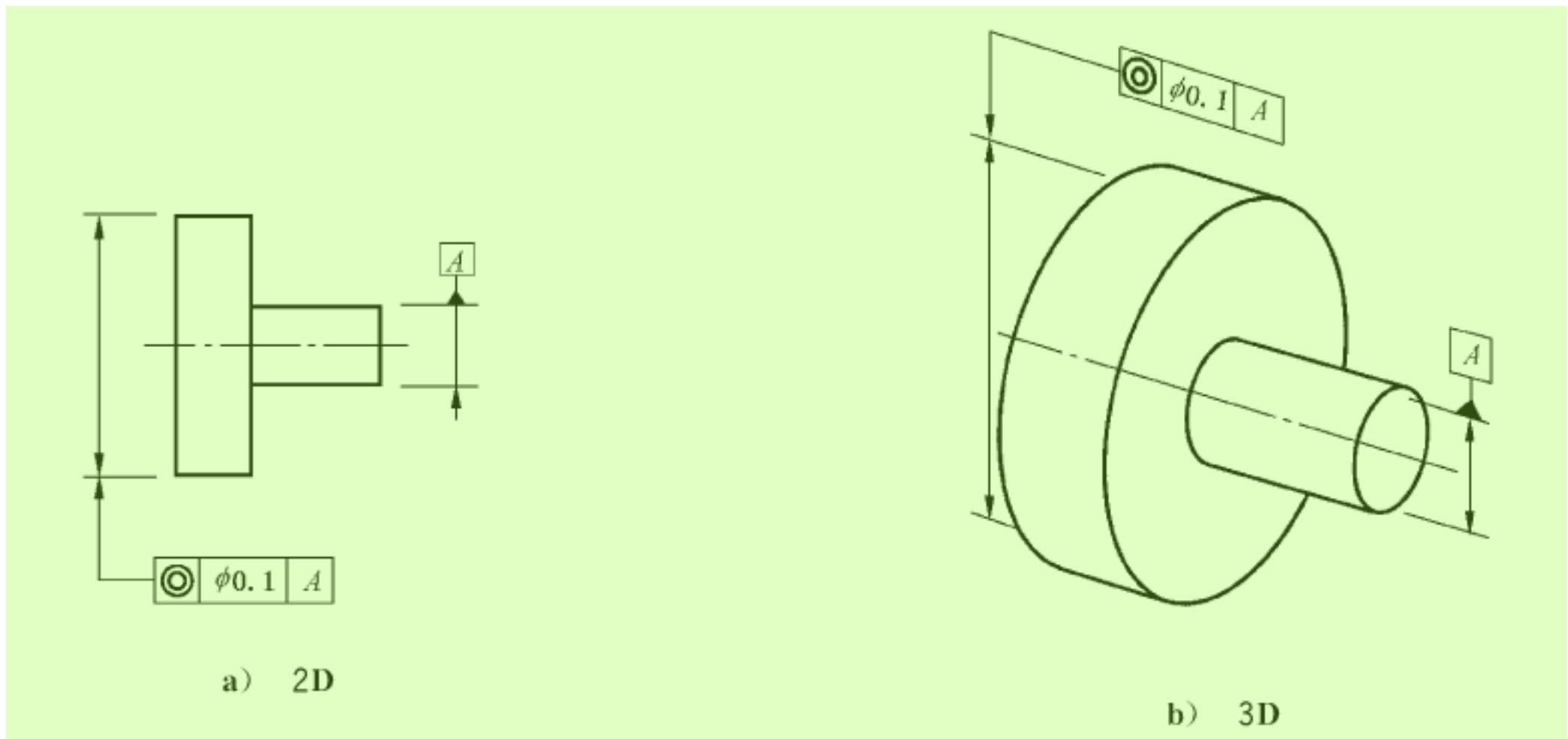
图 166 同轴度标注 3
