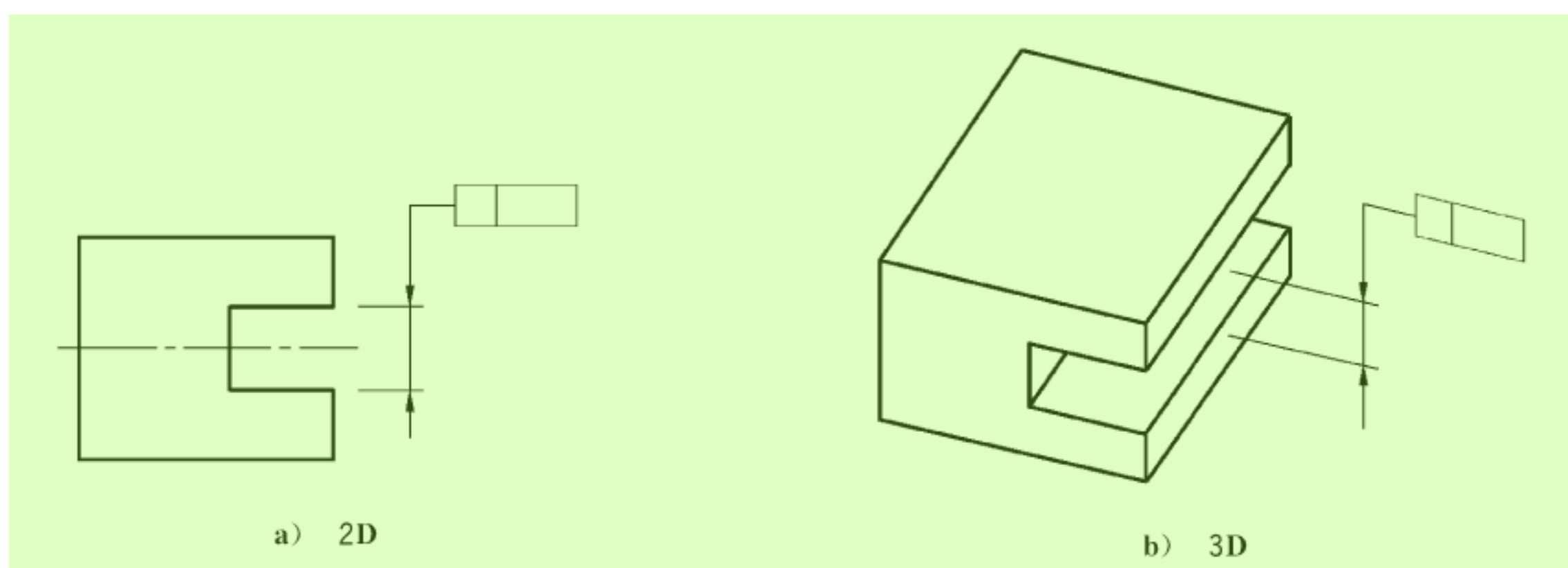
图 6 导出要素的标注
