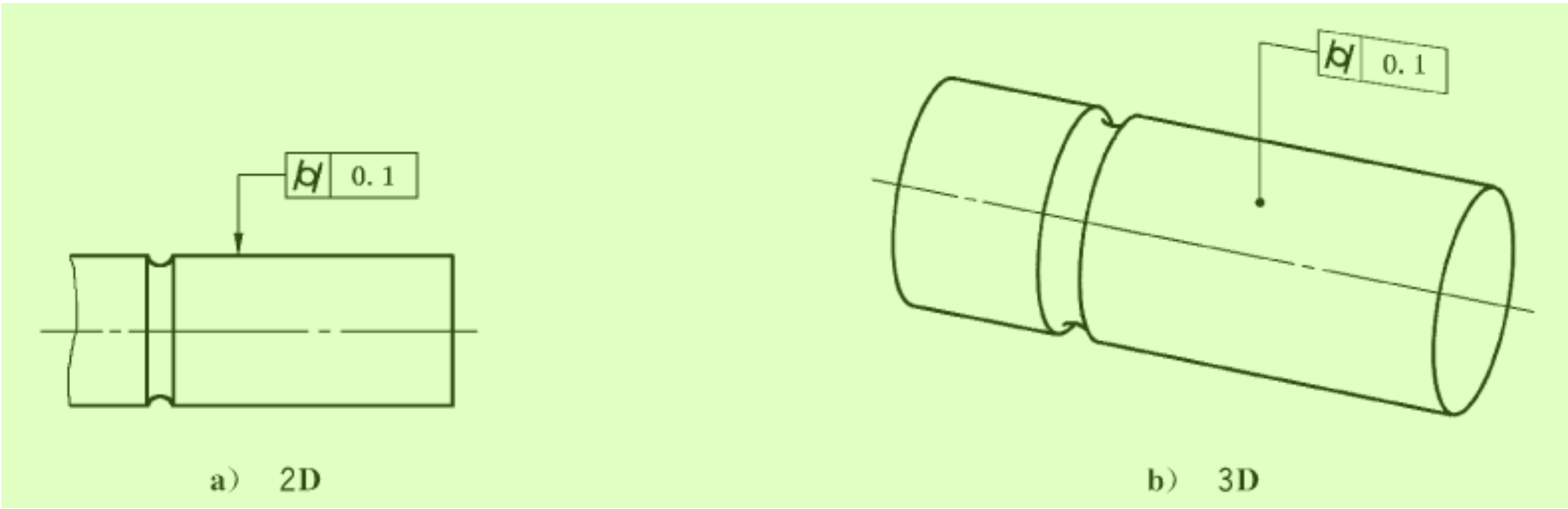
图 102 圆柱度标注
