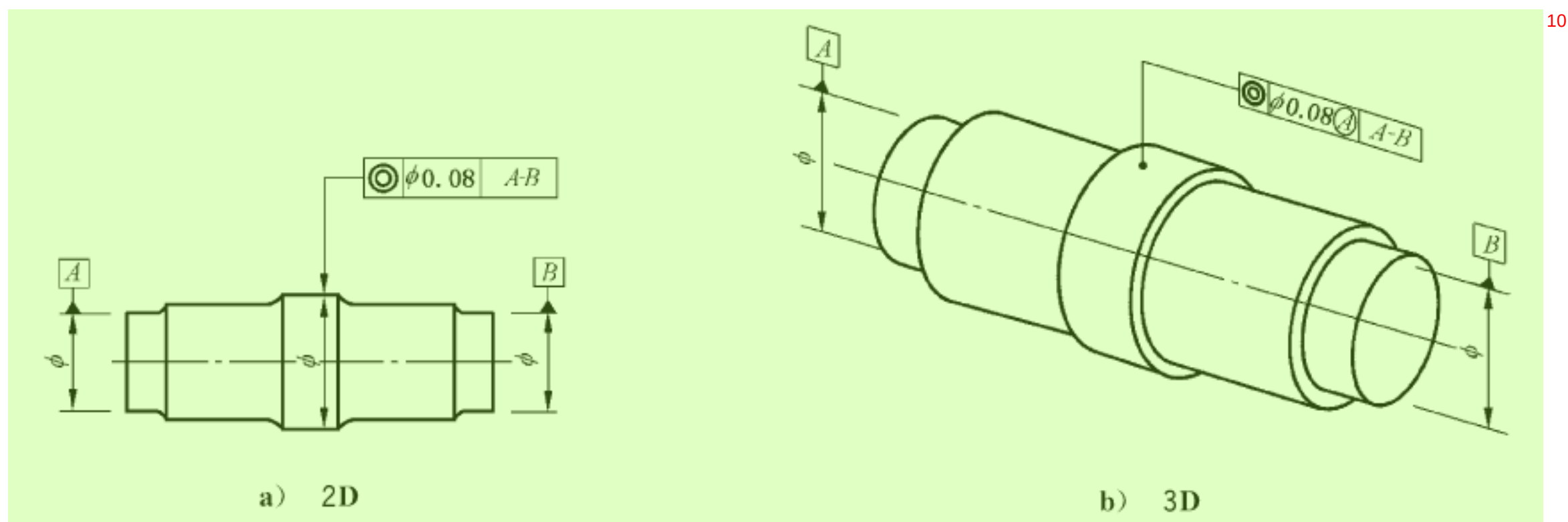
图 165 同轴度标注 11
