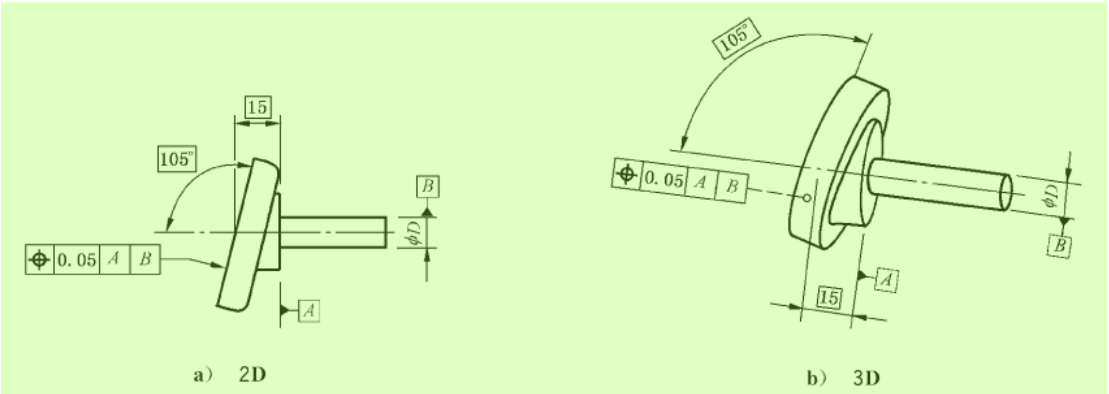
图 161 位置度标注 4
