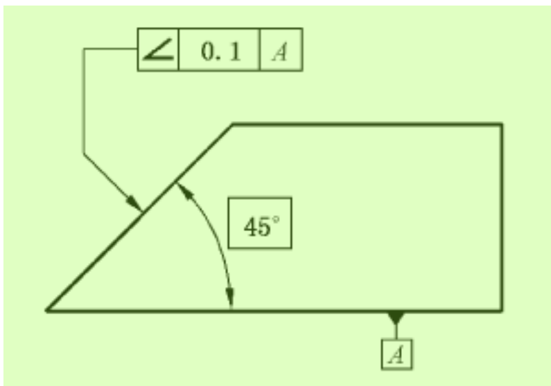
图 65 角度 TED 的标注
