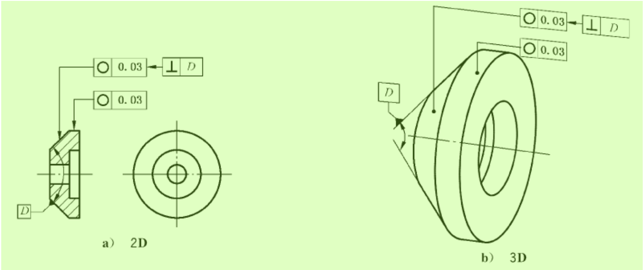
图 98 圆度标注 10
