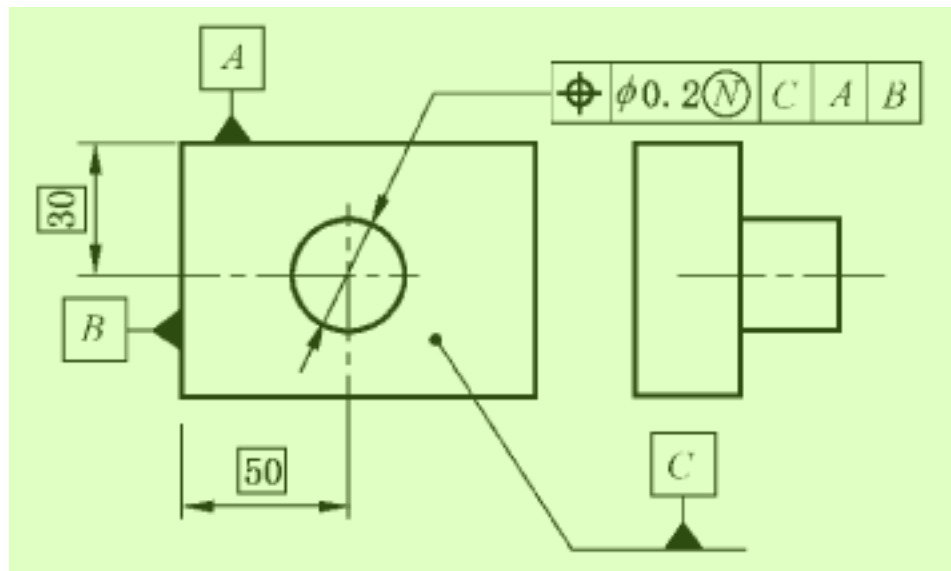
图 29 最小外接拟合被测要素——图样标注
