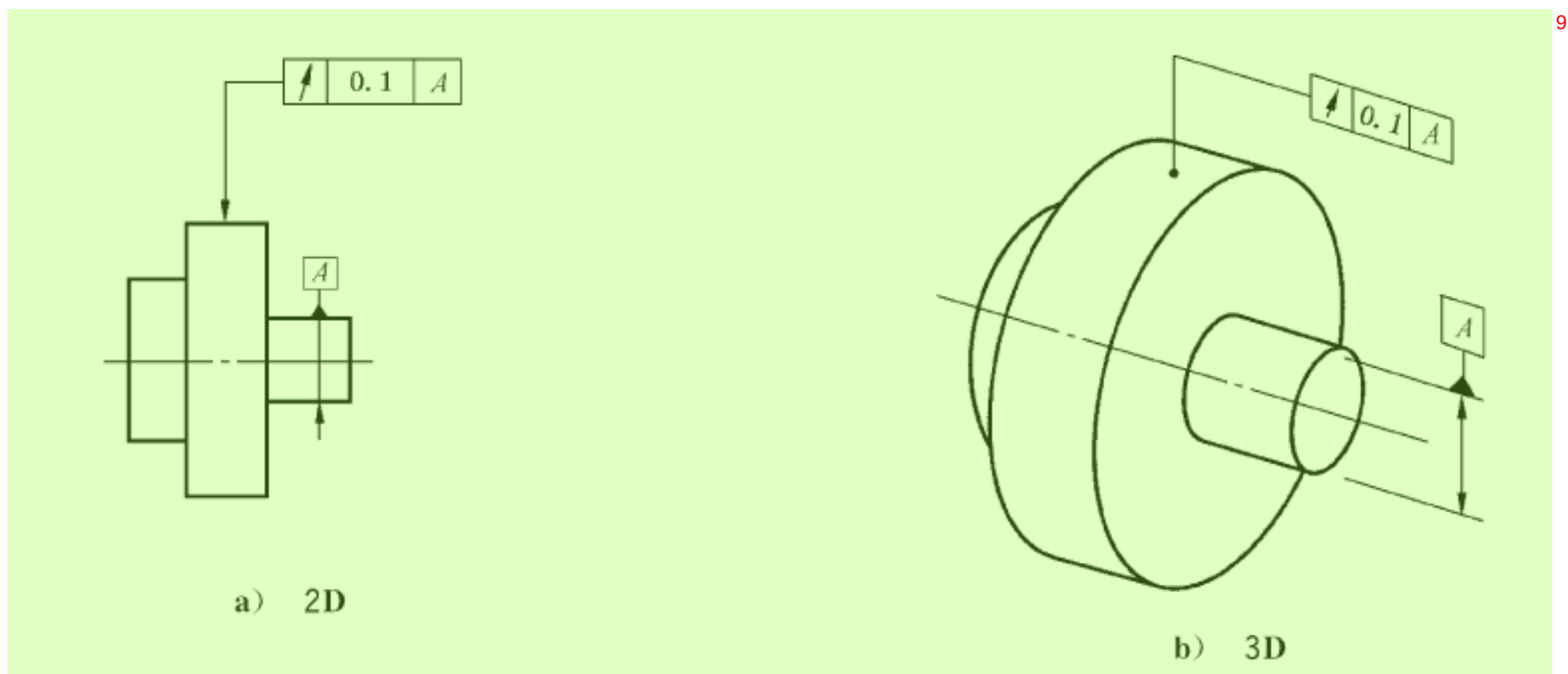
图 172 圆跳动标注
