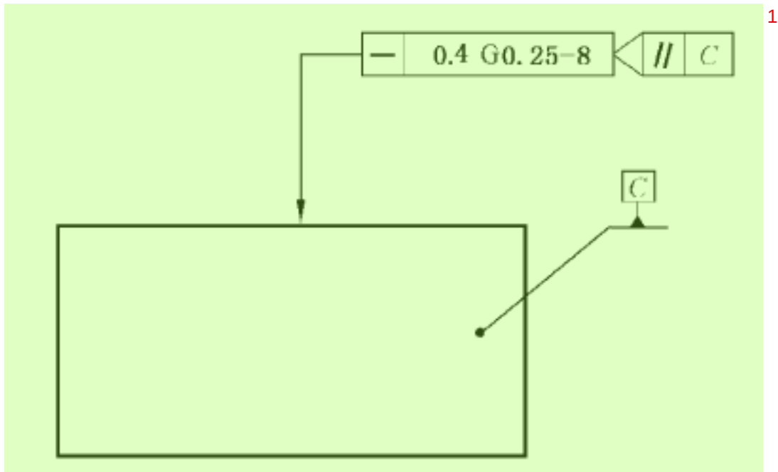
图 E.11 使用带通滤波器,用一种滤波器滤波后的直线度公差示例
