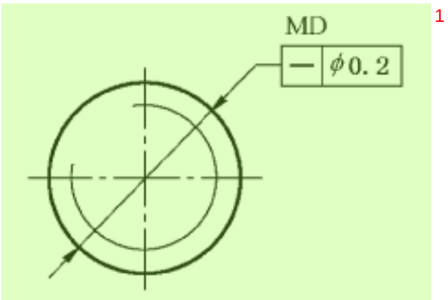
图 49 适用于螺纹大径的规范标注
