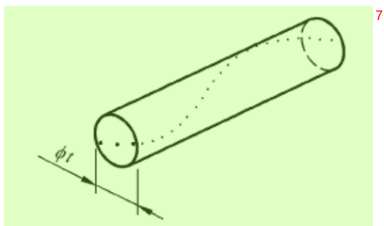
图 95 直线度公差带的定义
