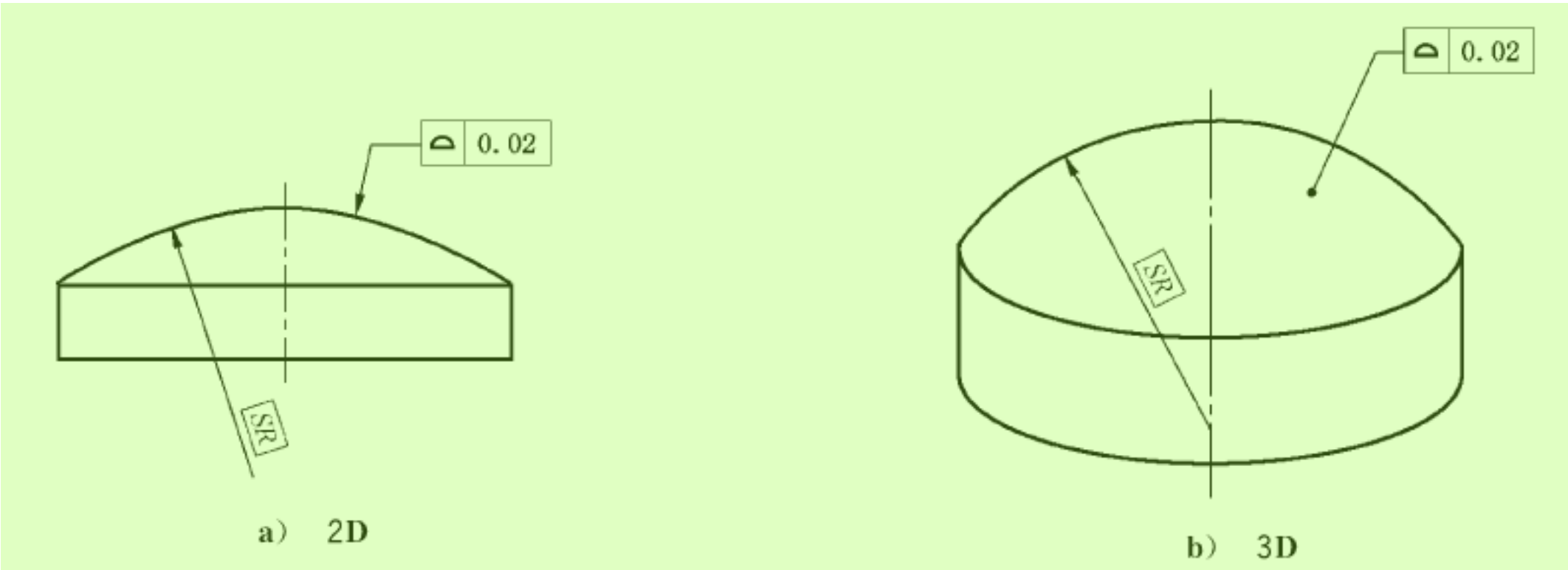
图 108 面轮廓度标注
