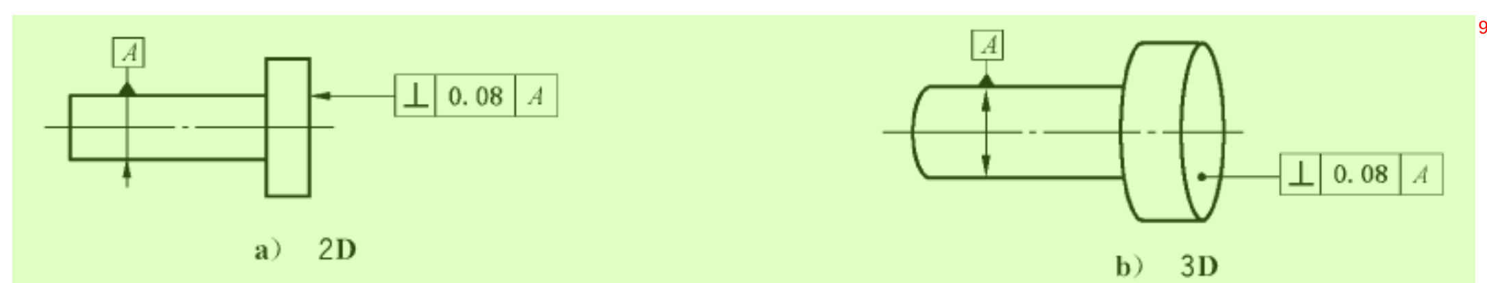
图 136 垂直度标注 10
