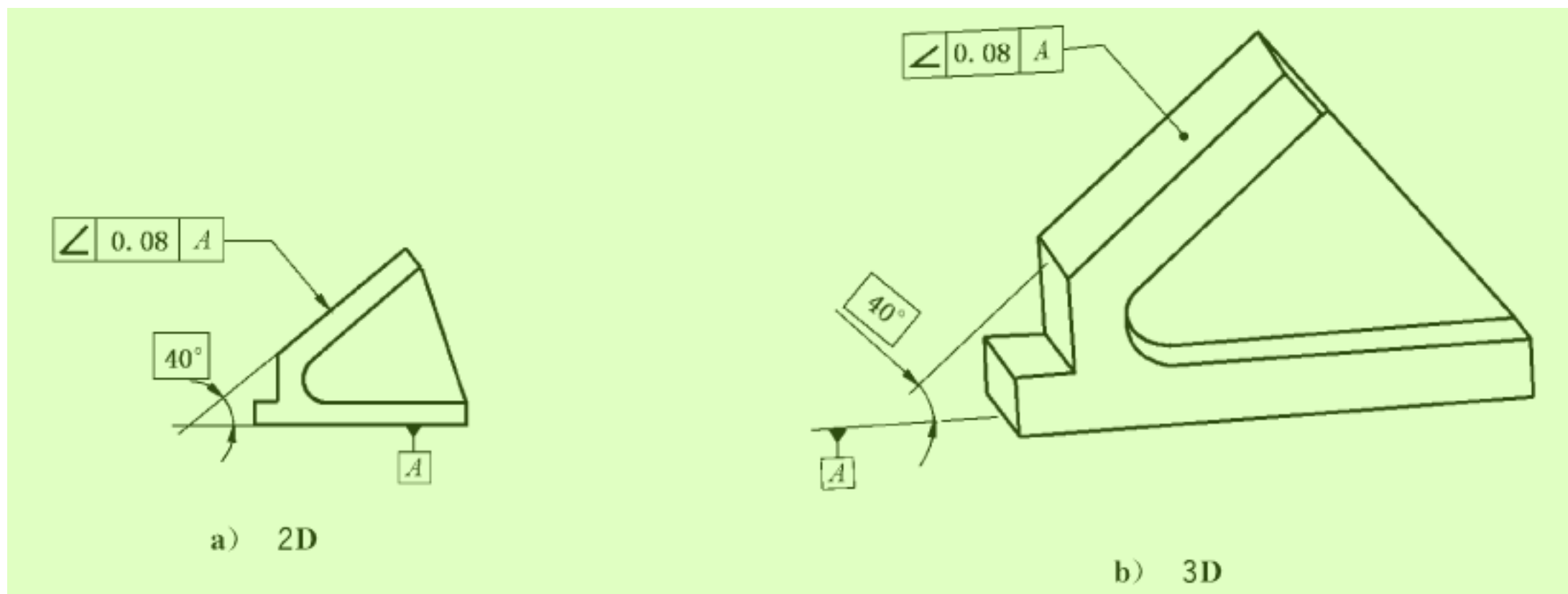
图 148 倾斜度标注 7
