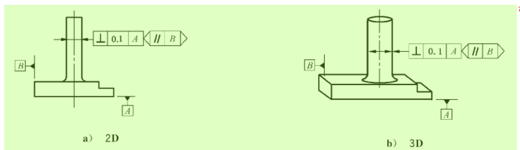
图 130 垂直度标注
