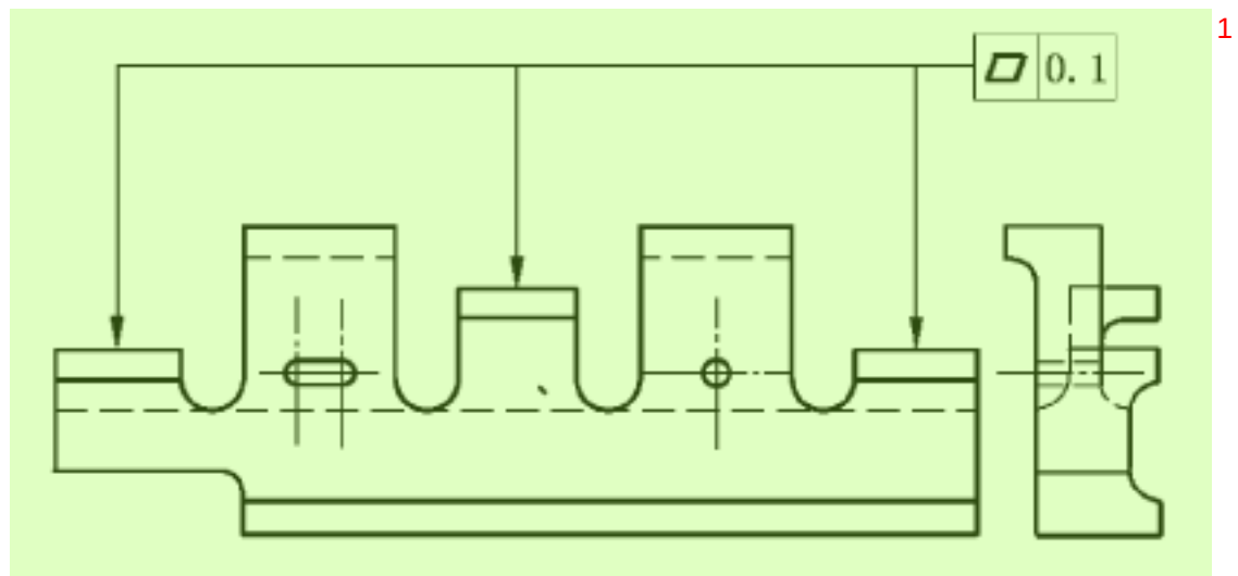
图 17 适用于多个单独要素的规范
