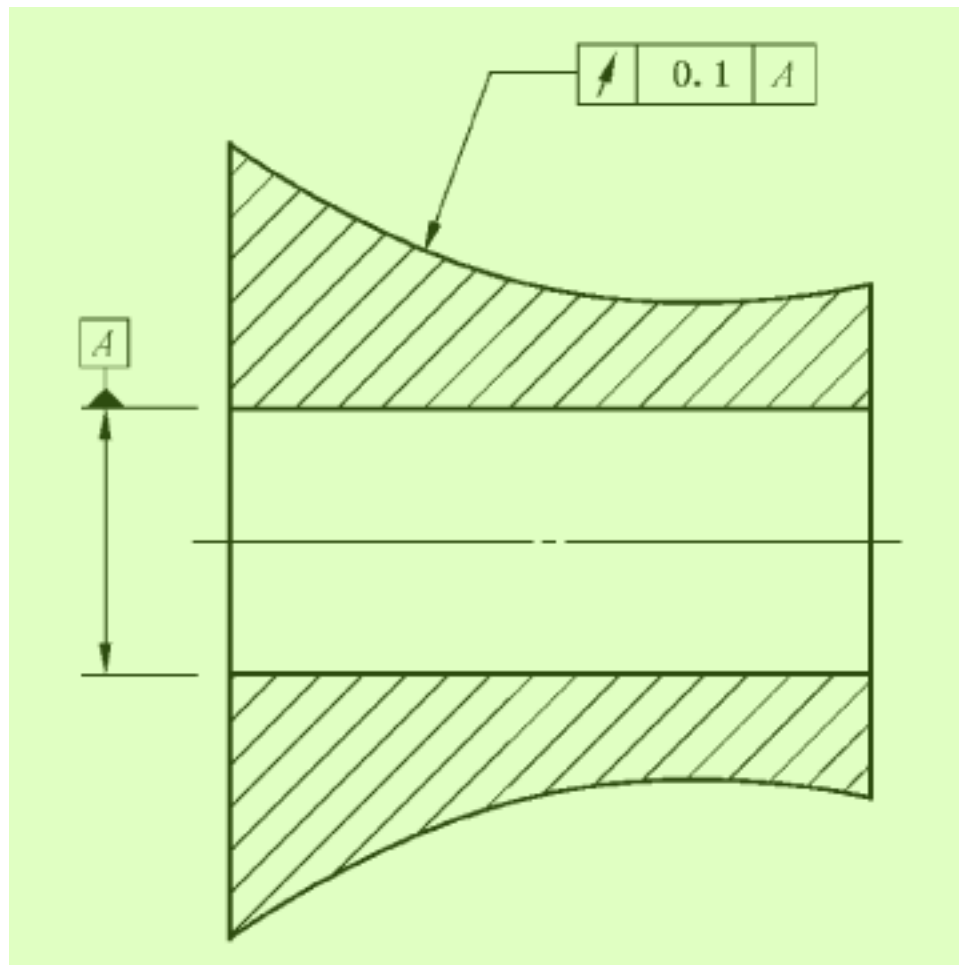
图 8 图样标注
