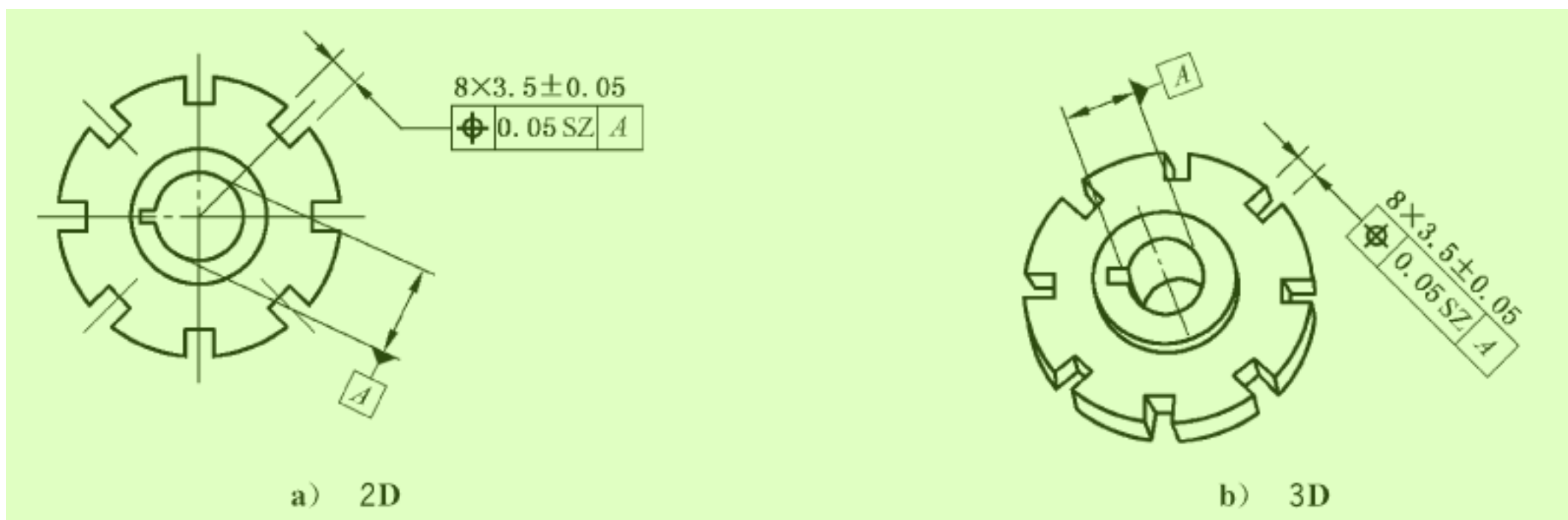
图 159 位置度标注
