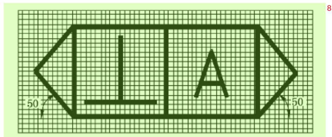
图 F.1 相交平面框格 6
