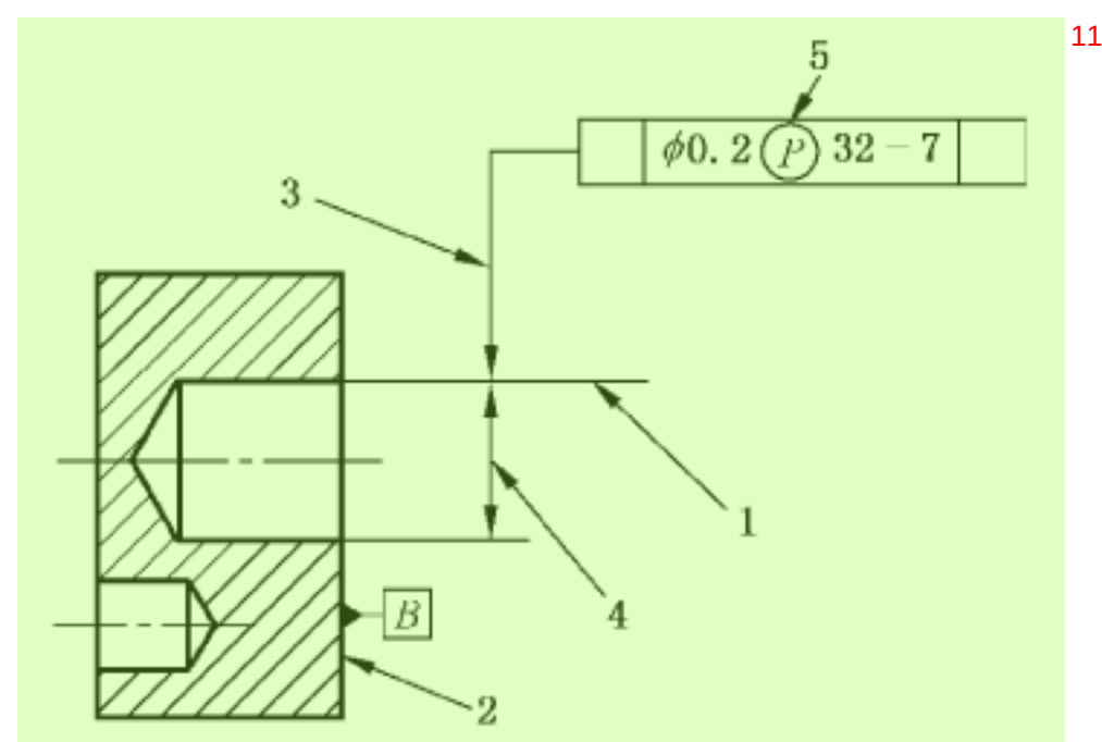
图 72 直接标注带偏置量的延伸公差带示例 8
