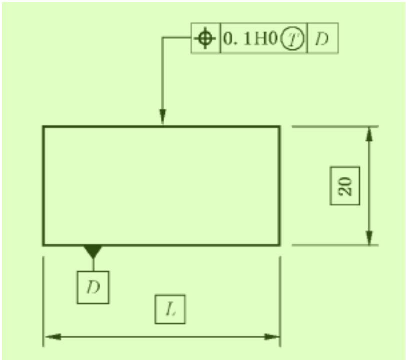
图 35 相对于凸包滤波要素拟合的贴切被测要素——图样标注
