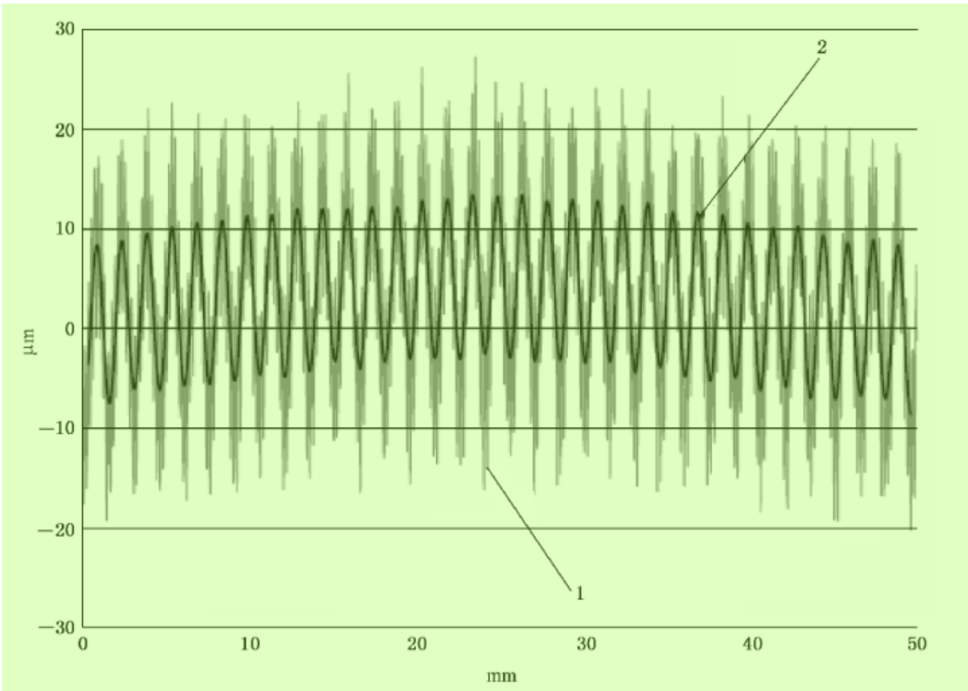
a) 0.8 mm 的长波通高斯滤波器
