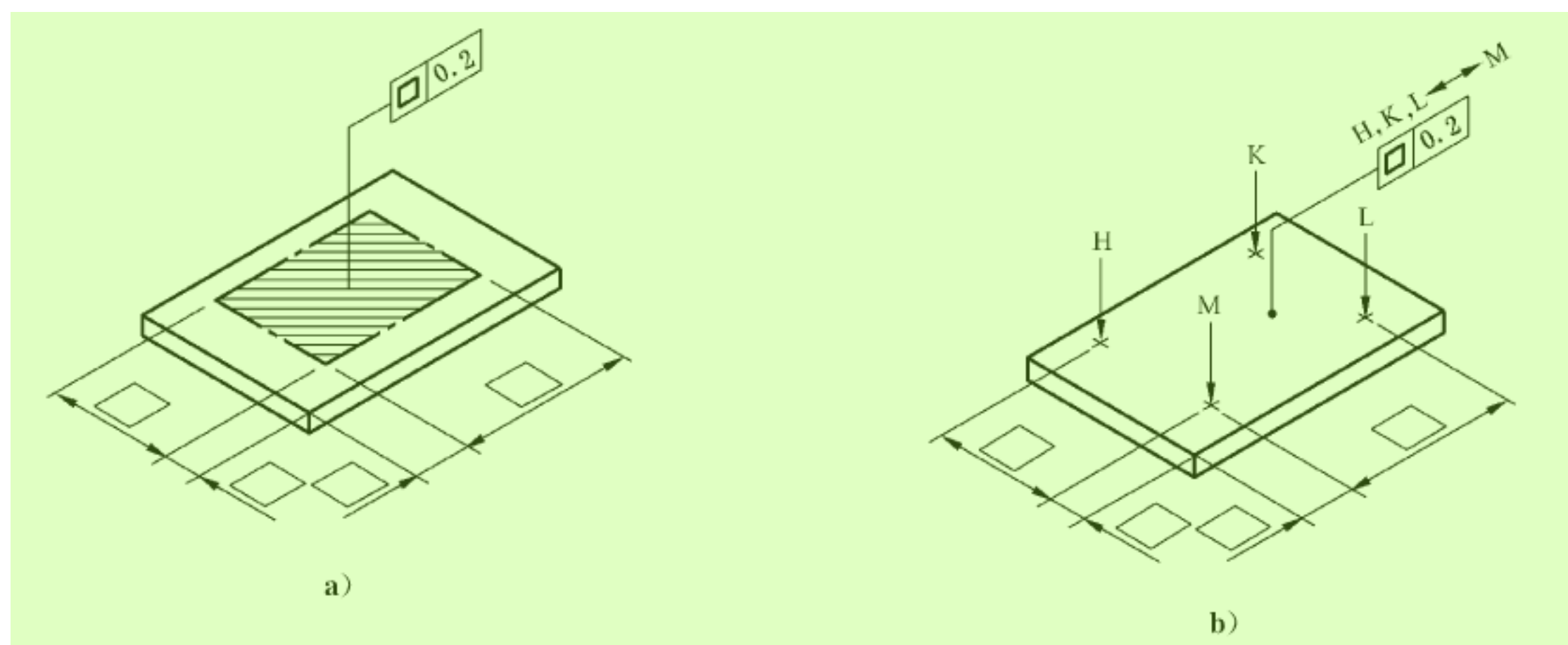
图 57 局部区域标注 5
