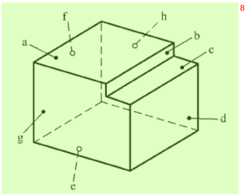
图 55 全表面图样标注
