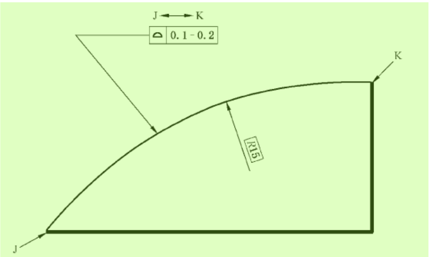
图 10 使用区间符号的变宽度公差带图样标注
