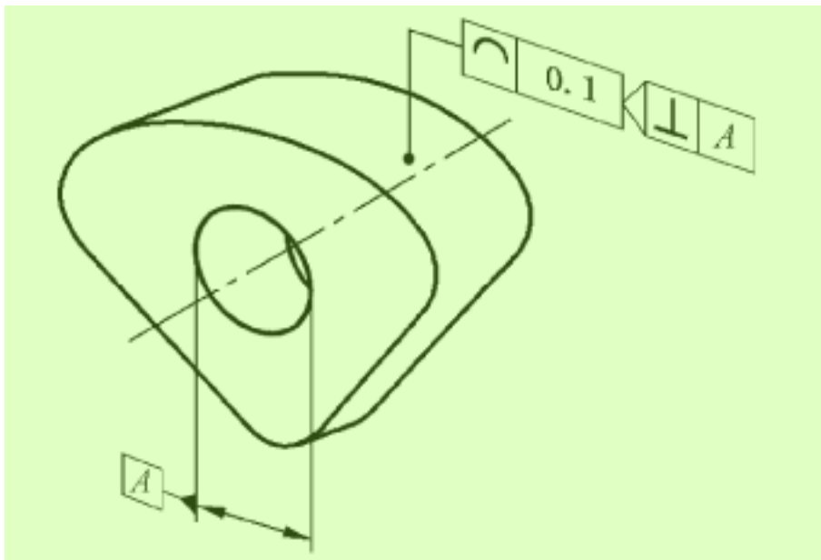
图 79 使用垂直于基准的相交平面规范 5
