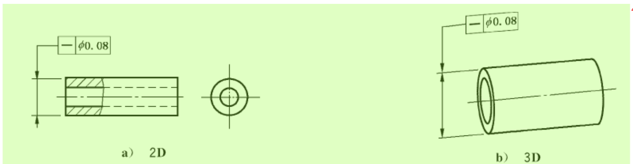
图 94 直线度标注
