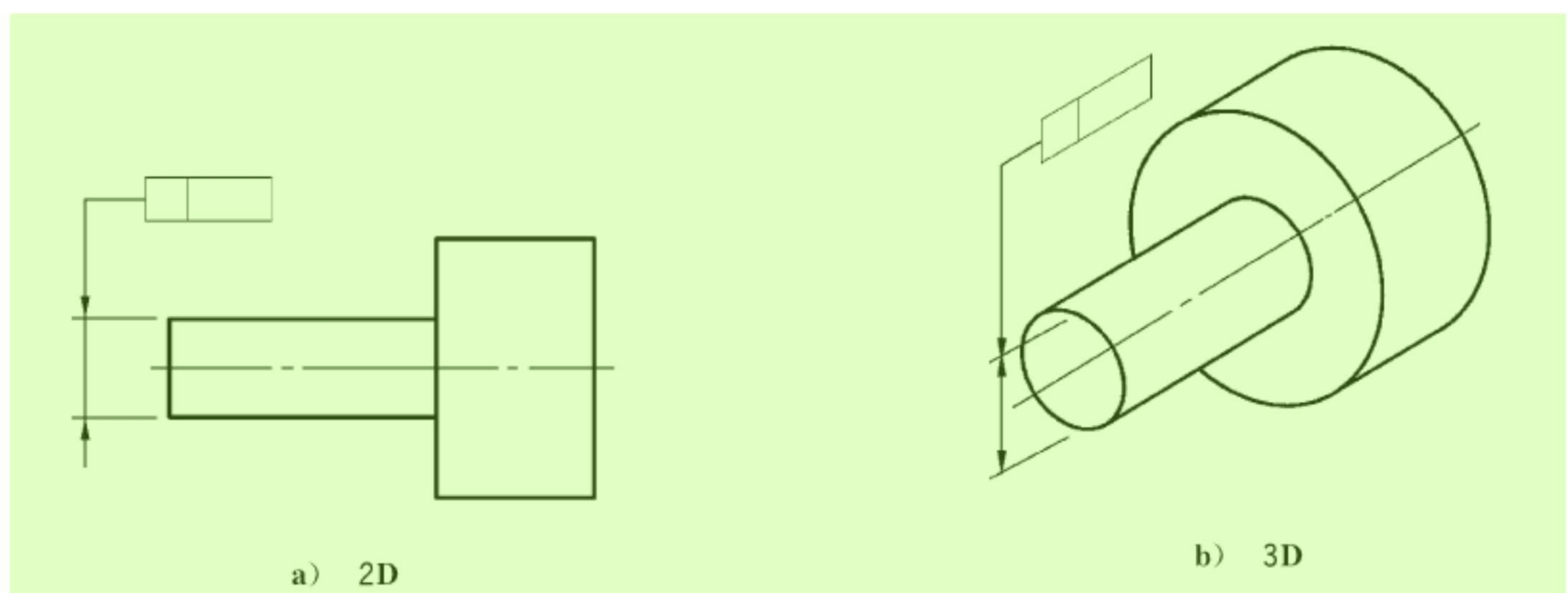
图 5 导出要素的标注
