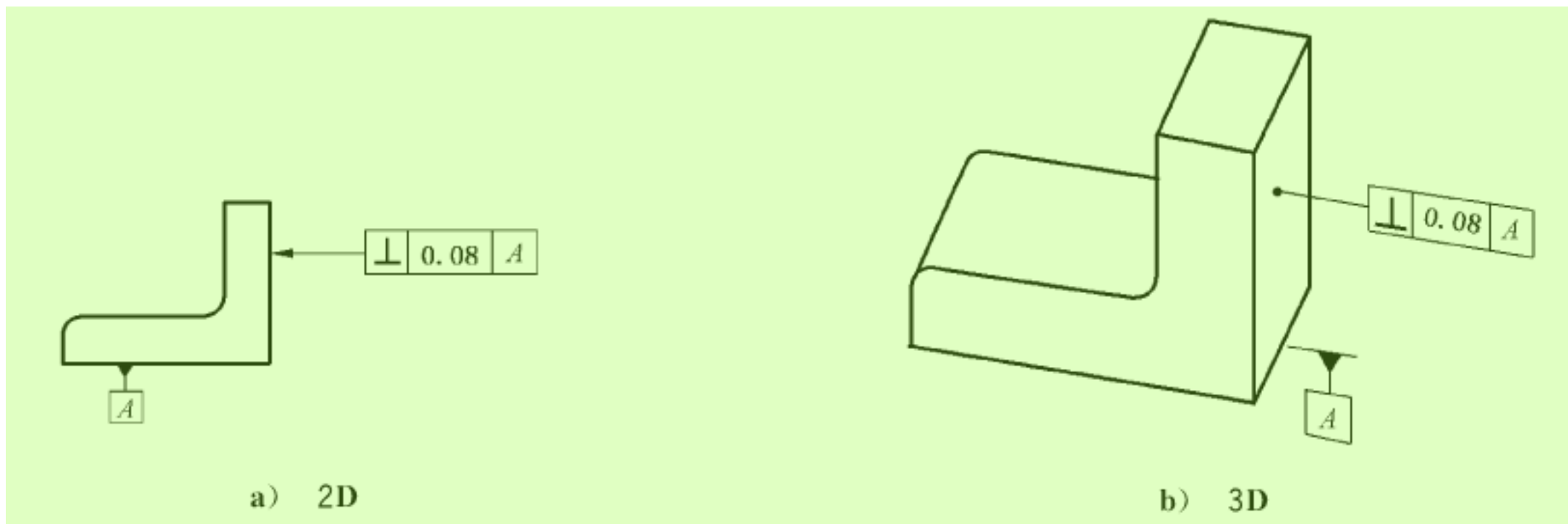
图 138 垂直度标注 8
