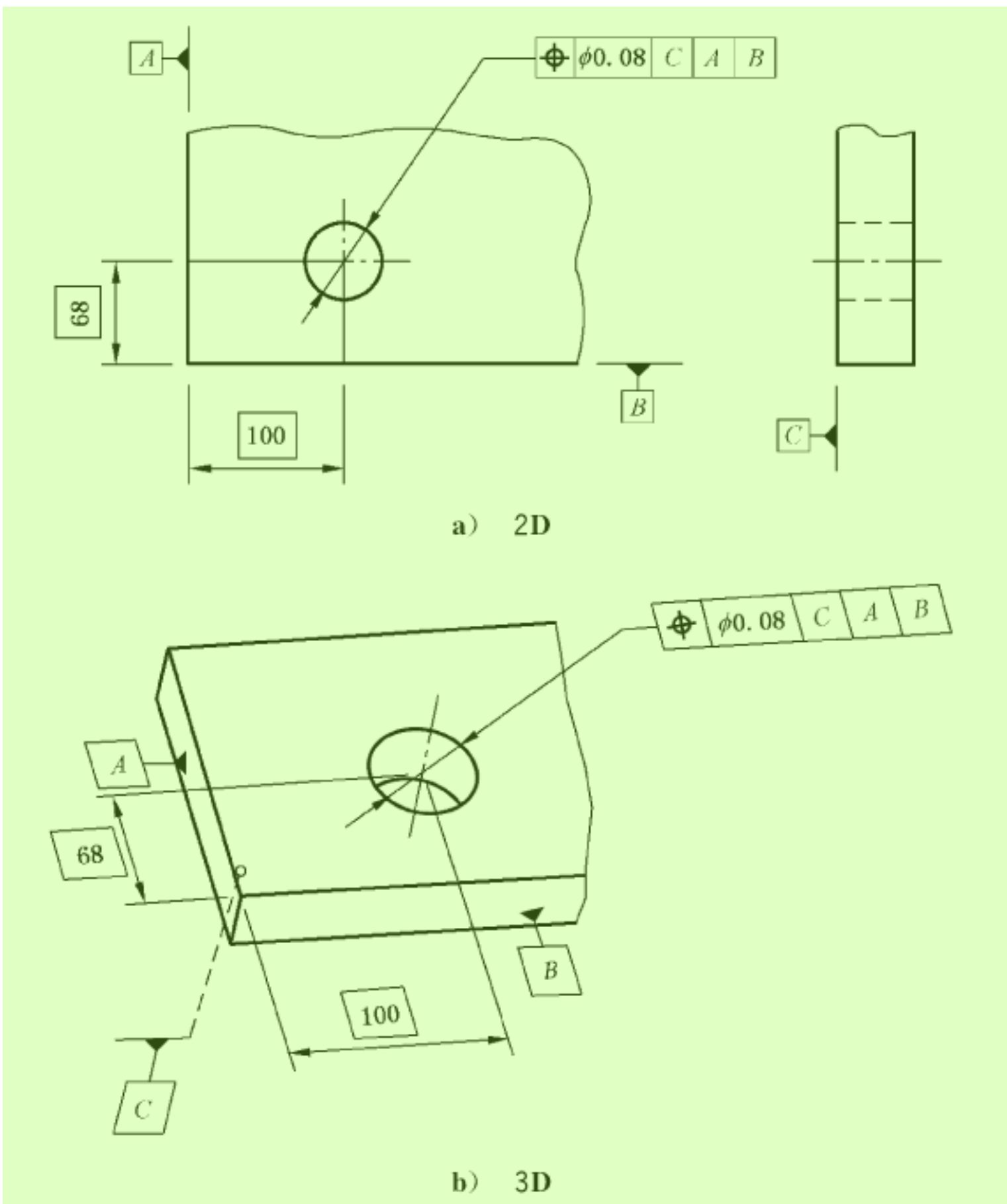
图 154 位置度标注 9
