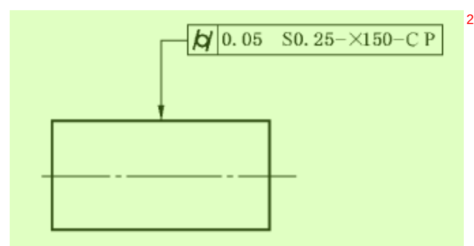
图 45 滤波规范,参照要素与特征规范元素 3
