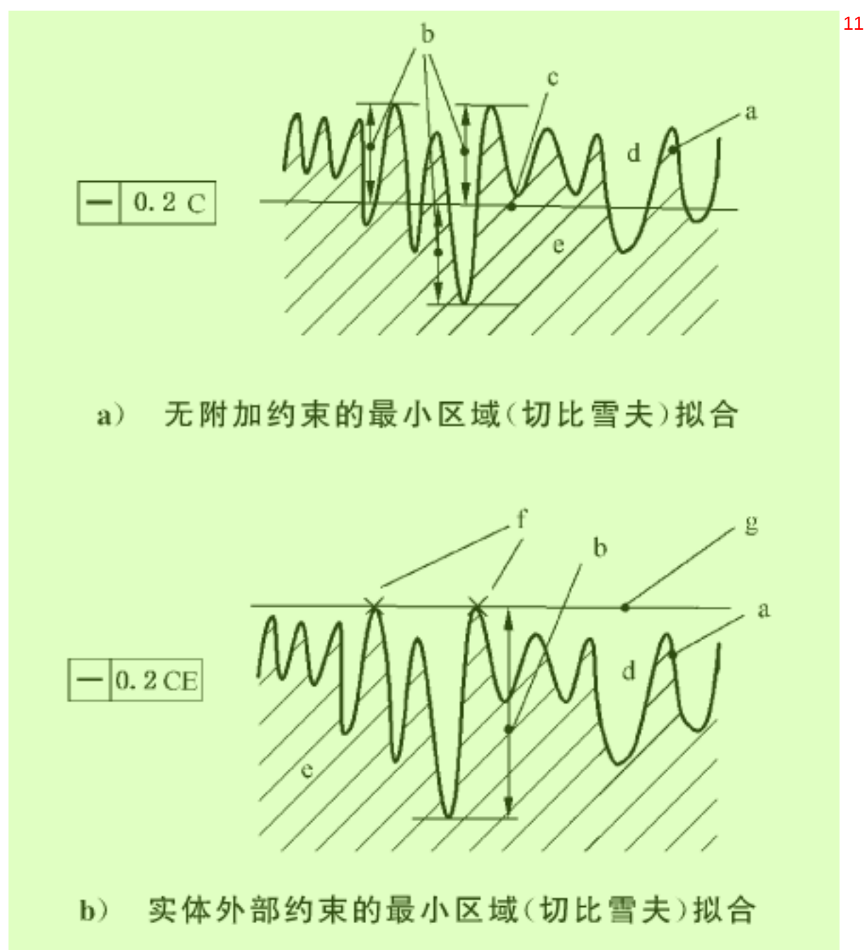
图 38 最小区域(切比雪夫)拟合 12
