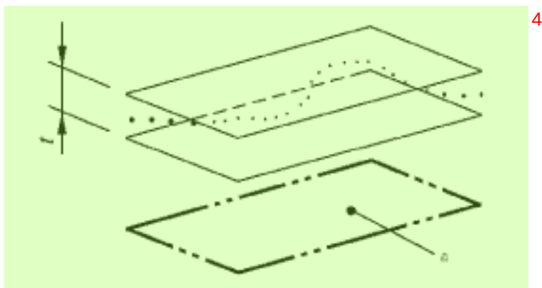
图 121 平行度公差带的定义 5
