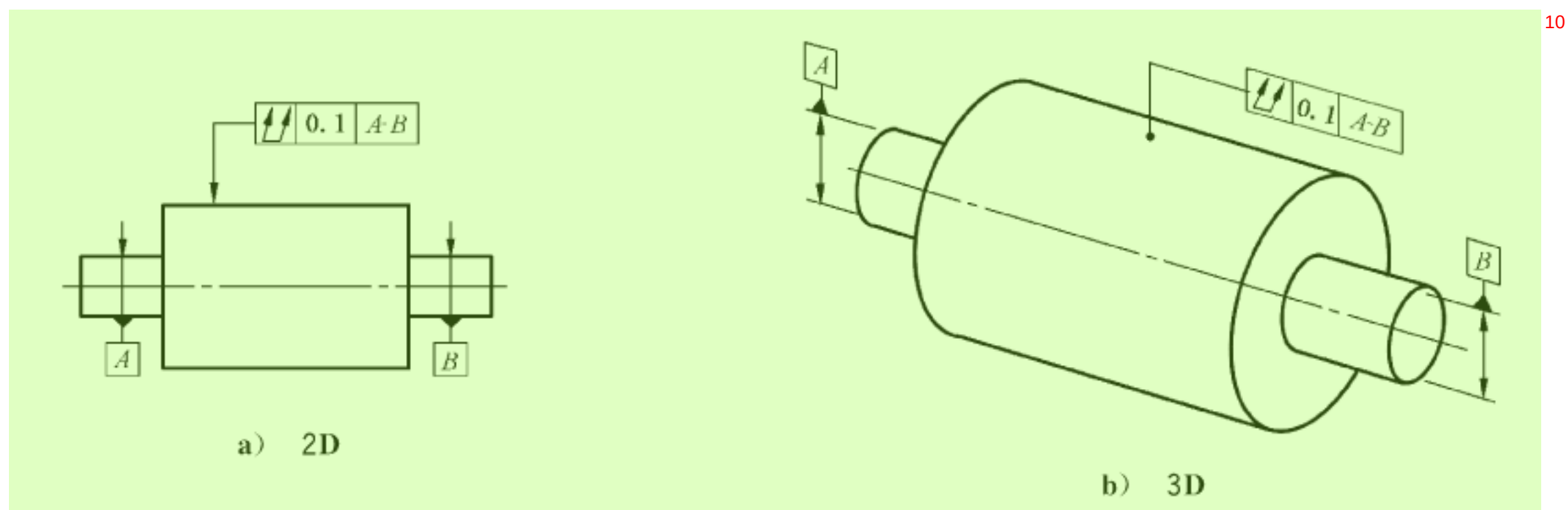
图 184 全跳动标注 11
