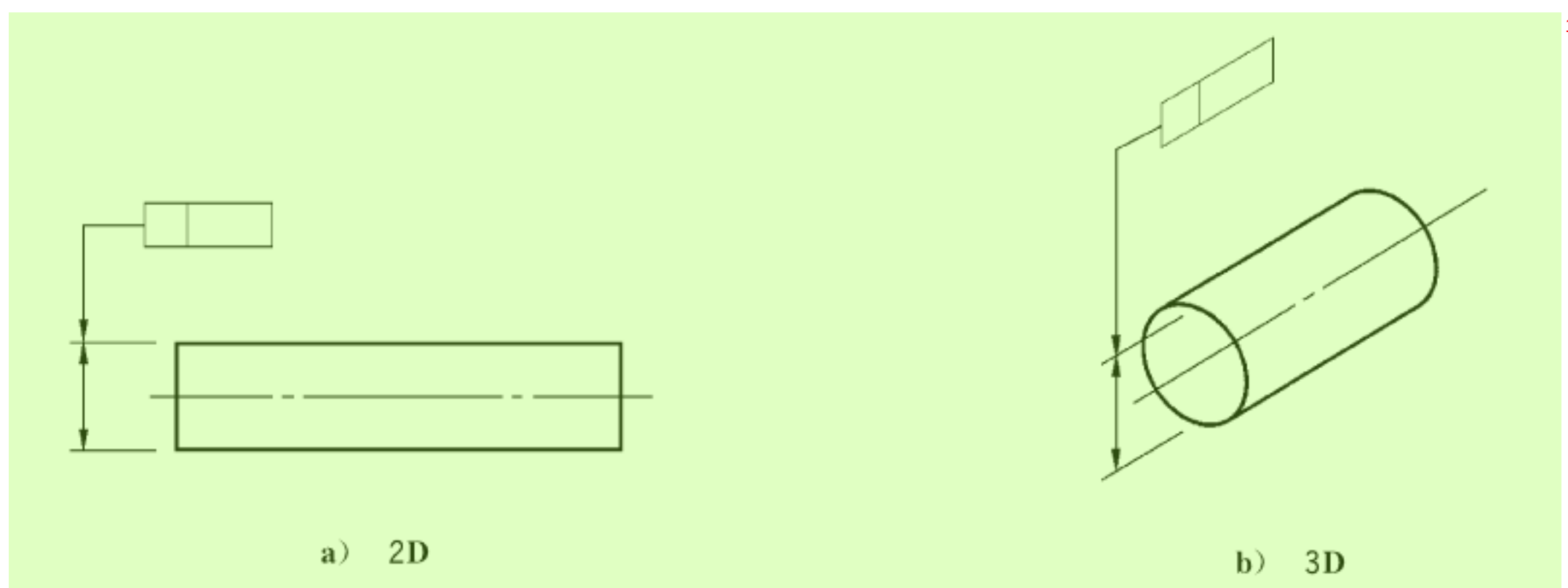
图 4 导出要素的标注
