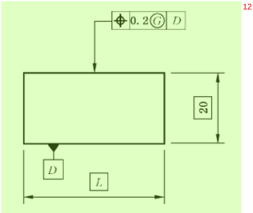
图 27 最小二乘(高斯)拟合被测要素——图样标注
