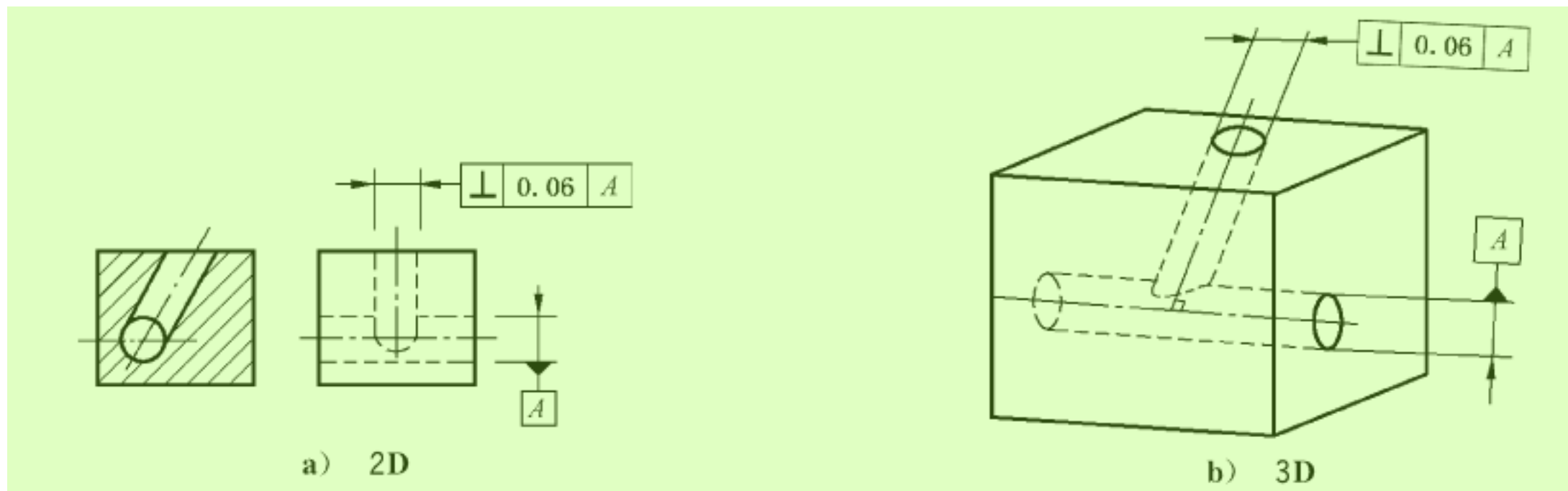
图 128 垂直度标注
