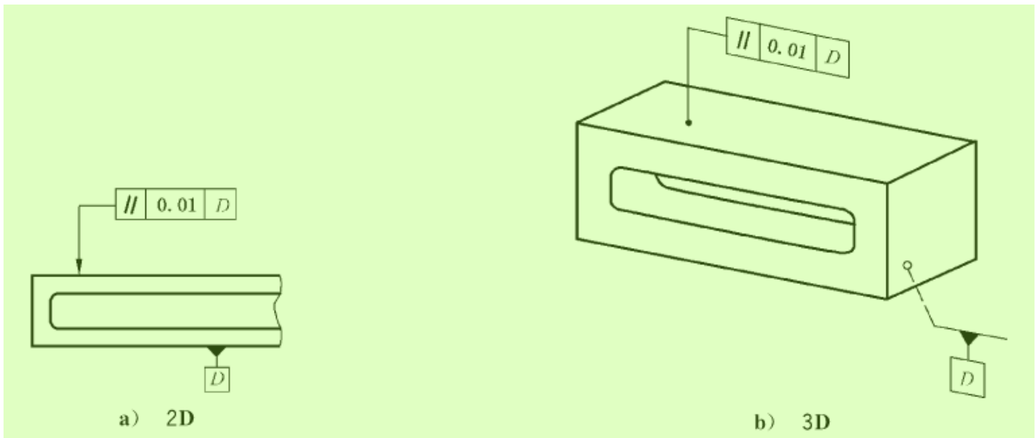
图 126 平行度标注
