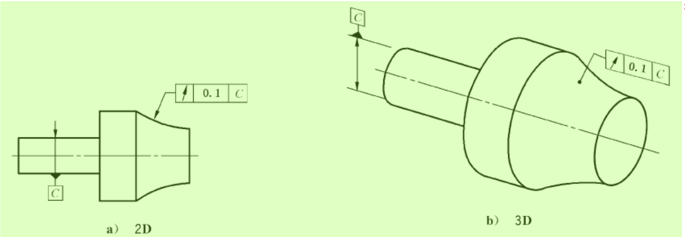
图 180 圆跳动标注 12
