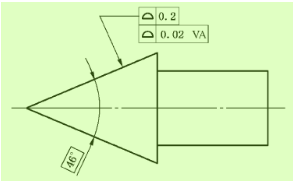
图 24 可变角度, VA, 修饰符 5
