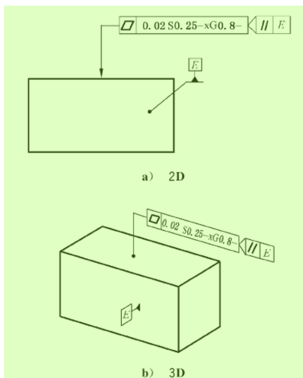
图 E.15 使用两种不同的长波通滤波器的平面度公差示例 2
