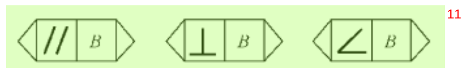
图 82 定向平面框格 12
