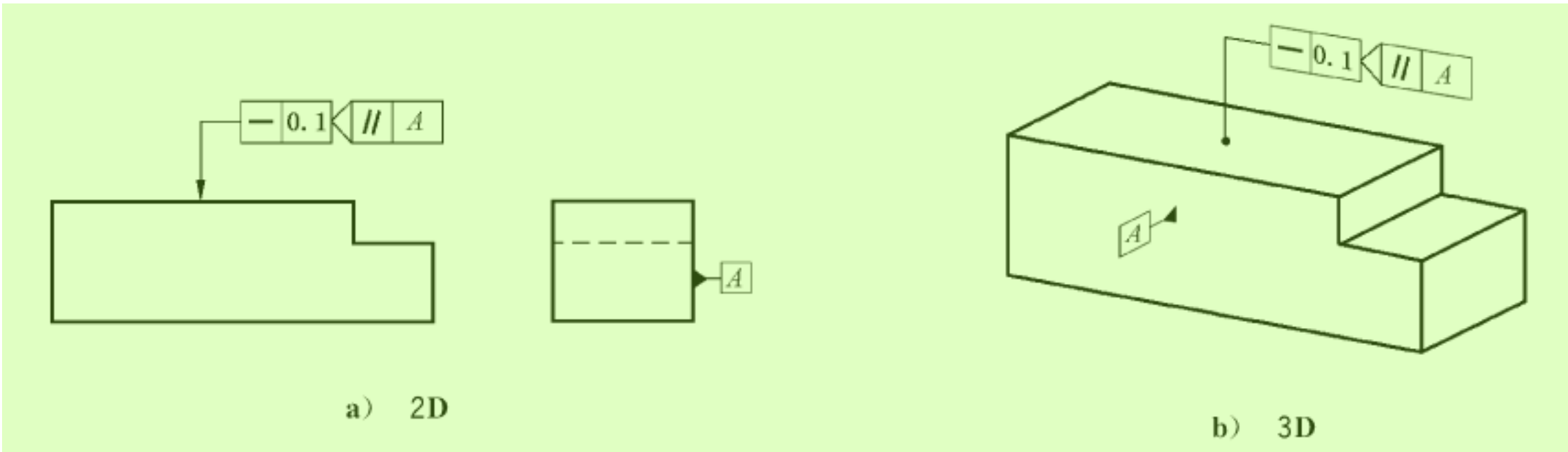
图 90 直线度标注 5
