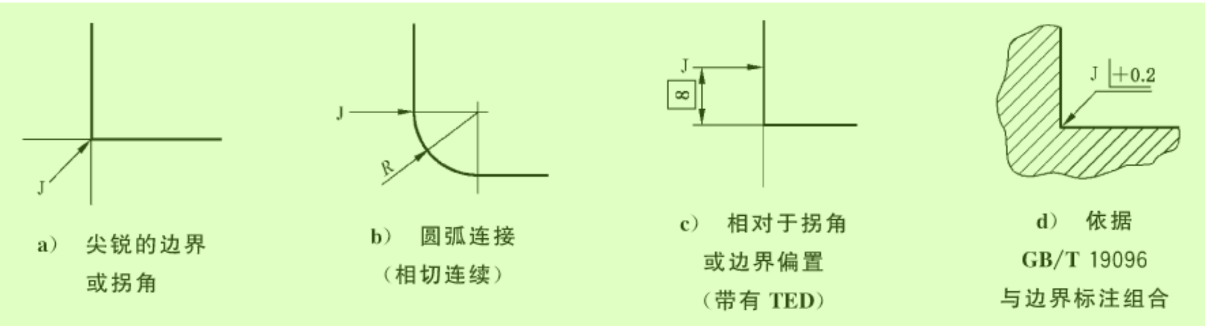
图 62 要素界限的标注
