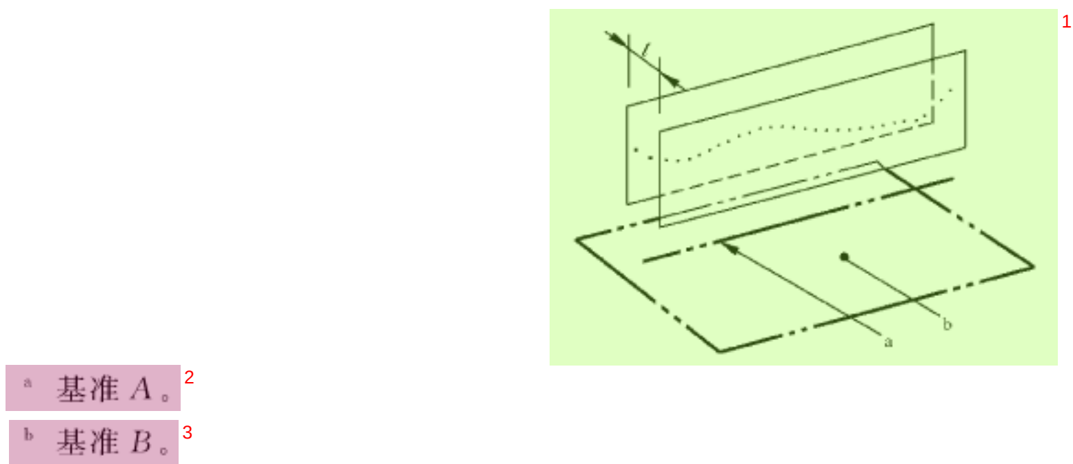
图 115 平行度公差带的定义
