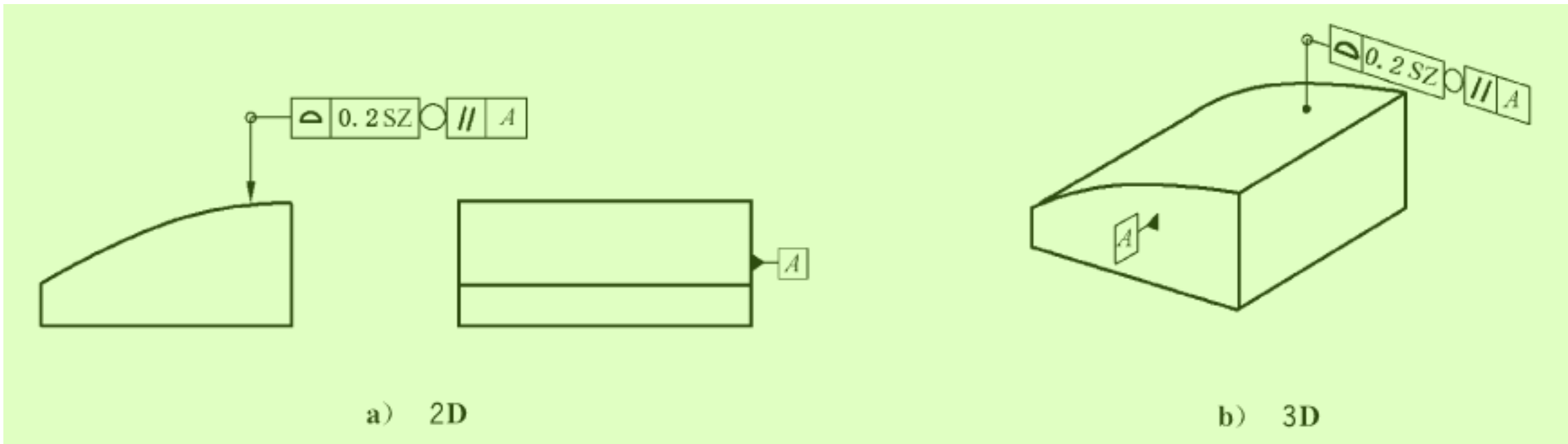
图 52 全周说明
