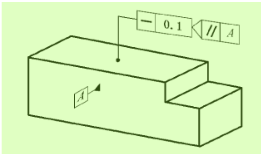
图 78 使用平行于基准的相交平面的规范 7
