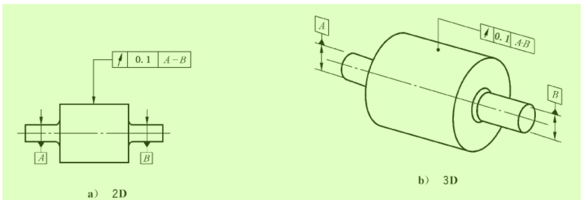
图 174 圆跳动标注 6
