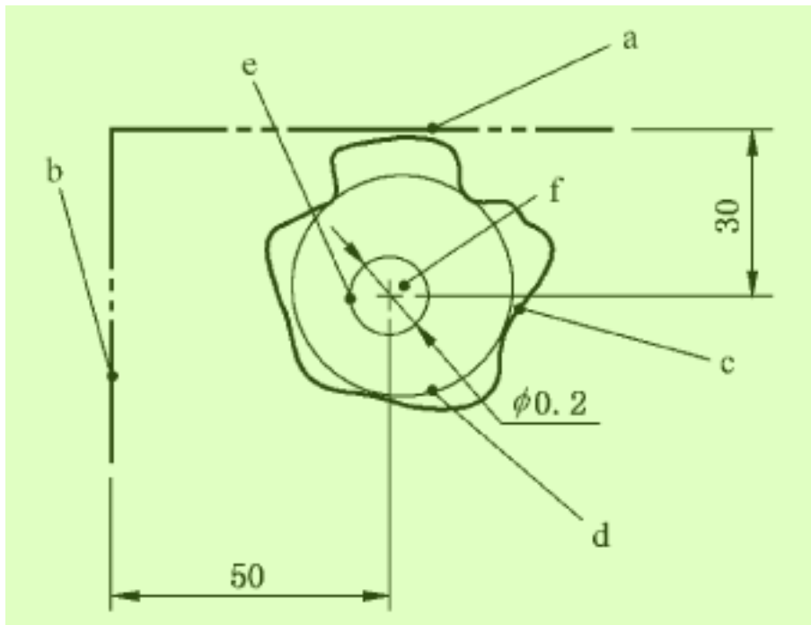
图 33 最大内切拟合被测要素——图样标注
