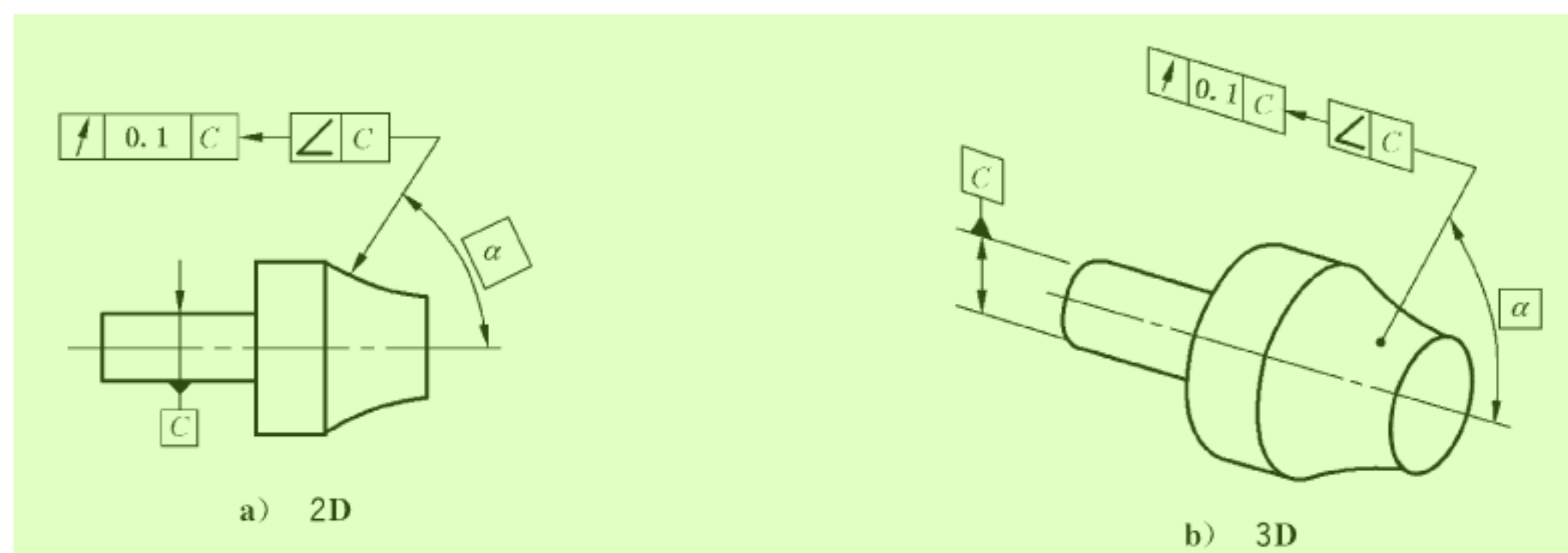
图 182 圆跳动标注 10
