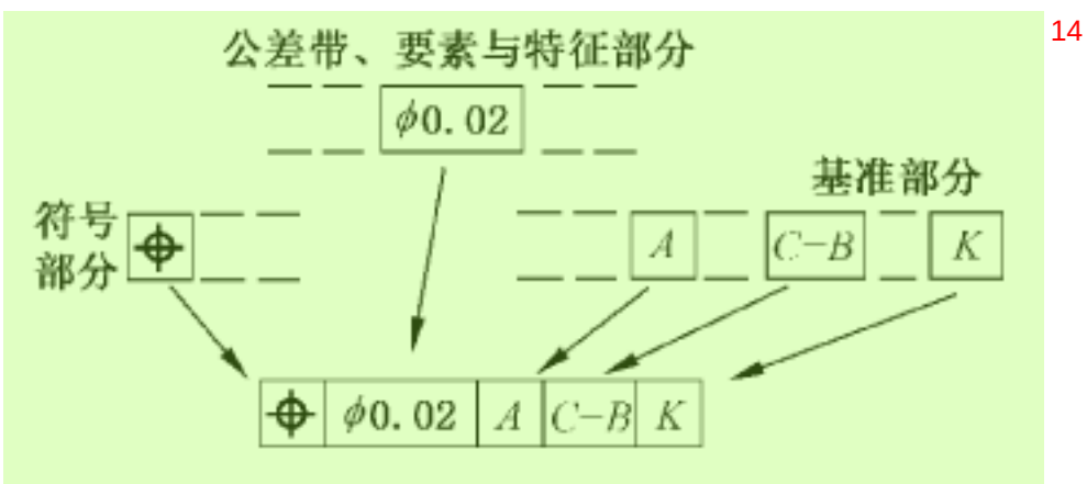
图 12 公差框格的三个部分 15
