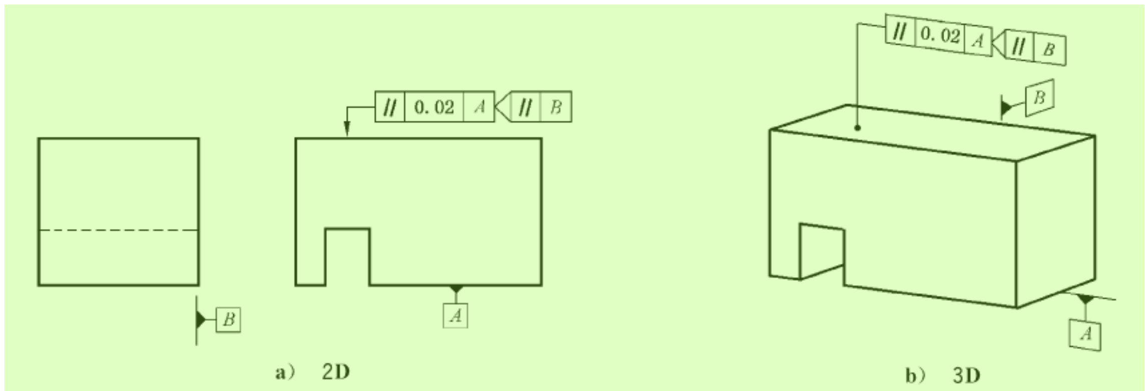
图 122 平行度标注 10
