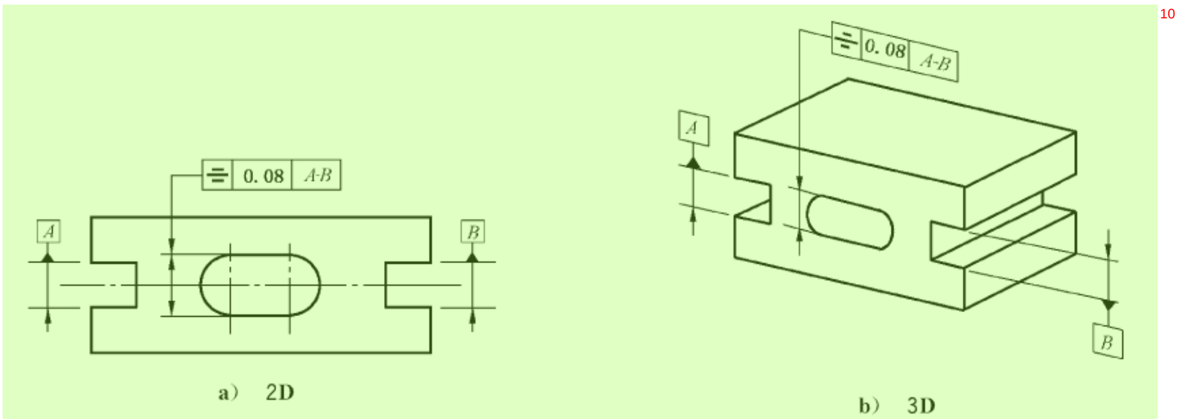
图 170 对称度标注 11
