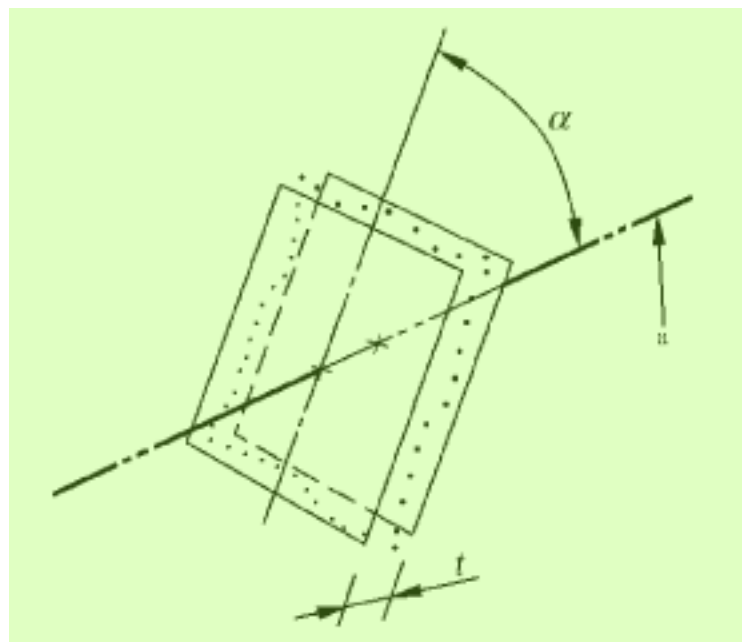
图 147 倾斜度公差带的定义 2
