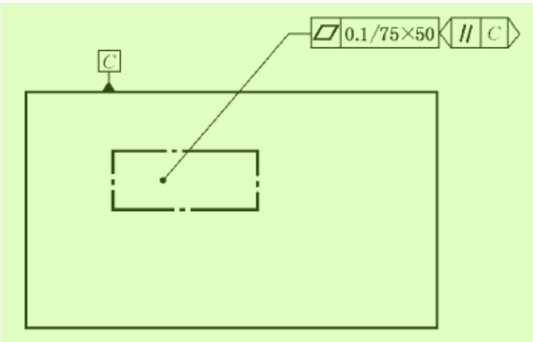
图 67 区域局部规范的标注 6
