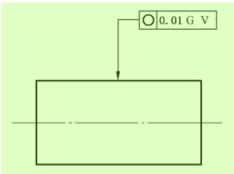
图 44 使用最小二乘(高斯)参照要素规范与谷深特征规范的规范 25
