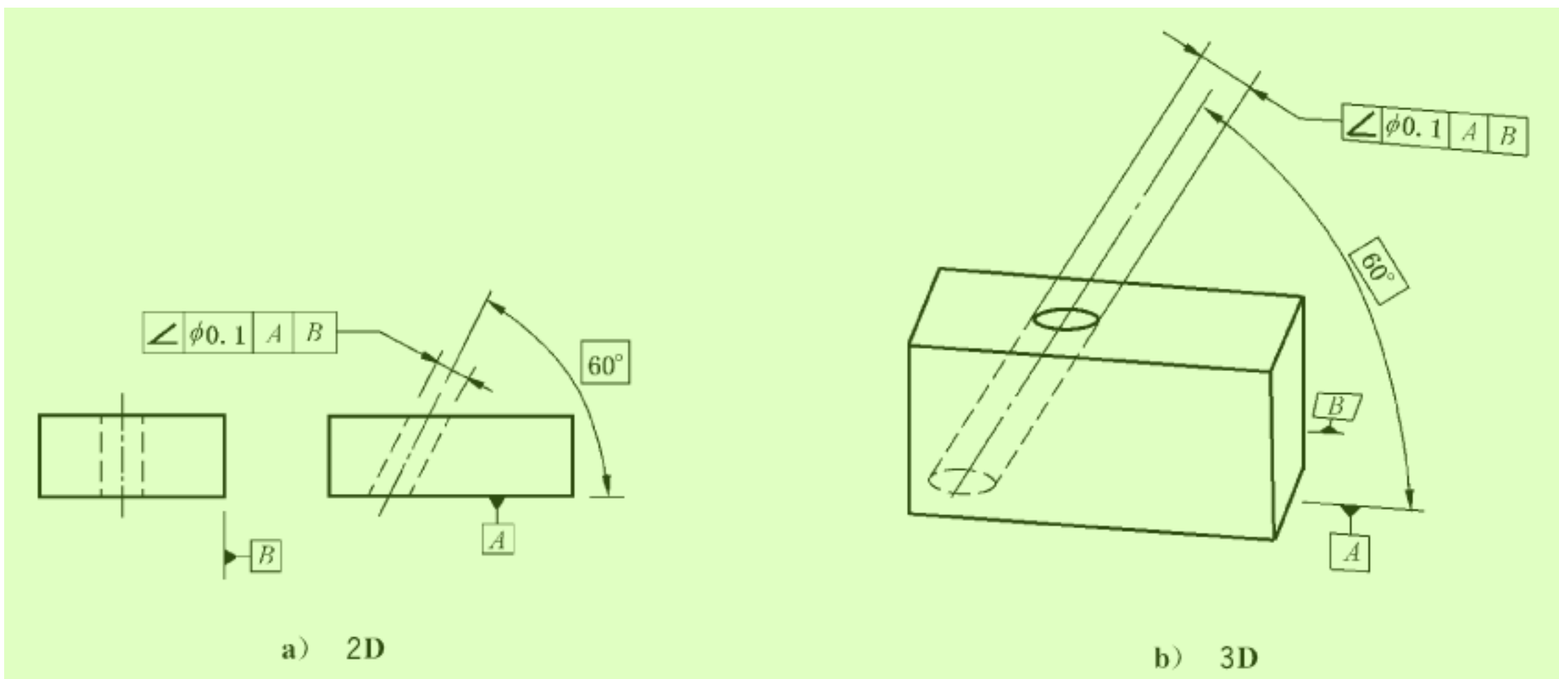
图 144 倾斜度标注
