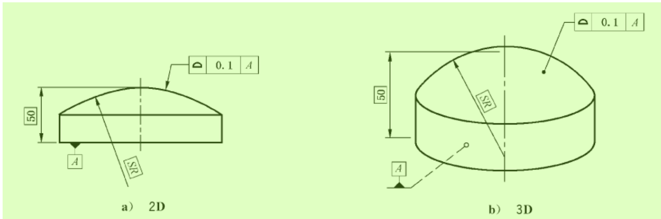
图 110 面轮廓度标注
