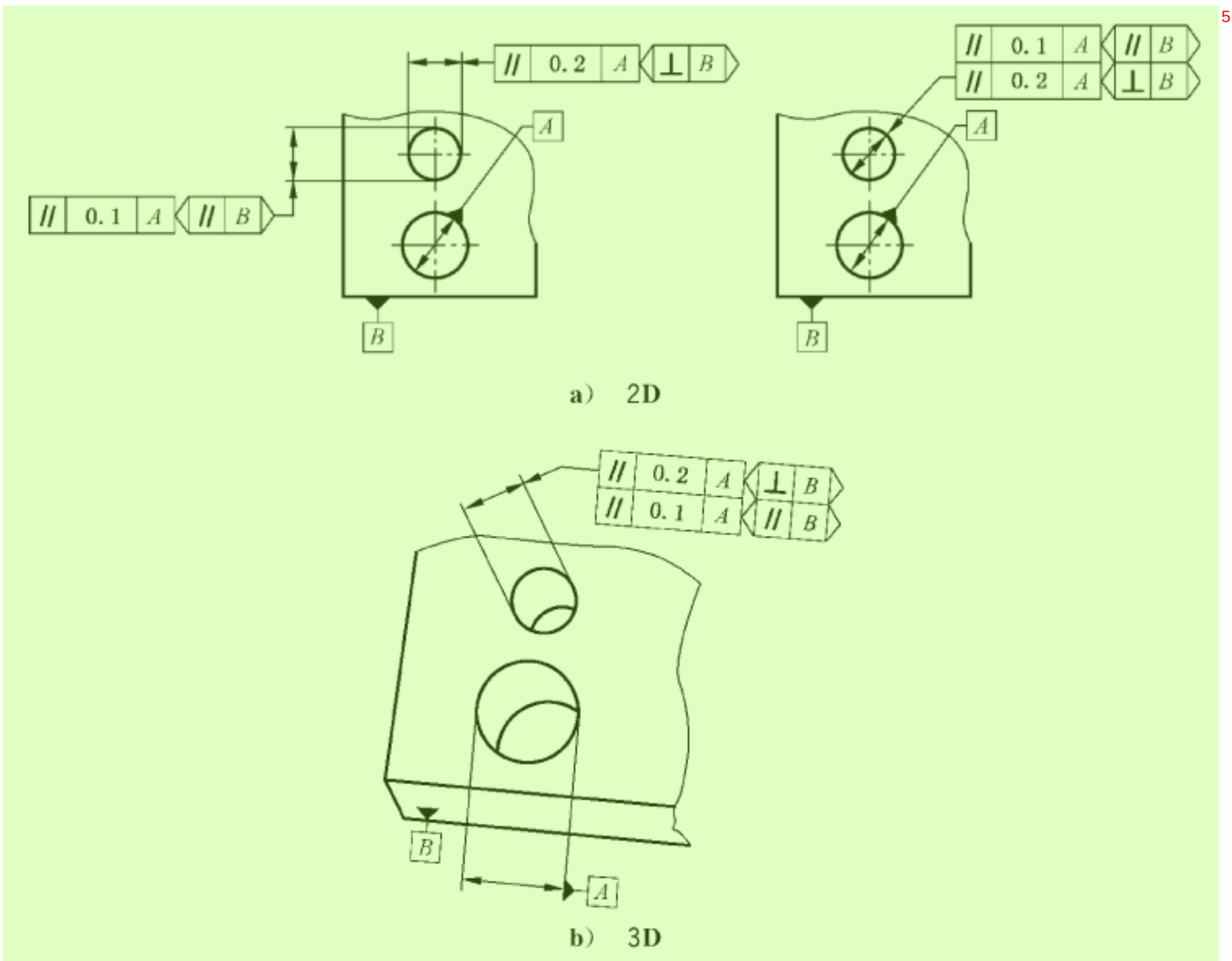
图 116 平行度标注 6
