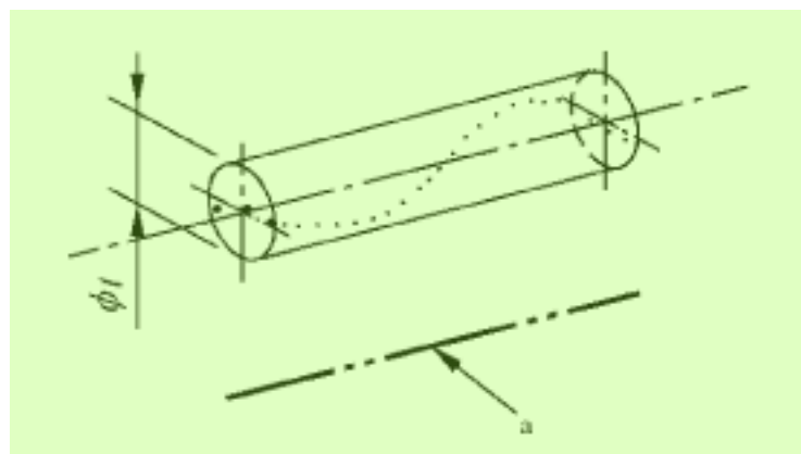
图 119 平行度公差带的定义 12
