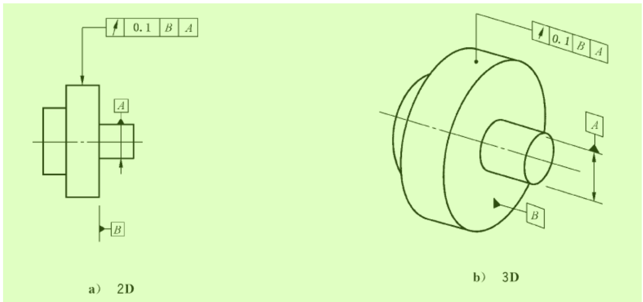
图 173 圆跳动标注 2
