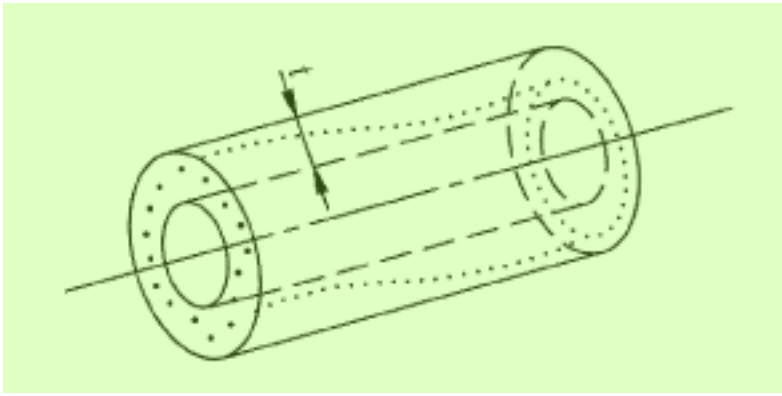
图 103 圆柱度公差带的定义
