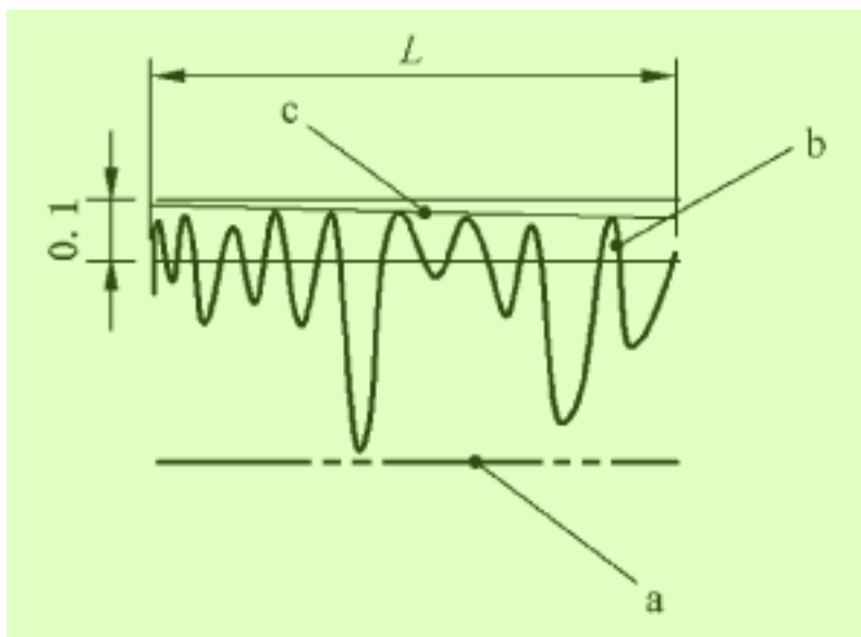
图 31 贴切拟合被测要素——图样标注
