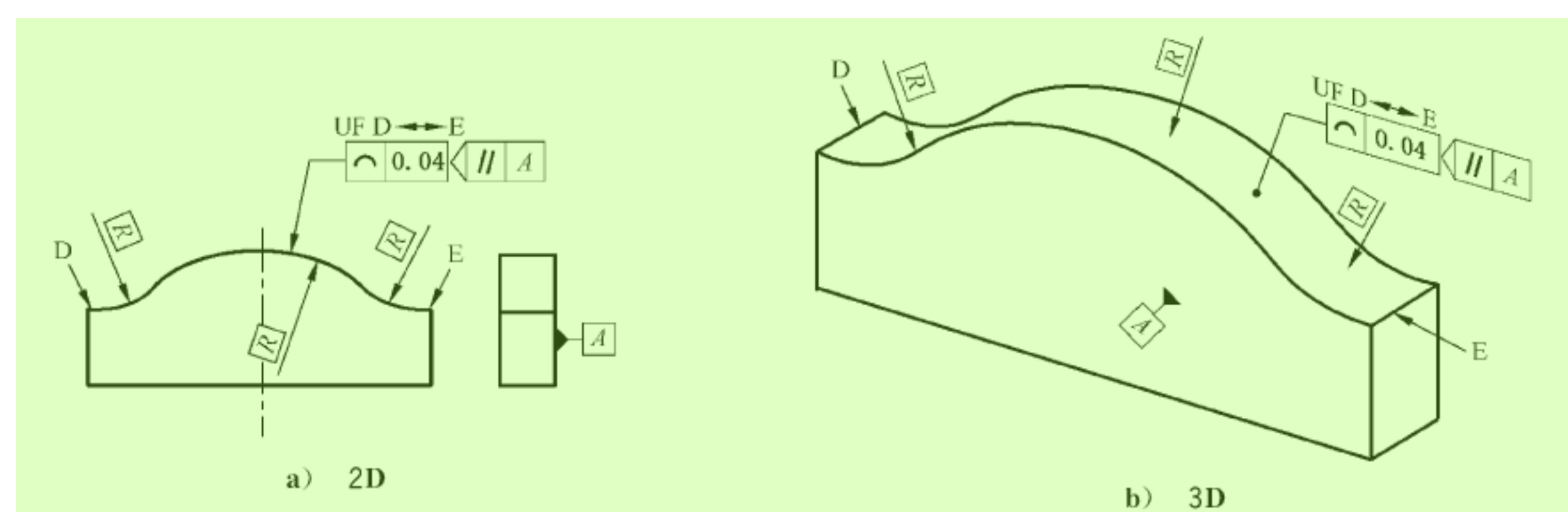
图 104 线轮廓度标注
