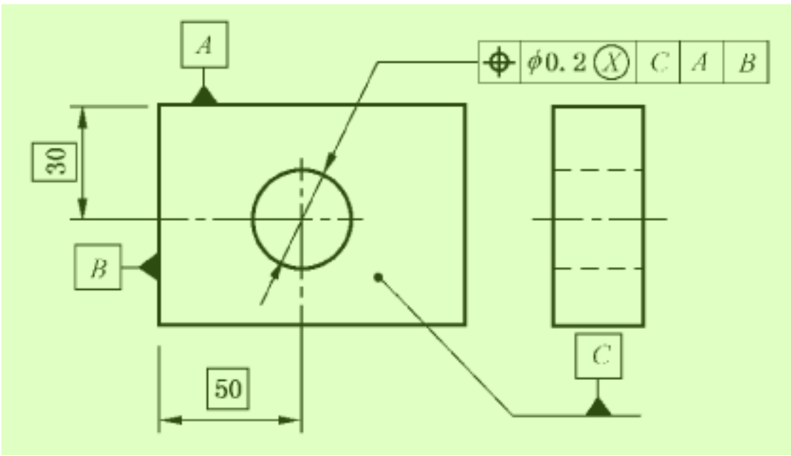
图 33 最大内切拟合被测要素——图样标注
