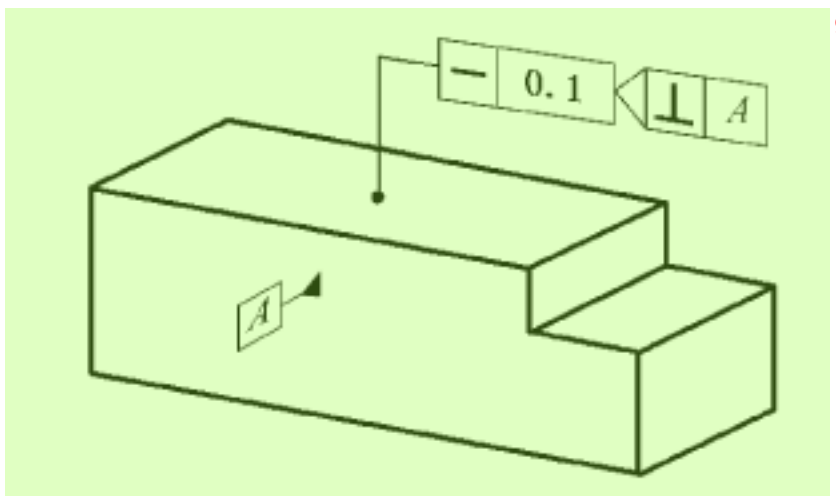
图 80 使用垂直于基准的相交平面规范 10
