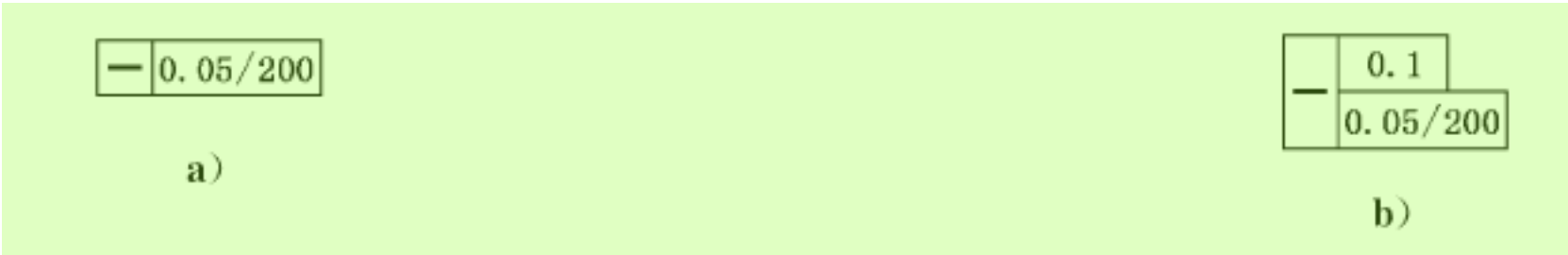
图 66 局部规范的标注
