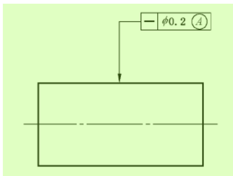
图 37 适用于中心要素的规范 2
