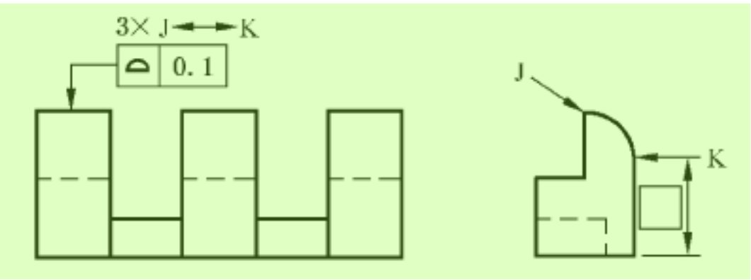
图 63 多个组合被测要素的标注
