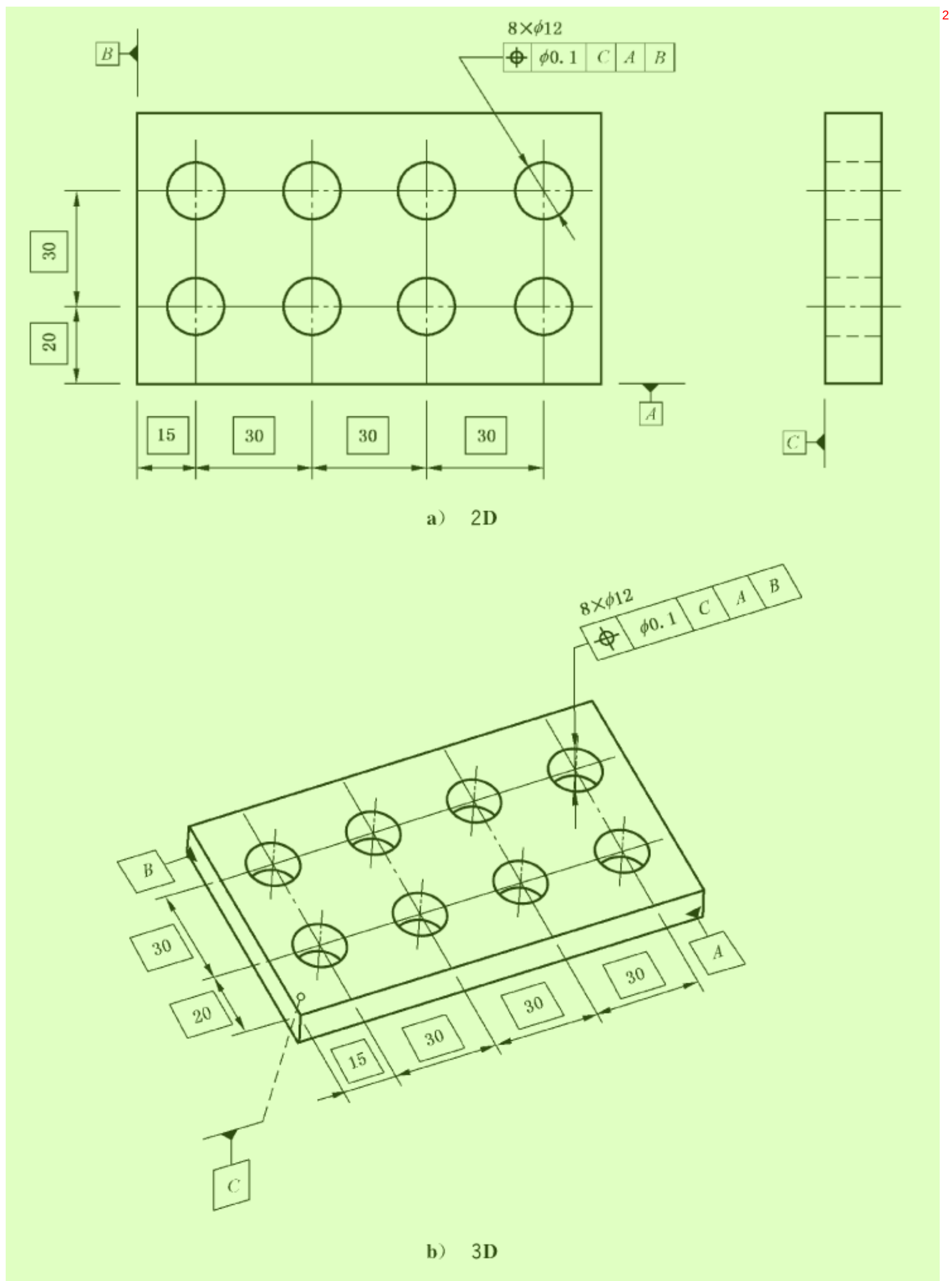
图 155 位置度标注 3
