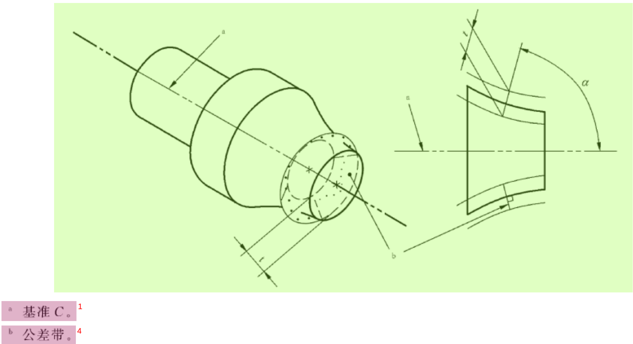
图 183 圆跳动公差带的定义 3
