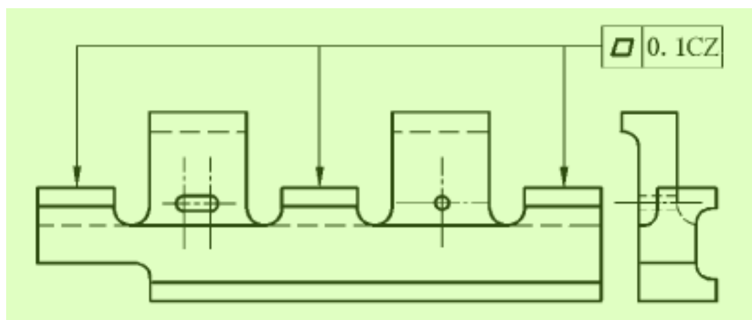
图 19 适用于多个要素的组合公差带规范
