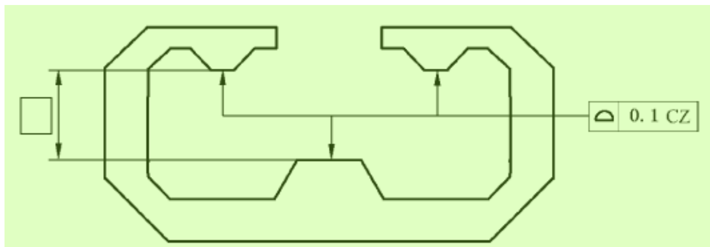
图 19 适用于多个要素的组合公差带规范
