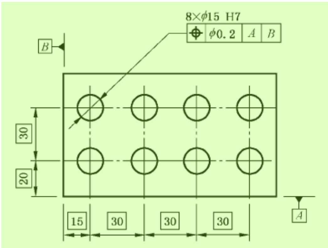
图 64 线性 TED 的标注
