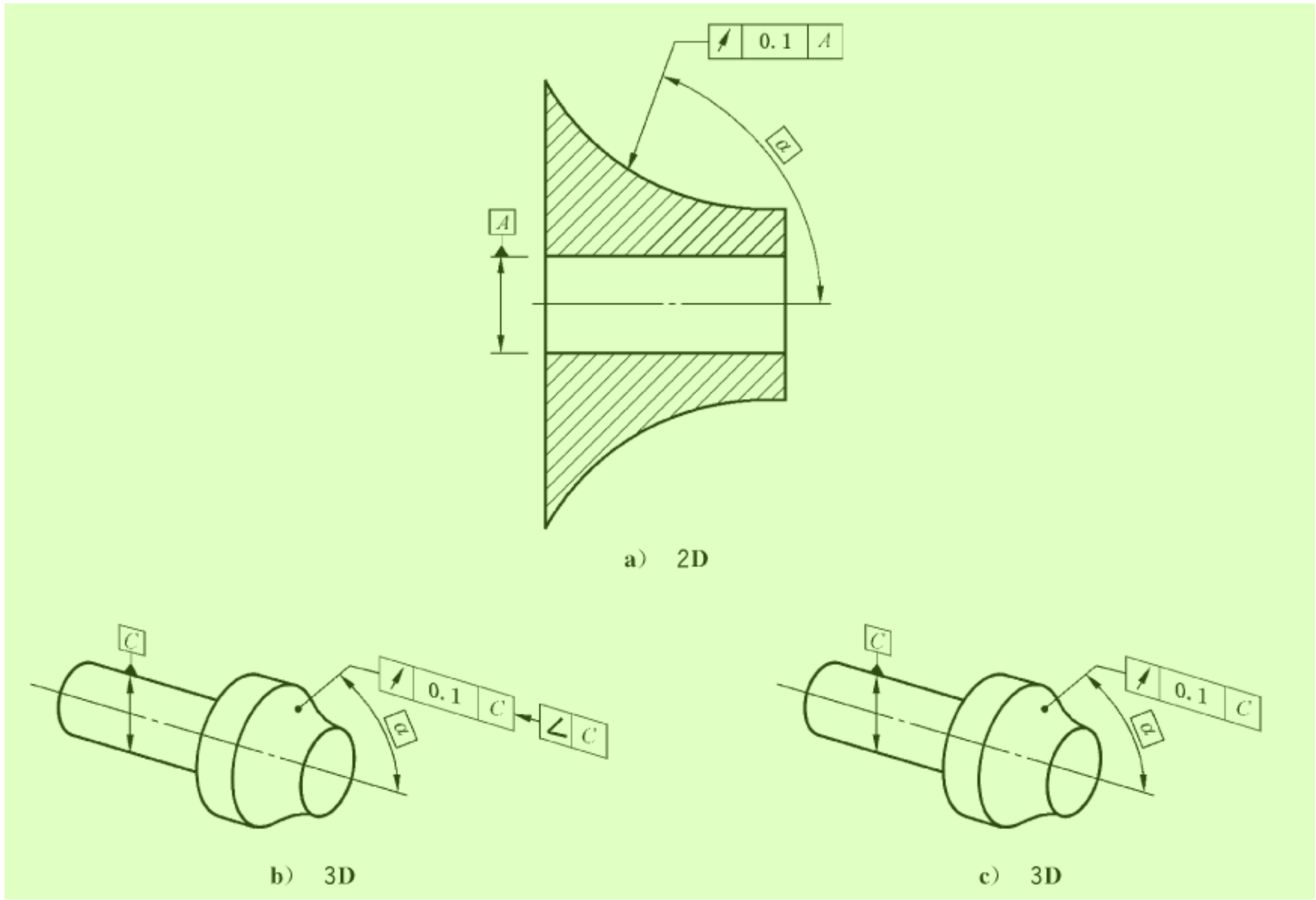
图 85 图样标注 3
