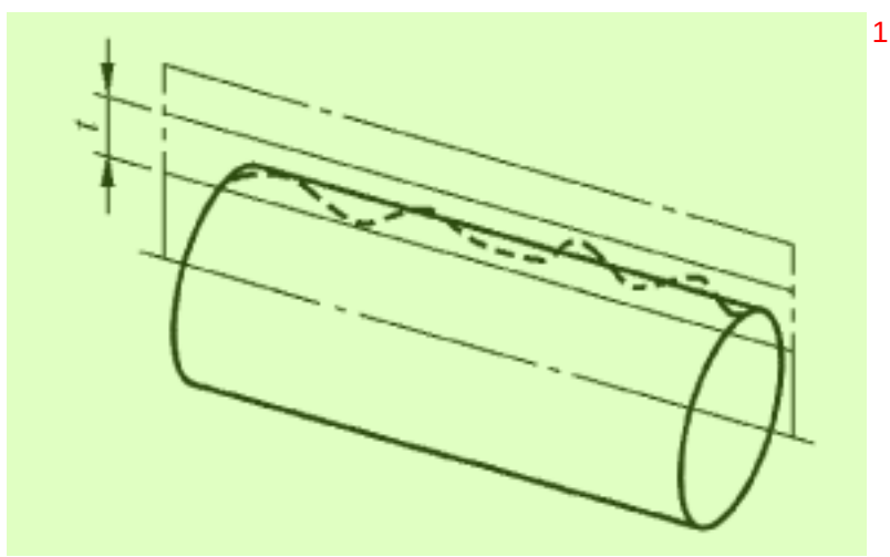
图 93 直线度公差带的定义
