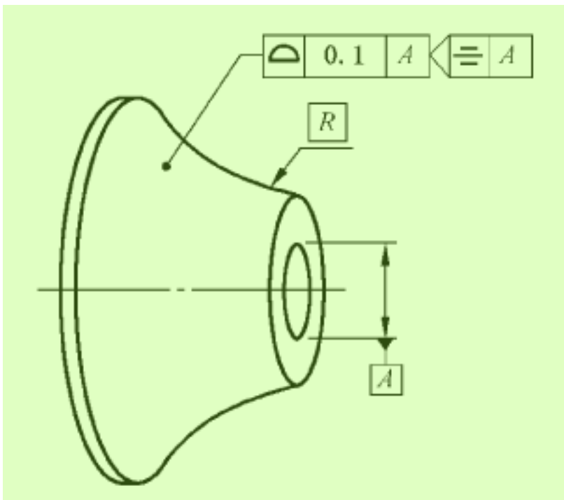
图 81 使用对称于(包含)基准的相交平面规范 12
