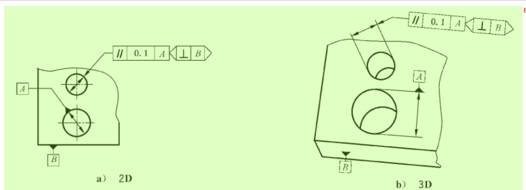
图 114 平行度标注
