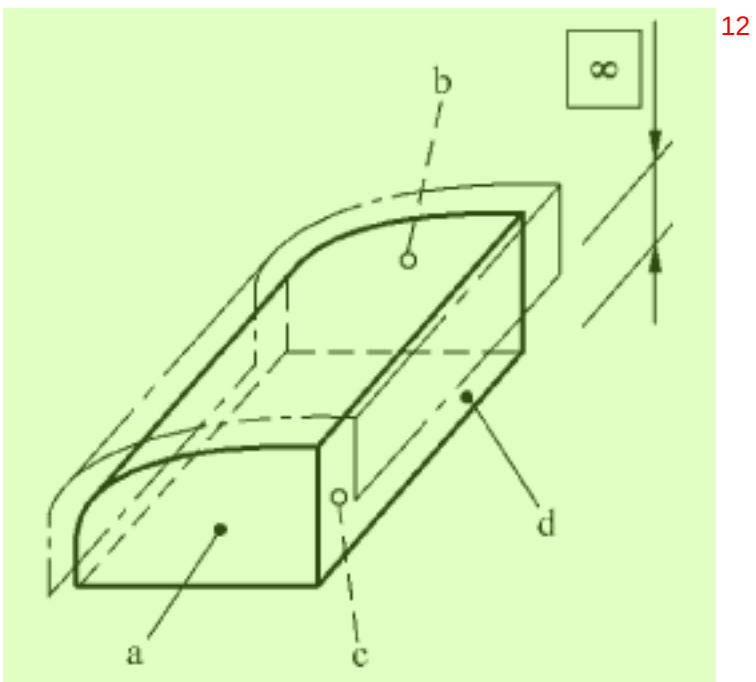
图 61 说明:长点划线勾勒出被测要素的轮廓——面要素 a、b、c 与 d 的下部不在规范的范围 内 13
