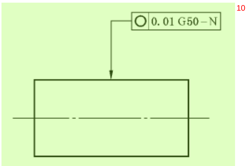
图 42 使用滤波与最小外接参照要素的规范 11
