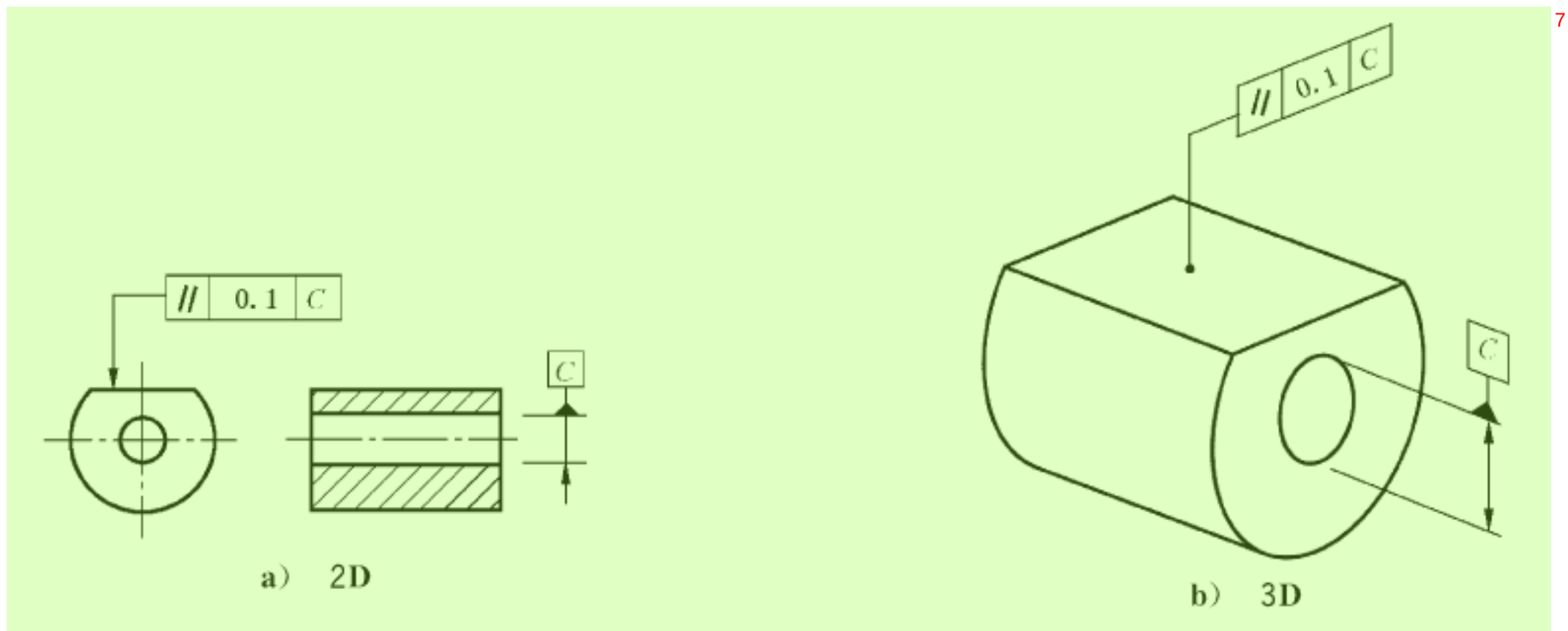
图 124 平行度标注 8
