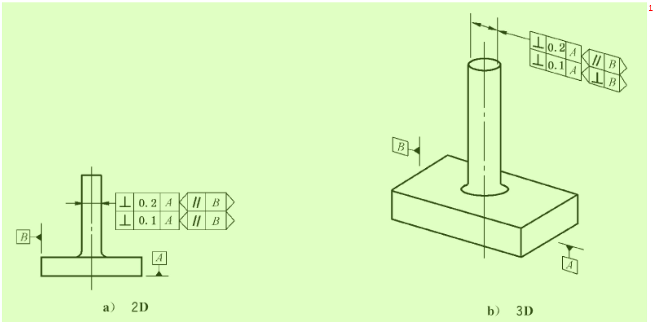
图 132 垂直度标注
