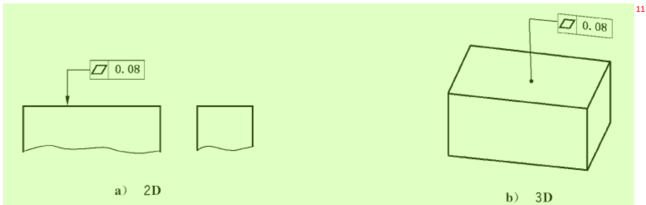
图 96 平面度标注
