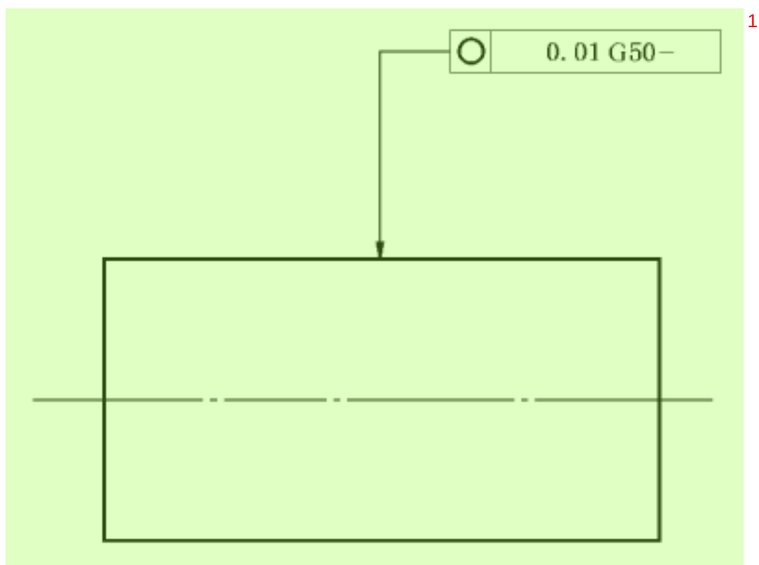
图 E.13 圆度公差示例——高斯滤波器 2
