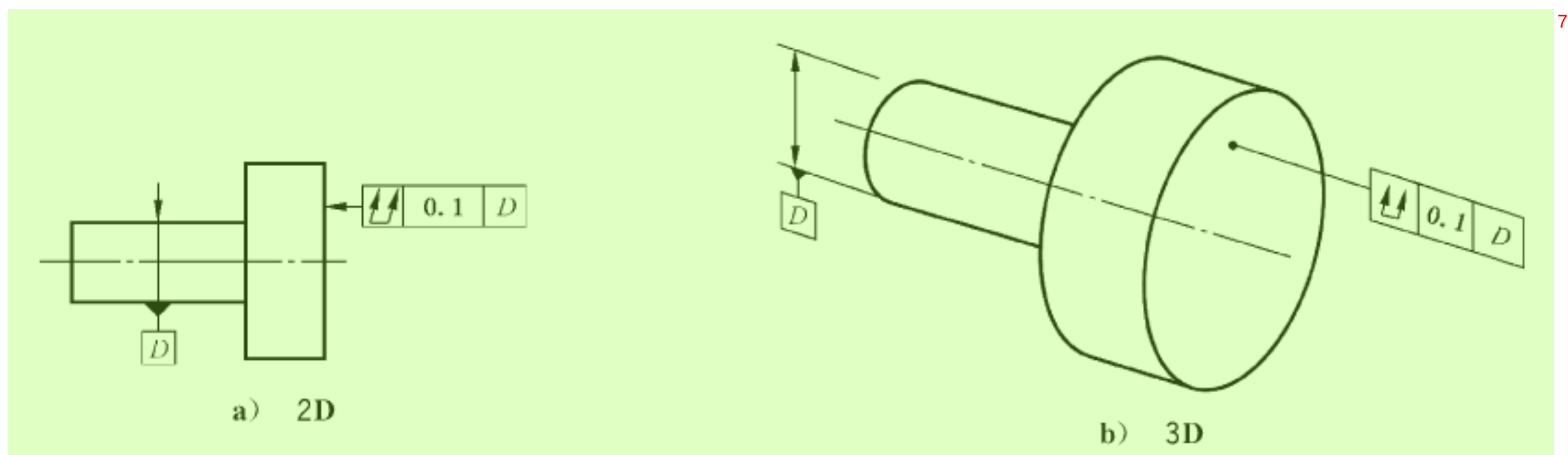
图 186 全跳动标注 7
