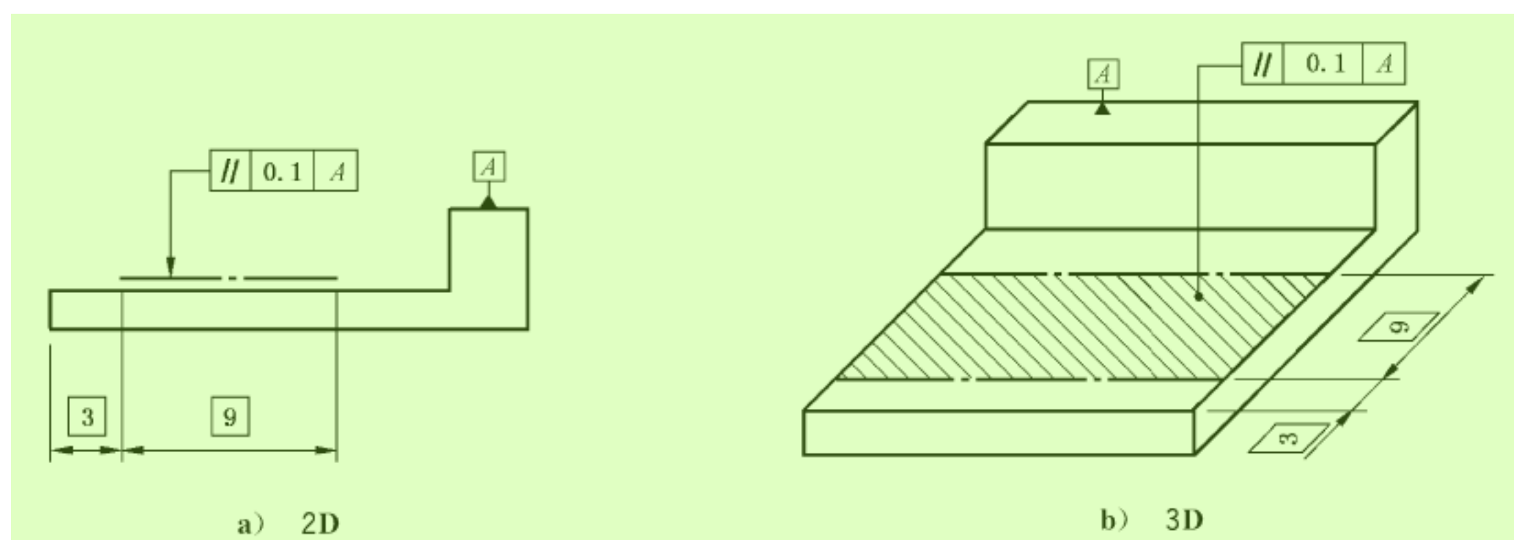
图 58 局部区域标注 7
