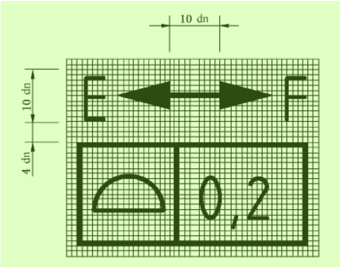
图 F.4 方向要素框格
