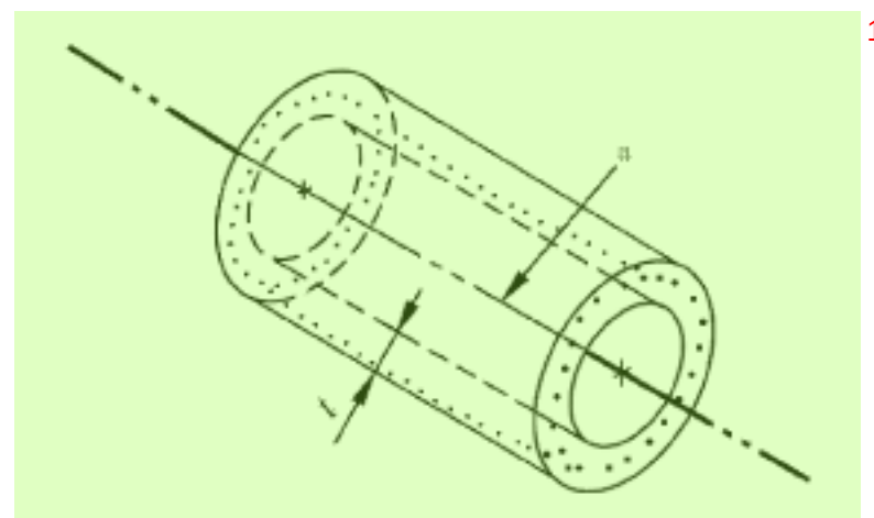
图 185 全跳动公差带的定义 2
