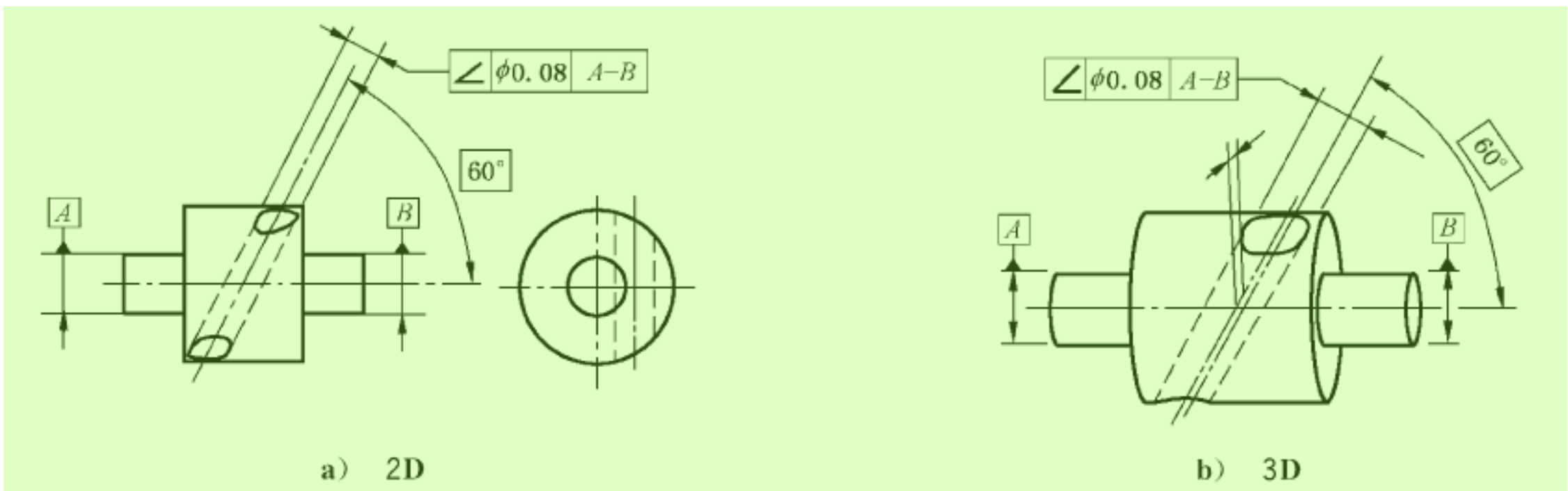
图 142 倾斜度
