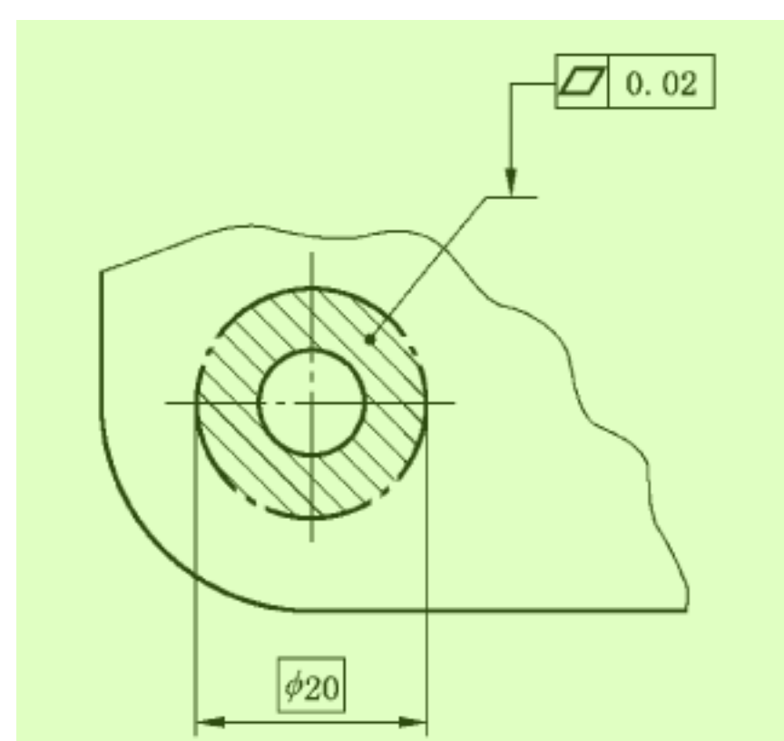
图 59 局部区域标注 10
