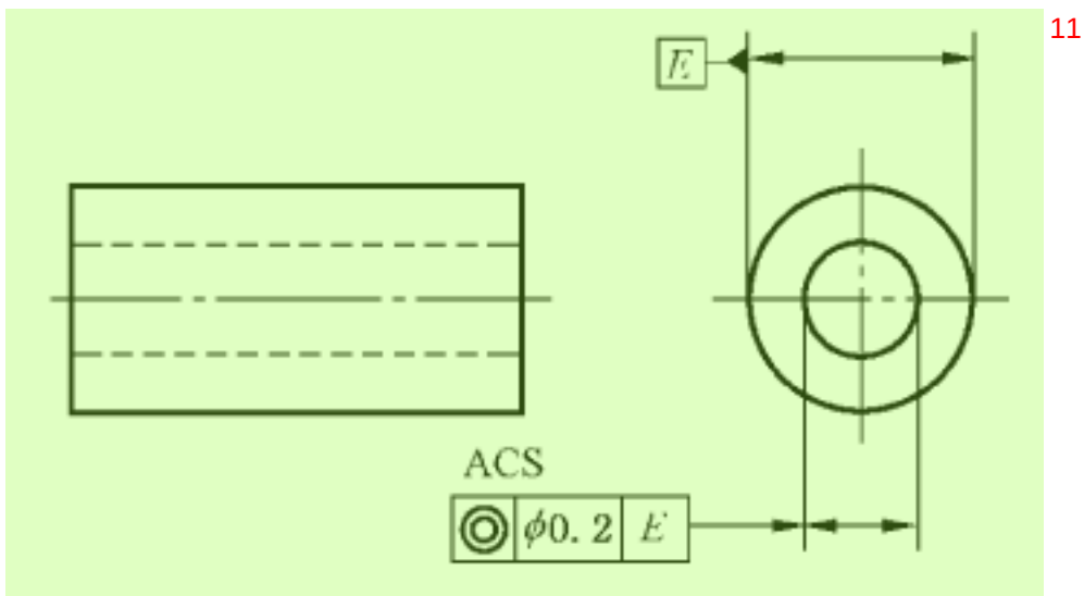
图 47 应用于任何横截面的规范标注 11
