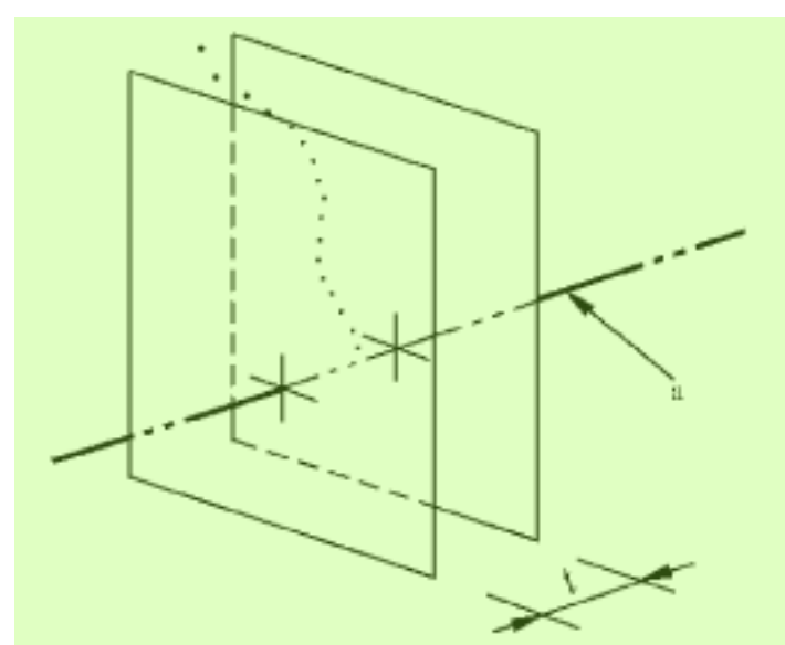
图 129 垂直度公差带的定义
