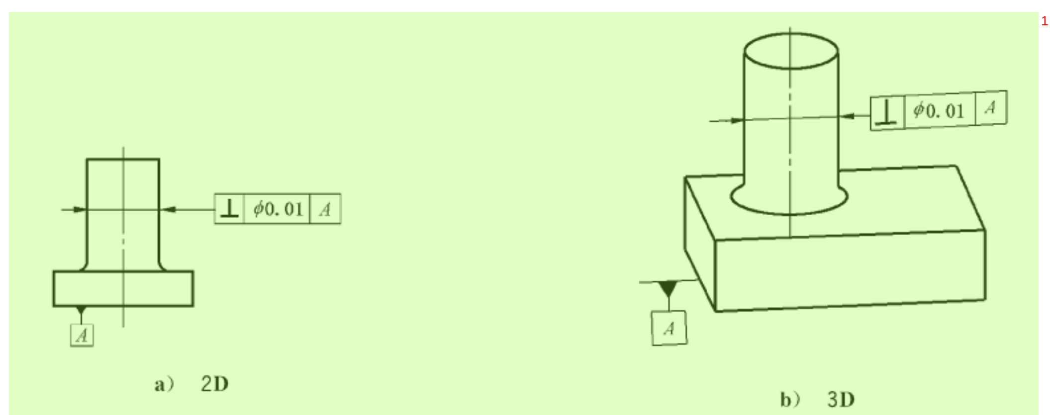
图 134 垂直度标注 2
