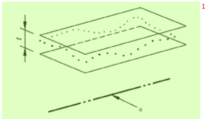
图 125 平行度公差带的定义 12
