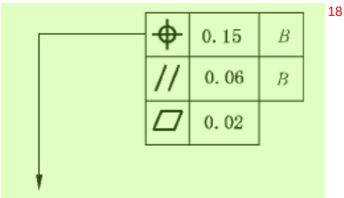
图 50 多层公差标注
