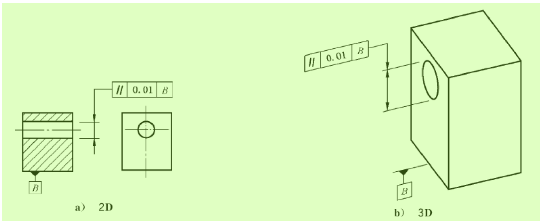
图 120 平行度标注 2
