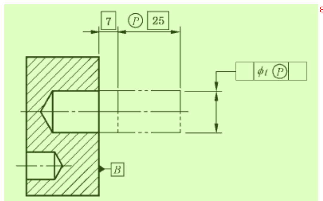
图 72 直接标注带偏置量的延伸公差带示例 8
