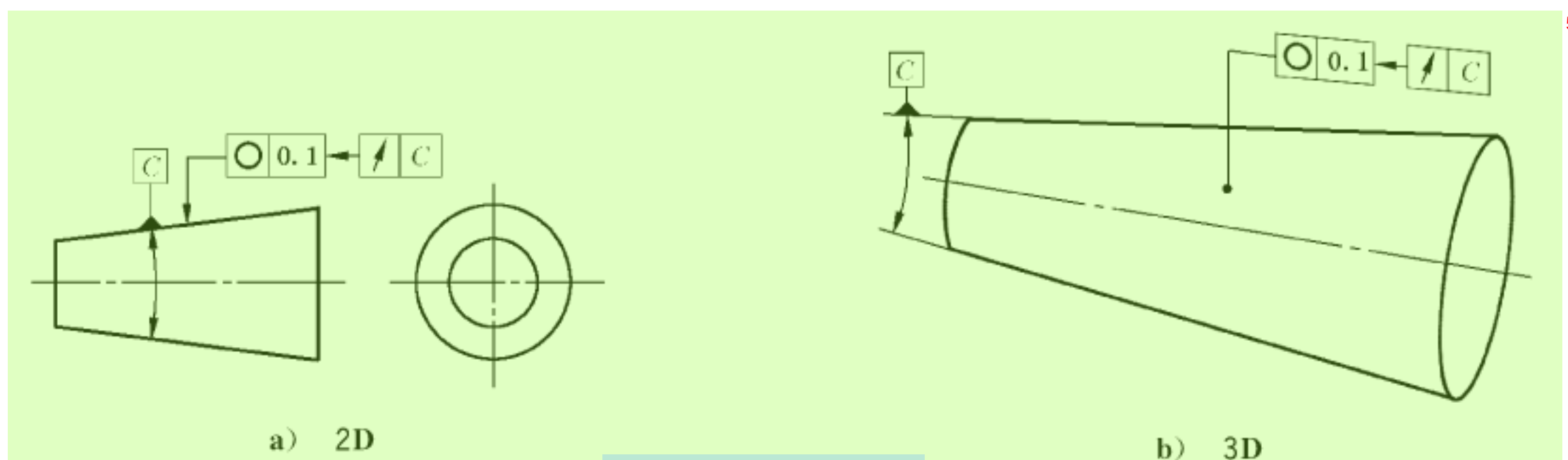
图 100 圆度标注 6
