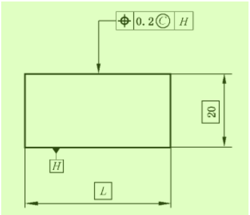
图 25 最小区域(切比雪夫)拟合被测要素——图样标注
