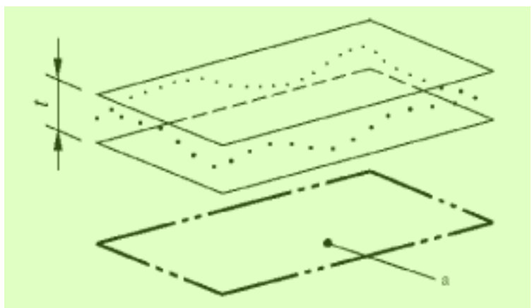
图 127 平行度公差带的定义
