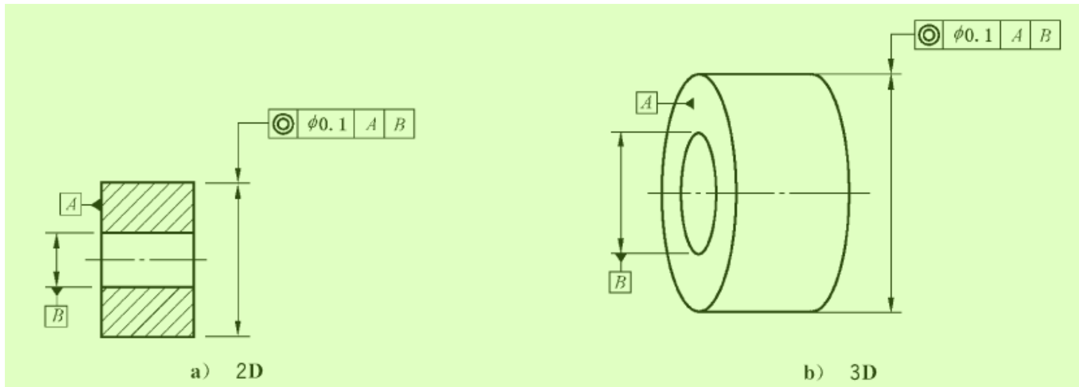
图 167 同轴度标注 6
