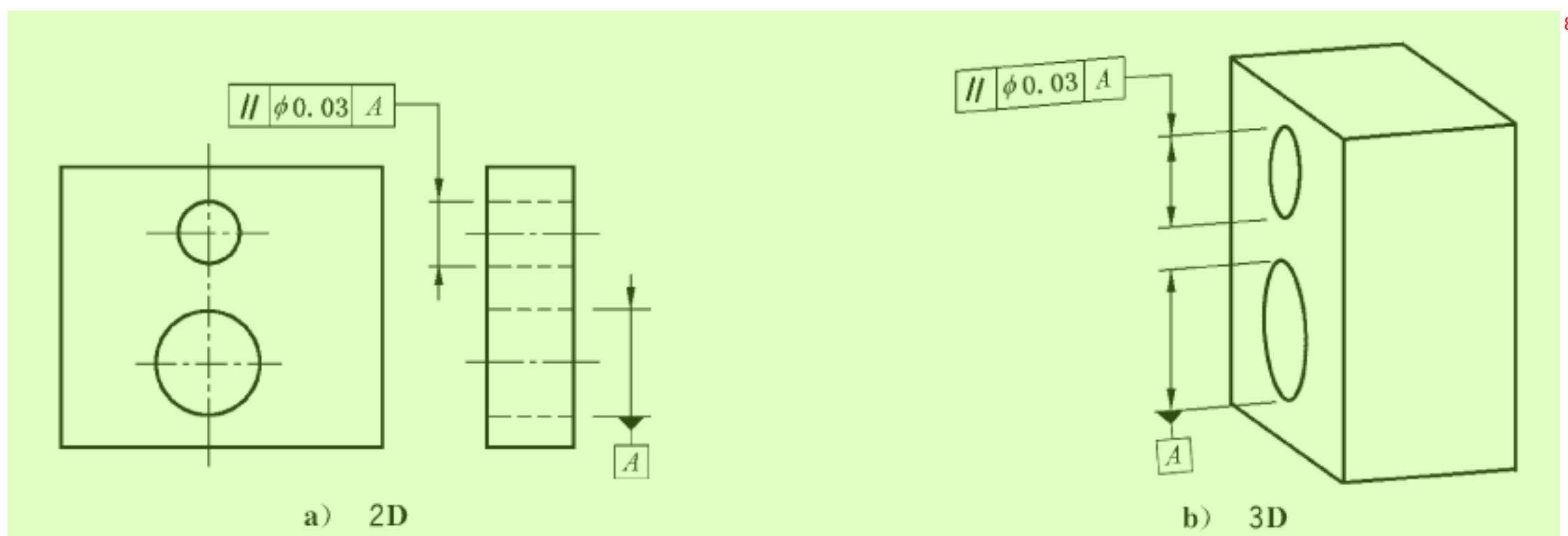
图 118 平行度标注 9
