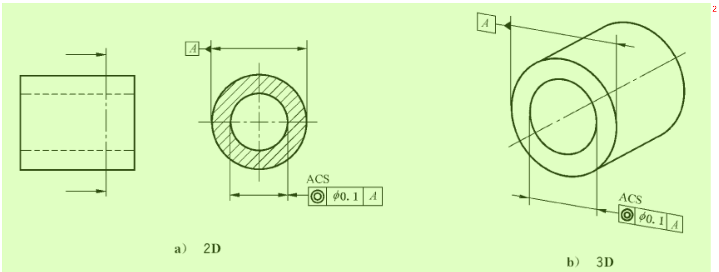
图 163 同心度标注 3
