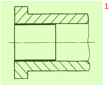
图 11 装配图中狭小面积的剖面可用涂黑代替剖面符号
