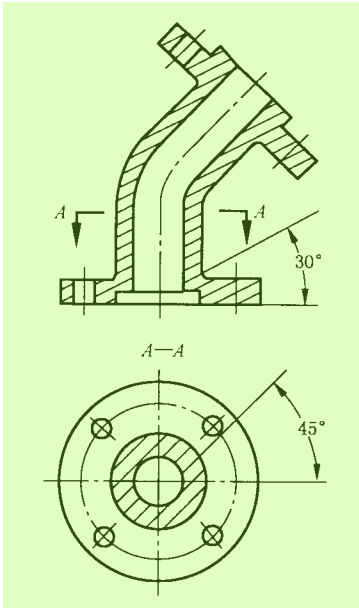
图 2 与主要轮廓线成适当角度剖面线的应用示例
