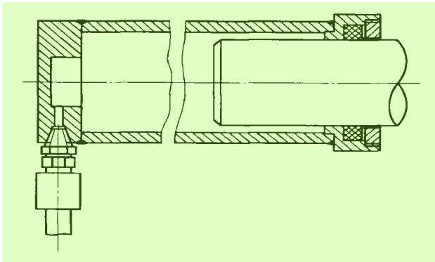
图 10 绘制接合件与其他零件的装配图时剖面符号绘制方法 7
