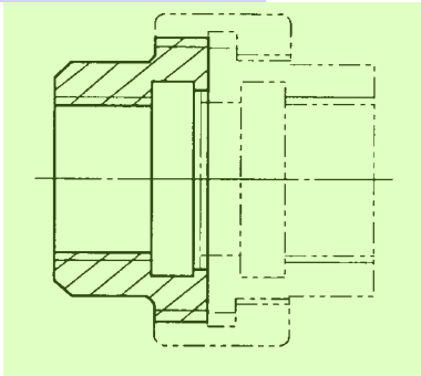
图 3 相邻辅助零件(或部件)不画剖面符号
