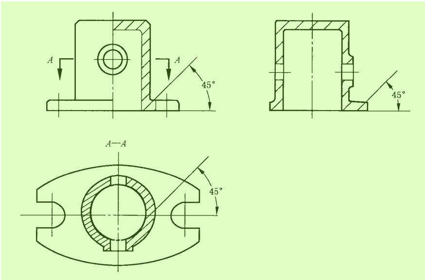
图 1 与主要轮廓线成 45°剖面线的应用示例 6
