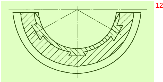
图 7 接合件图中各零件的剖面符号绘制方法(一)
