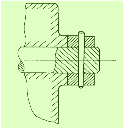
图 4 剖面区域较大时可以只沿轮廓的周边画出剖面符号
