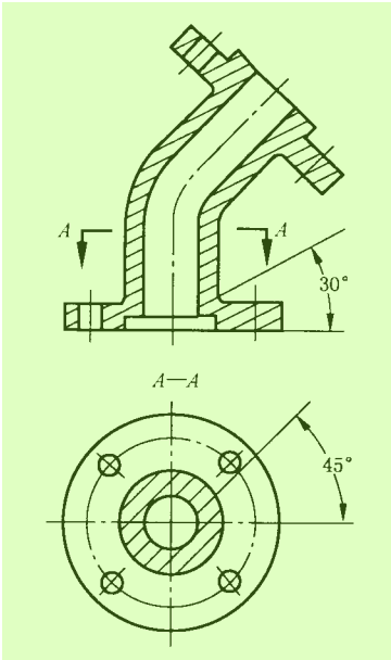
图 2 与主要轮廓线成适当角度剖面线的应用示例
