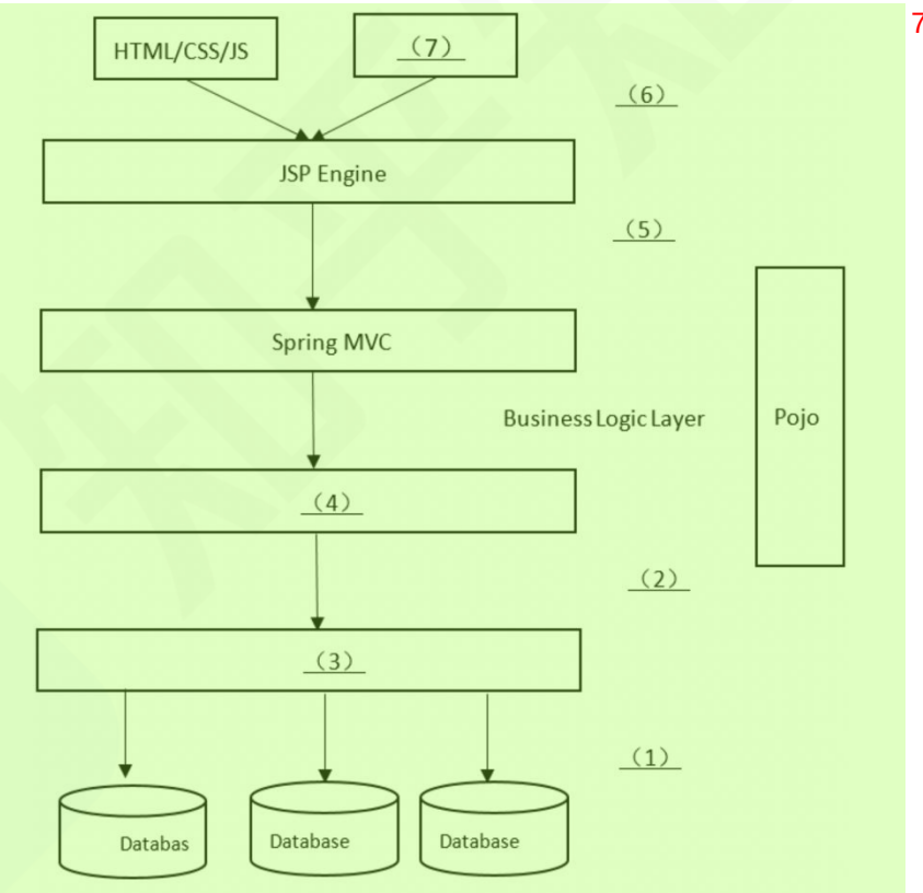
图 5-1 SSM 框架工作流程图8
