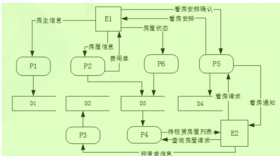
图 2-1 房屋租赁服务系统顶层 DFD
