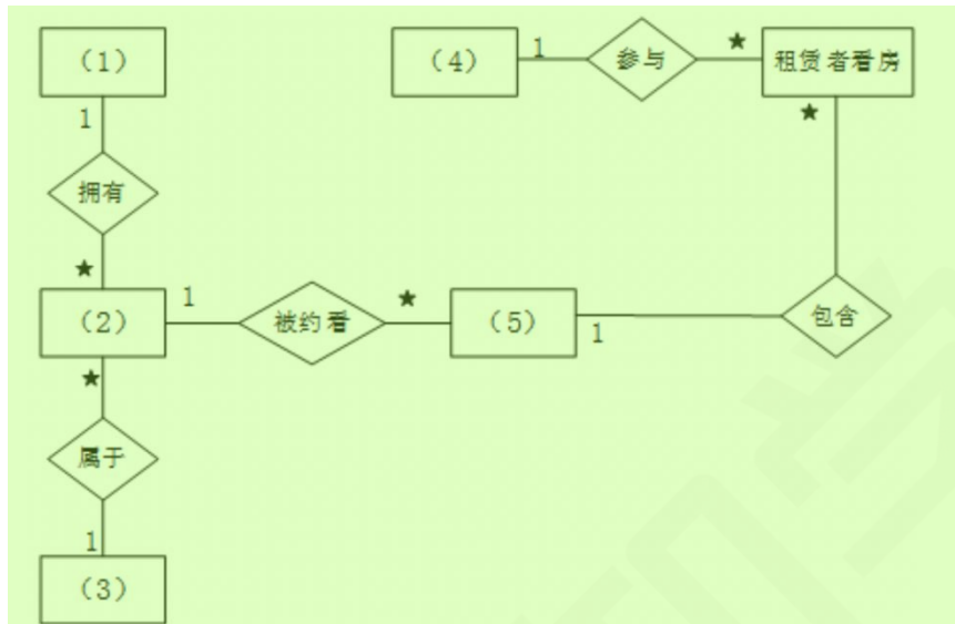
图 2-2 房屋租赁服务系统 ERD 4
