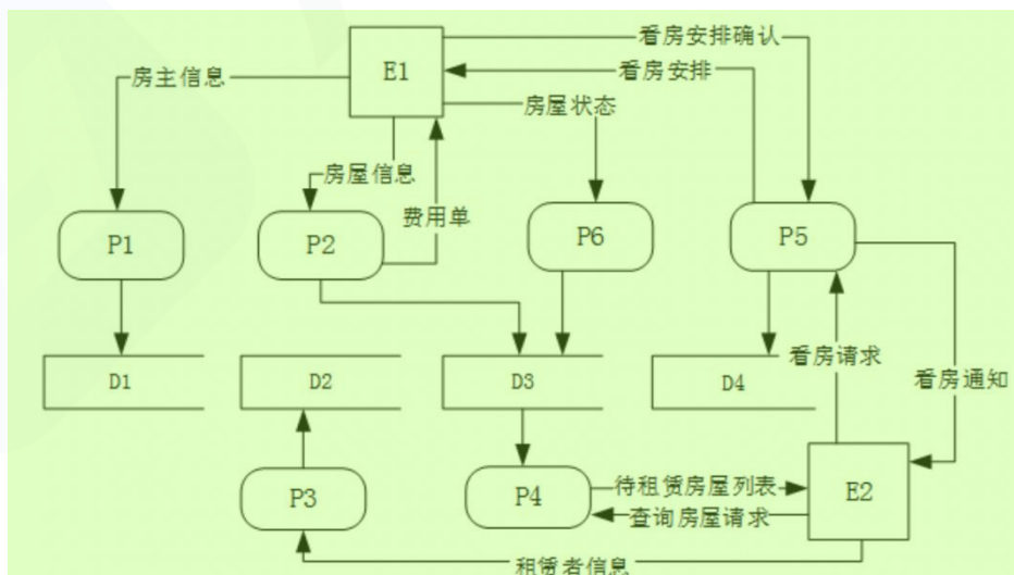
图 2-1 房屋租赁服务系统顶层 DFD 14
