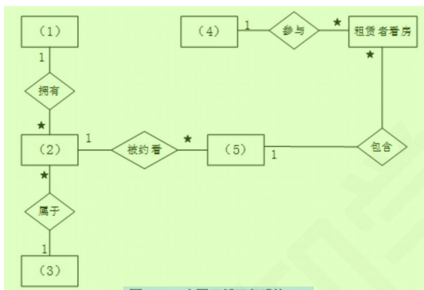
图 2-2 房屋租赁服务系统 ERD 4
