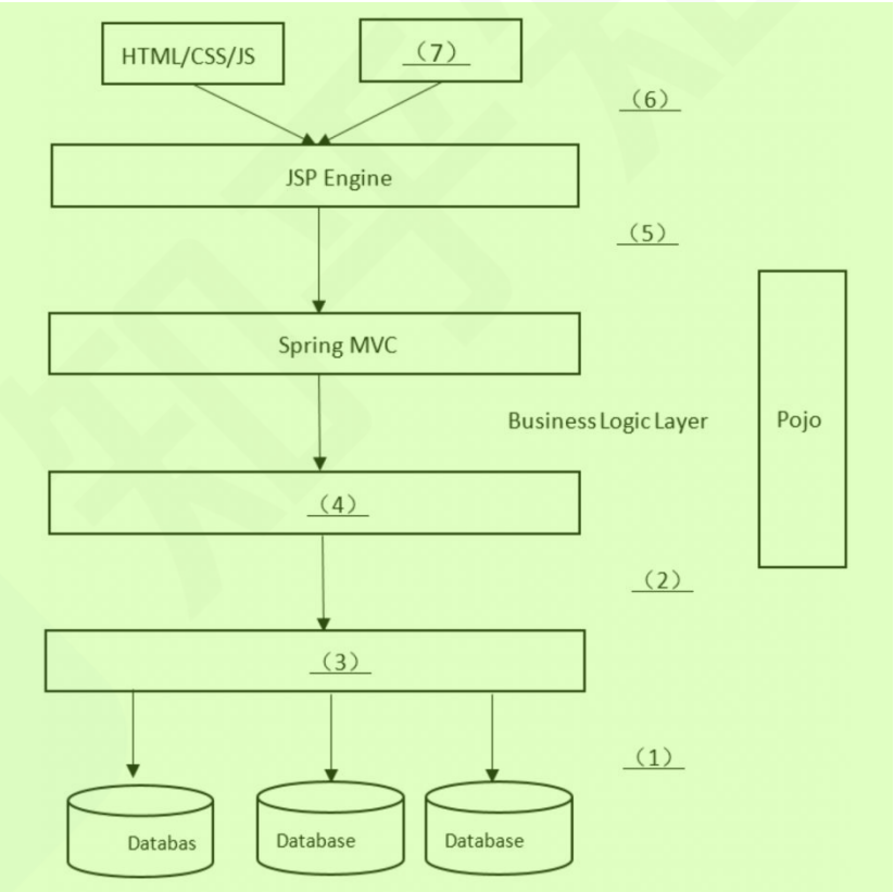
图 5-1 SSM 框架工作流程图 16
