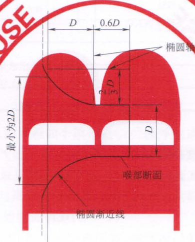
图 B.6 喷嘴
