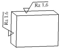
图 1 粗糙度标注在表面上
