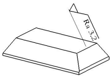
图 2 粗糙度标注在表面延长线上
