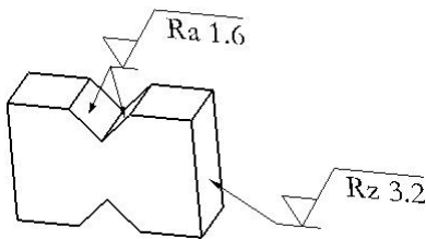
图 3 粗糙度标注在指引线上
