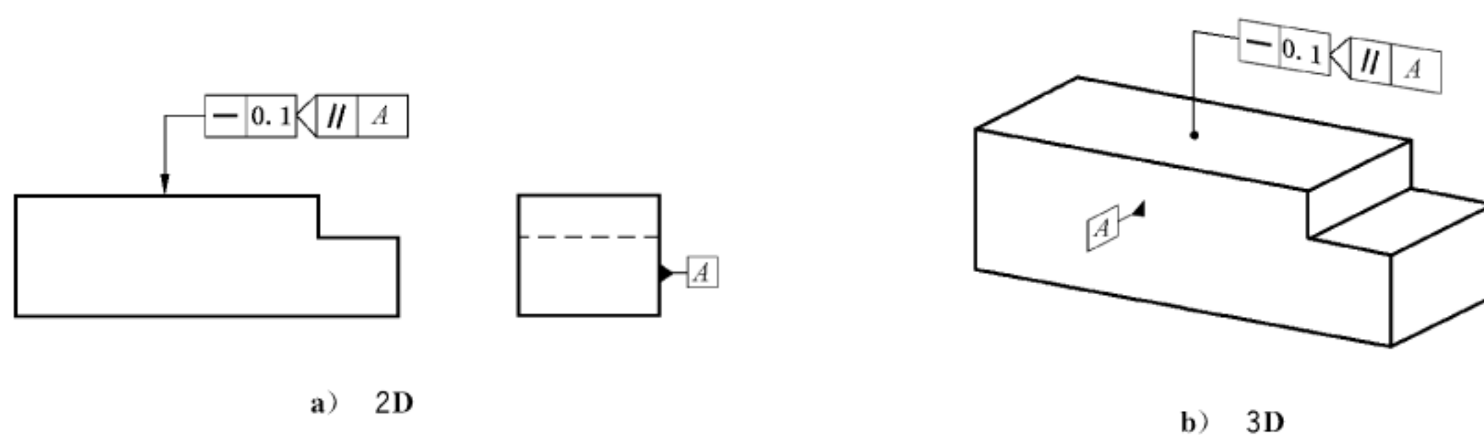
图 90 直线度标注
