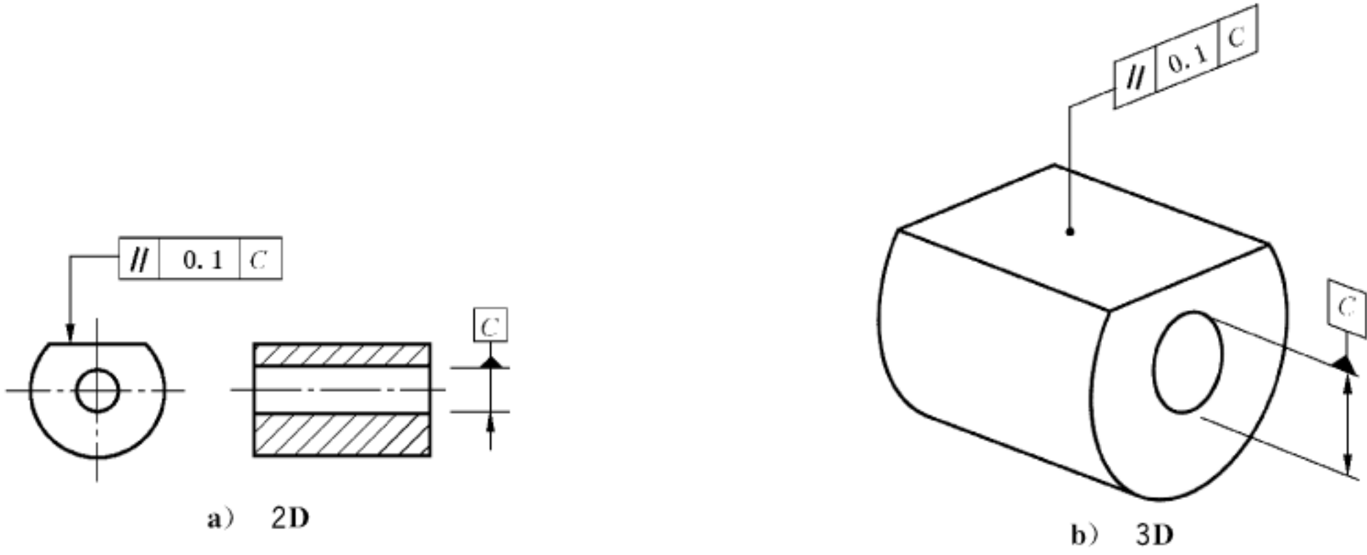
图 124 平行度标注
