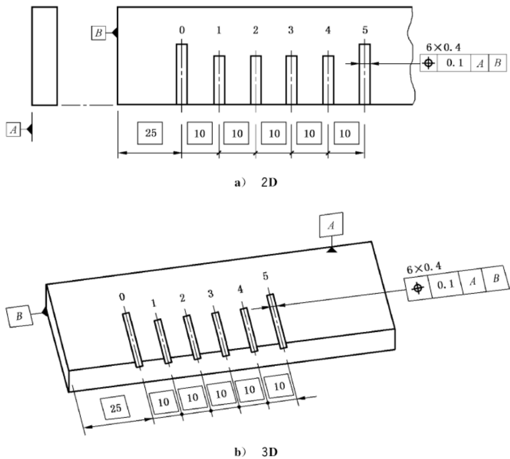
图 157 位置度标注
