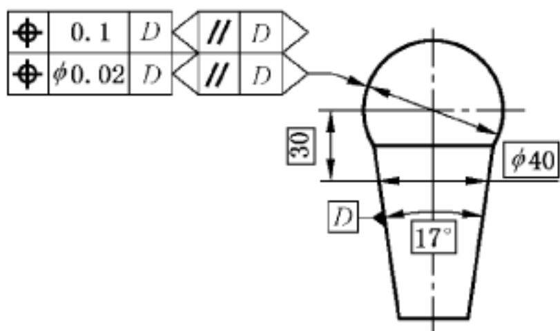
图 84 使用定向平面同时确定圆柱公差带以及由两个平行平面约束的公差带方向的规范
