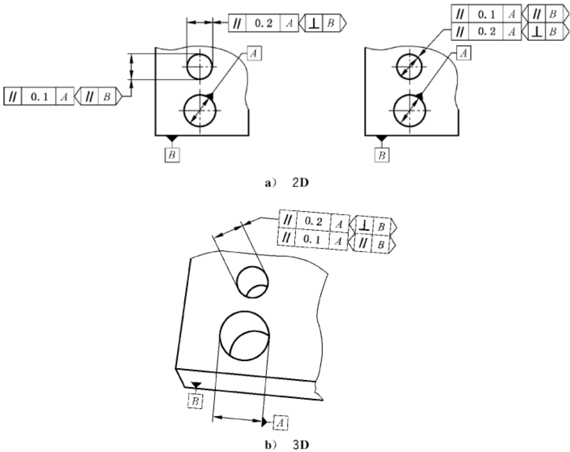
图 116 平行度标注
