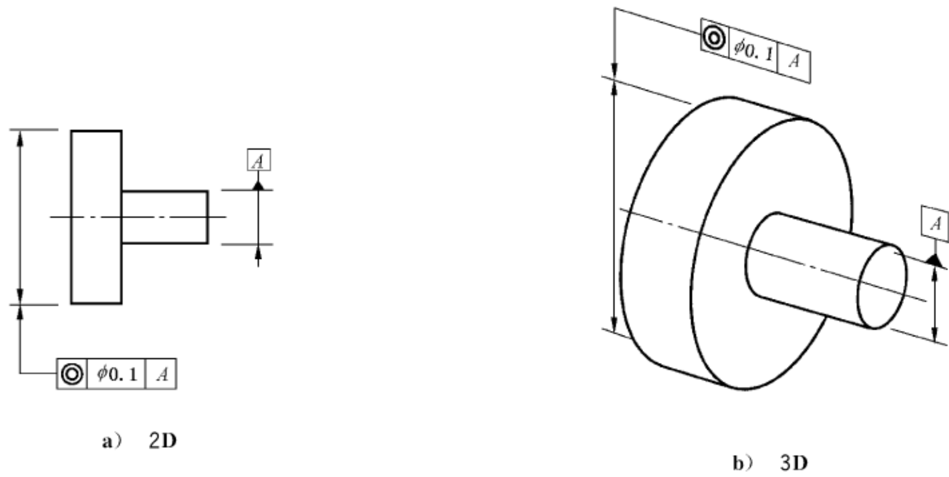
图 166 同轴度标注
