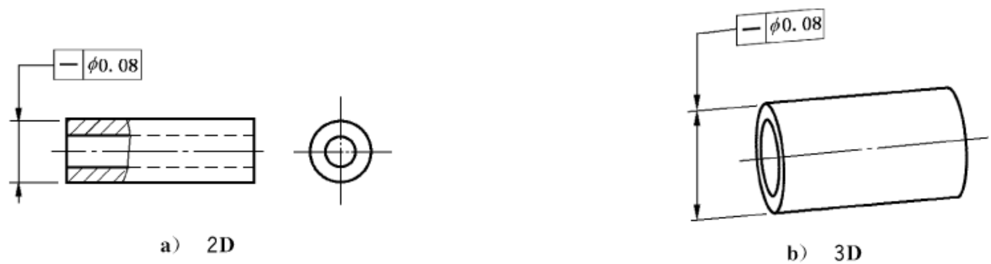
图 94 直线度标注
