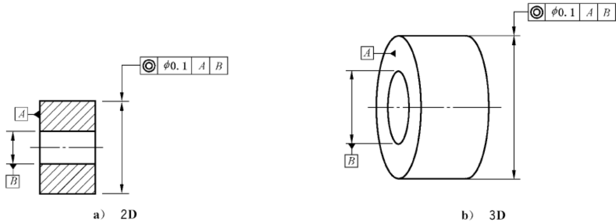
图 167 同轴度标注
