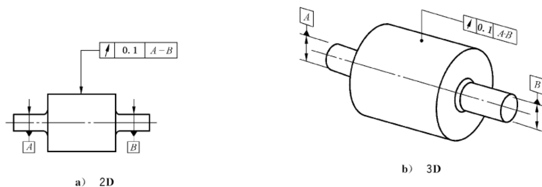
图 174 圆跳动标注
