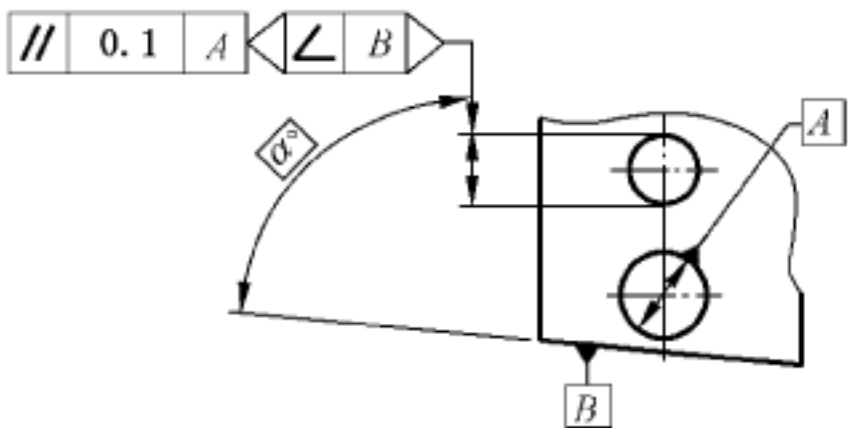
图 83 使用与基准保持特定的角度的定向平面规范
