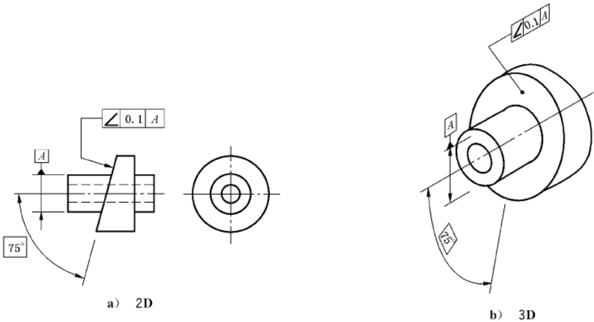
图 146 倾斜度标注
