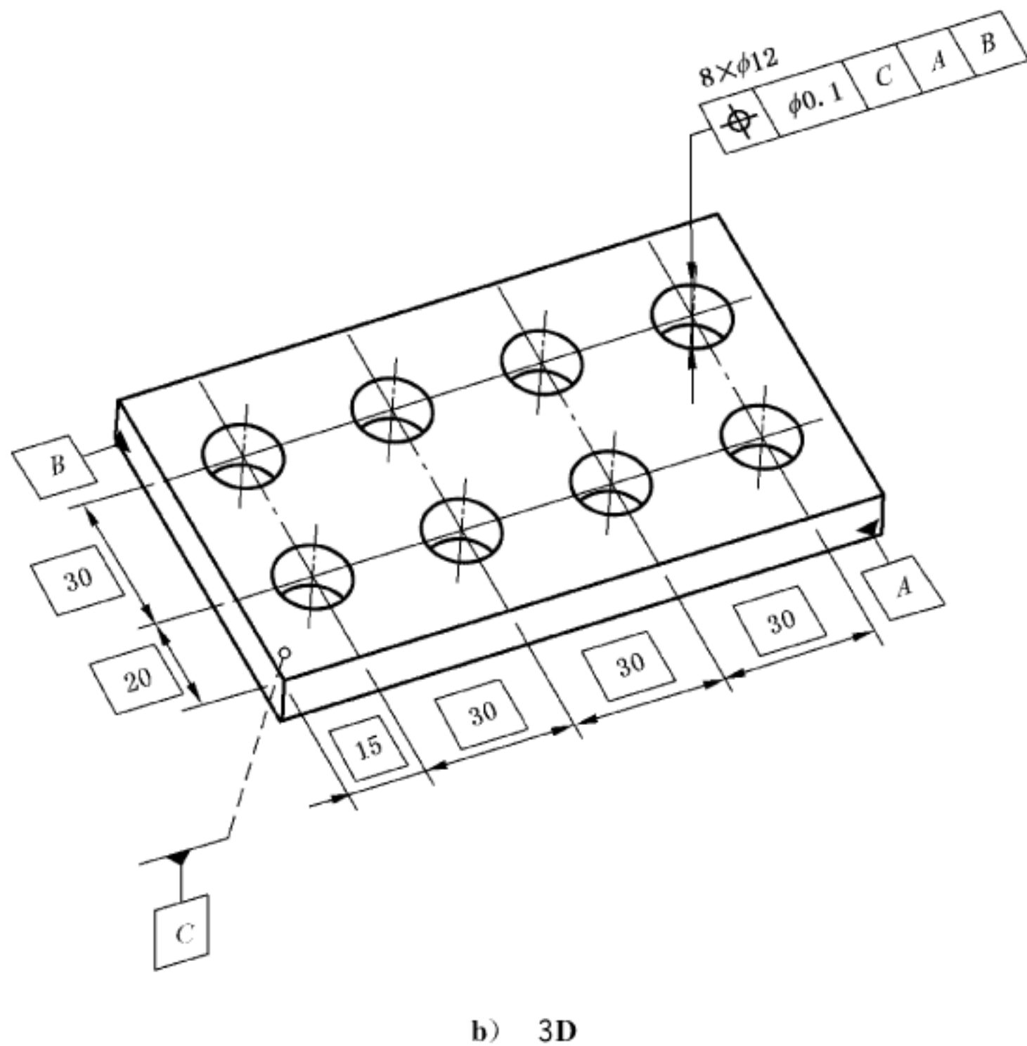
图 155 位置度标注
