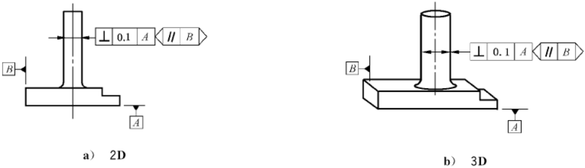
图 130 垂直度标注
