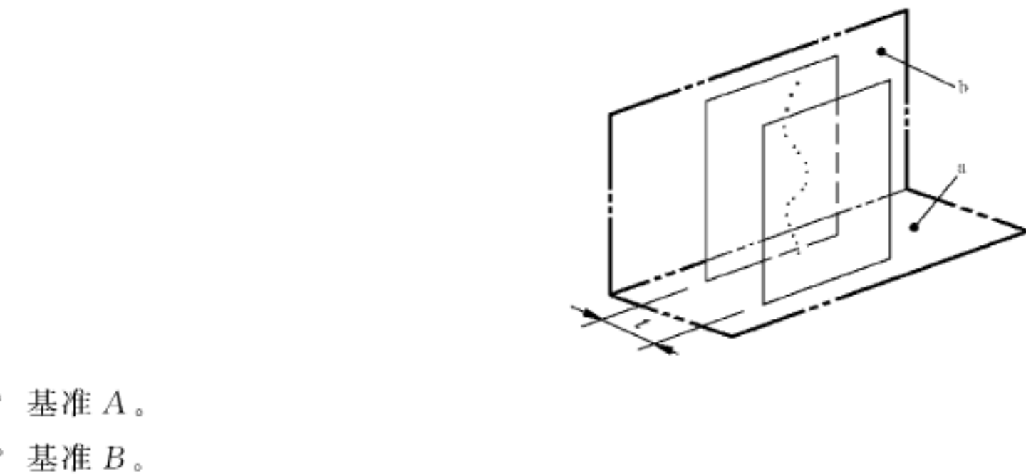
图 131 垂直度公差带的定义
