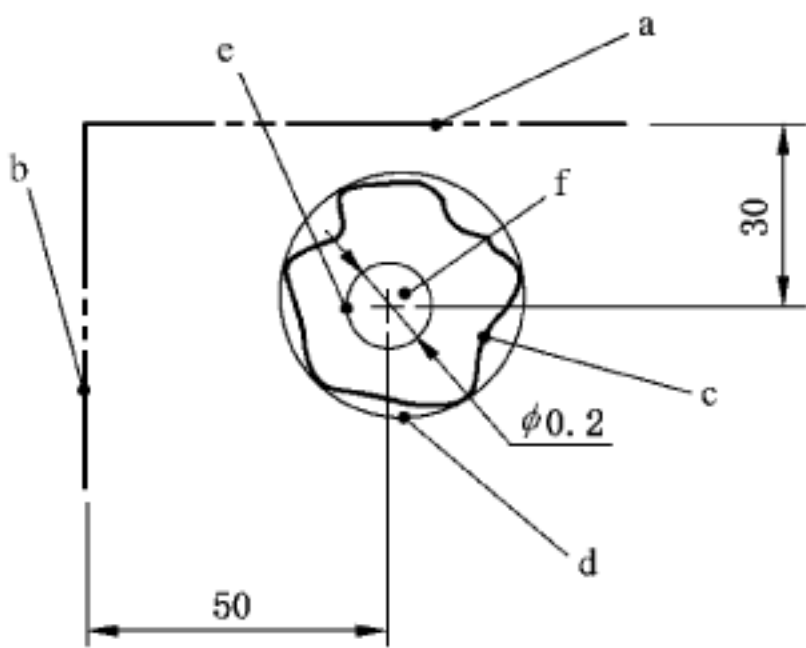
图 29 最小外接拟合被测要素——图样标注
