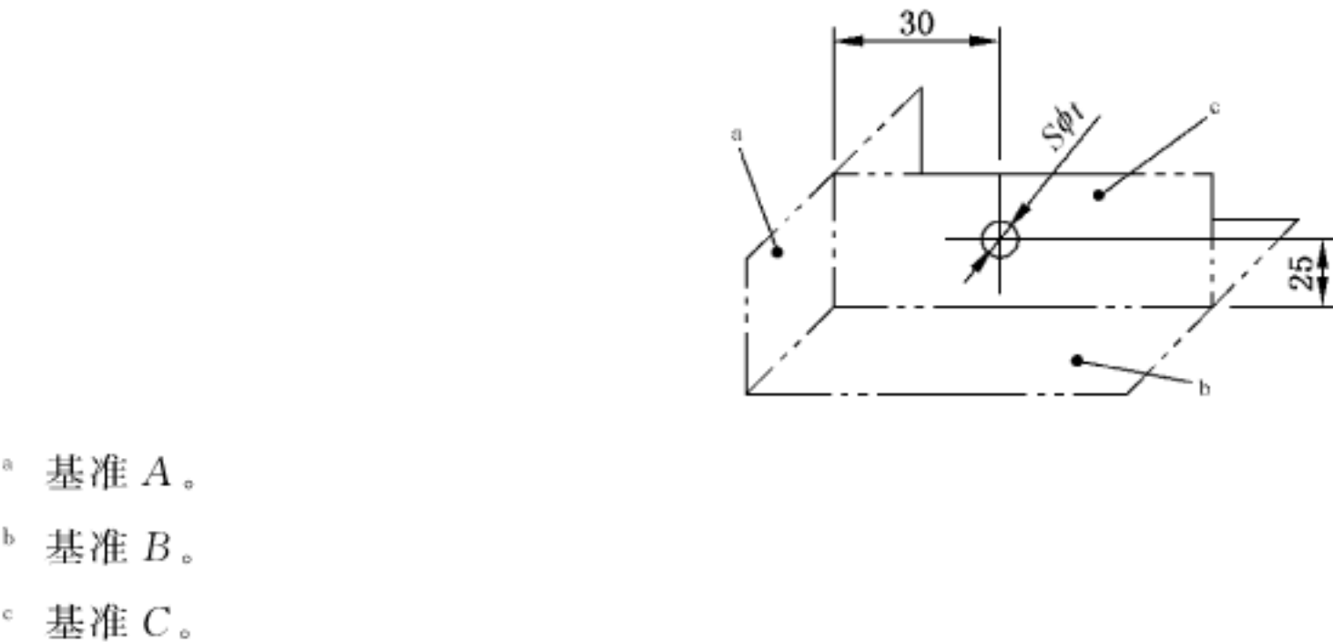
图 151 位置度公差带的定义
