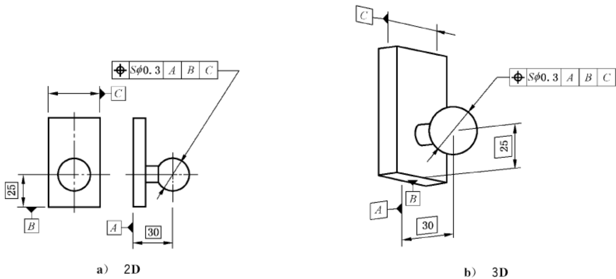
图 150 位置度标注
