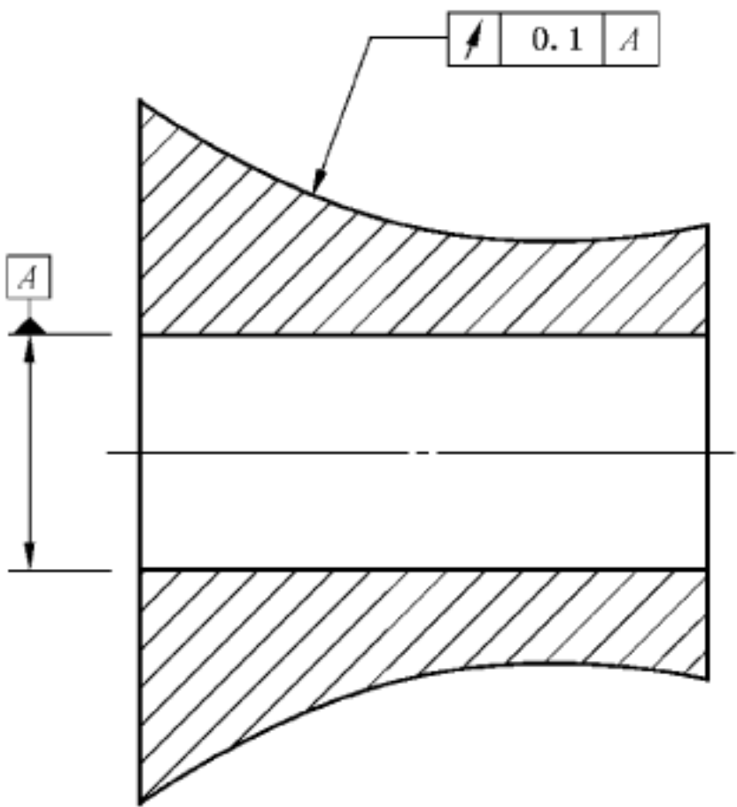
图 8 图样标注
