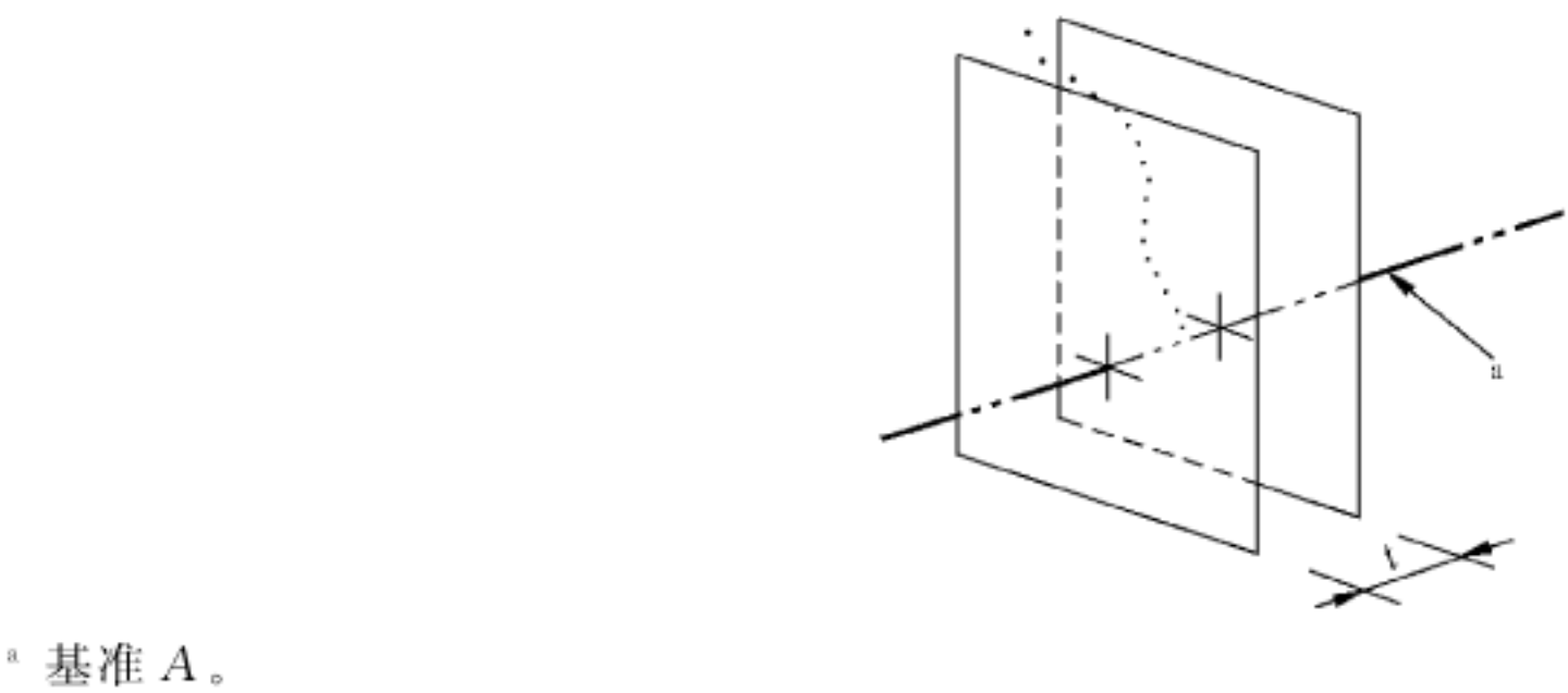
图 129 垂直度公差带的定义
