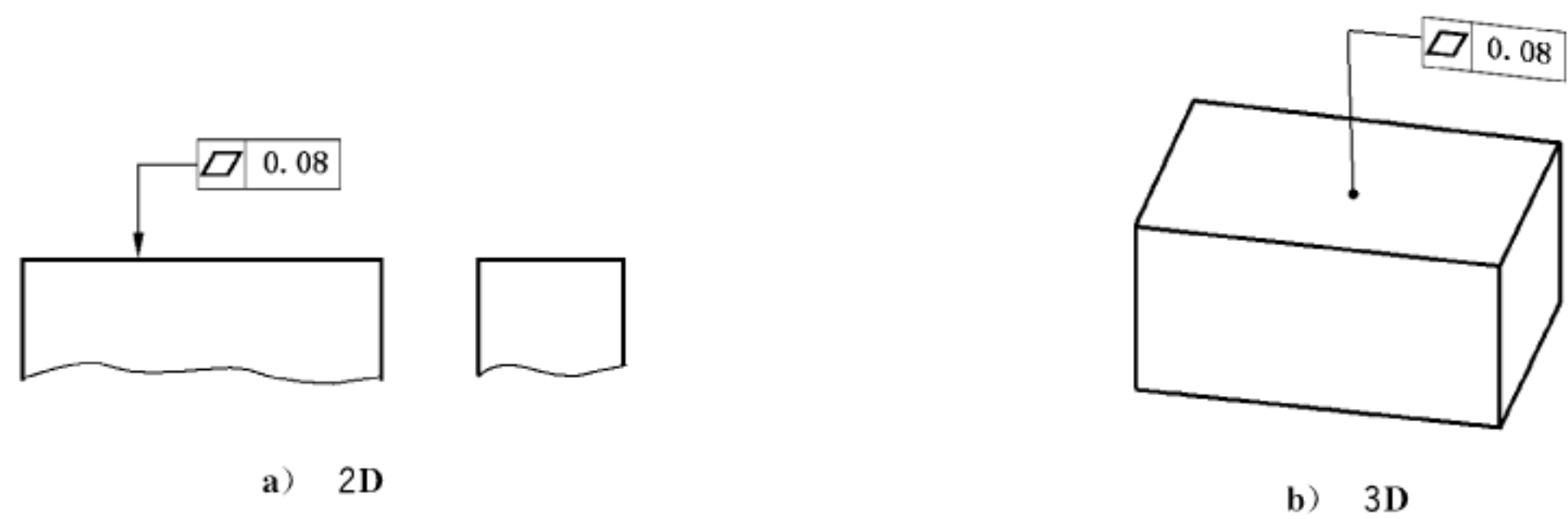
图 96 平面度标注
