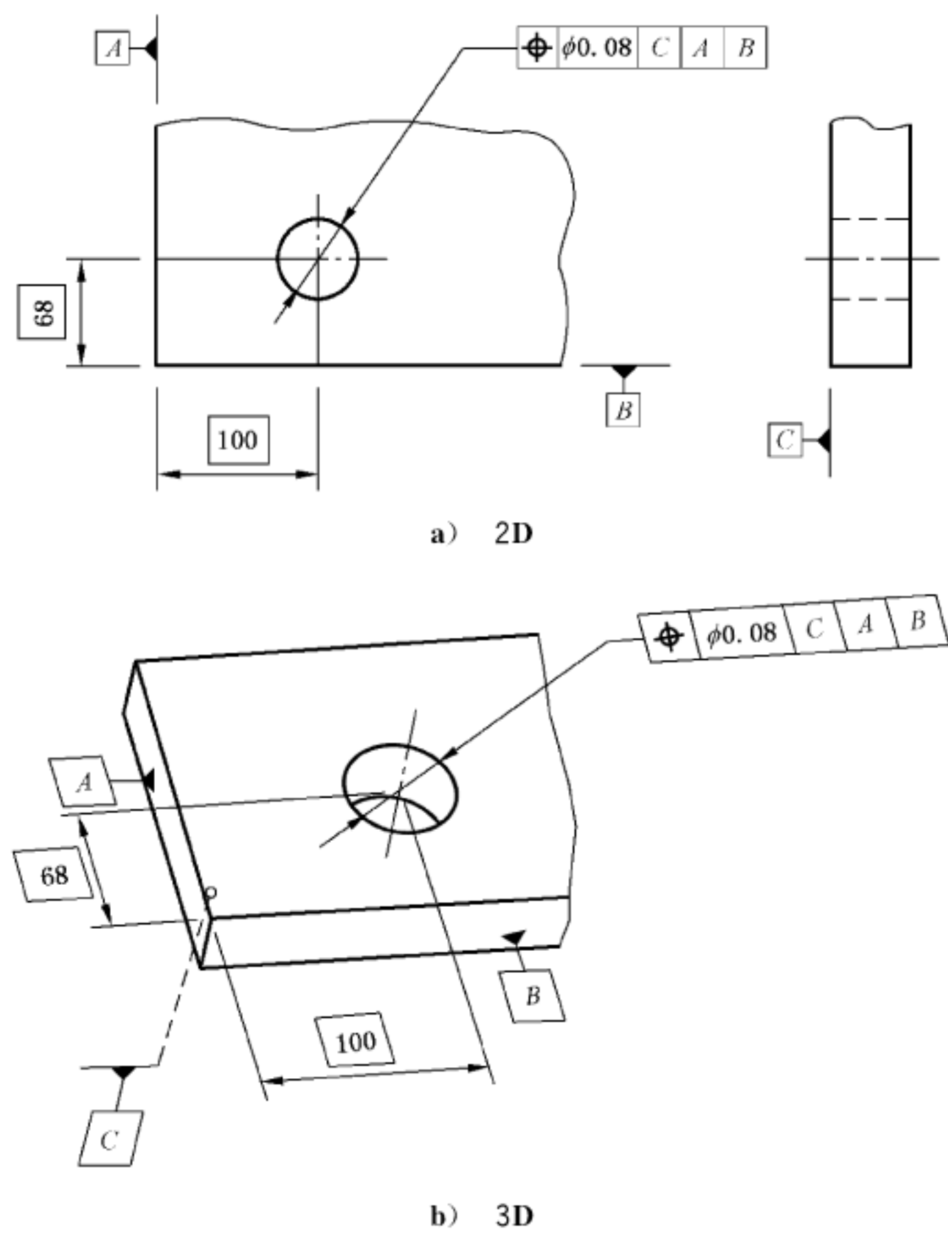
图 154 位置度标注
