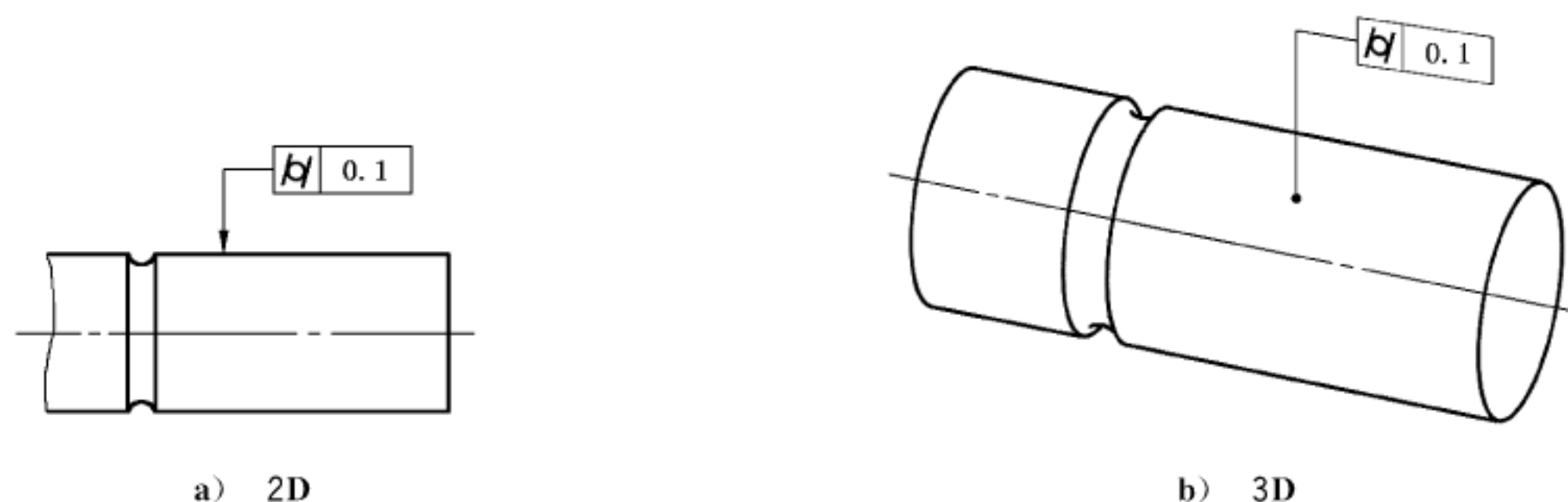
图 102 圆柱度标注
