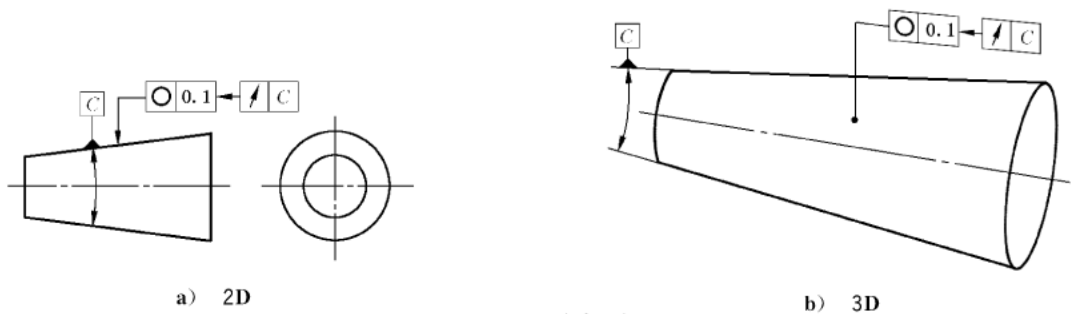
图 100 圆度标注
