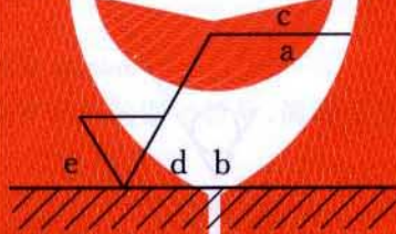
图 6 补充要求的注写位置(a~e)
