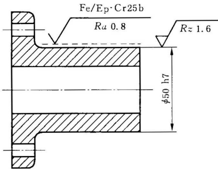
图 29 同时给出镀覆前后的表面结构要求的注法
