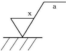
图 I.1 “x”和“a”的位置
