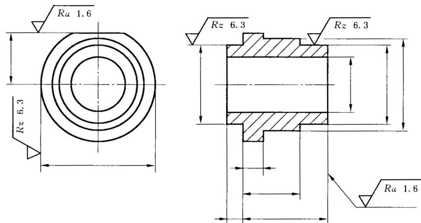
图 21 表面结构要求标注在圆柱特征的延长线上
