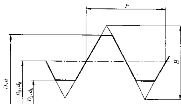
图 1 基本尺寸
