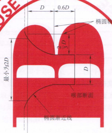
图 B.6 喷嘴
