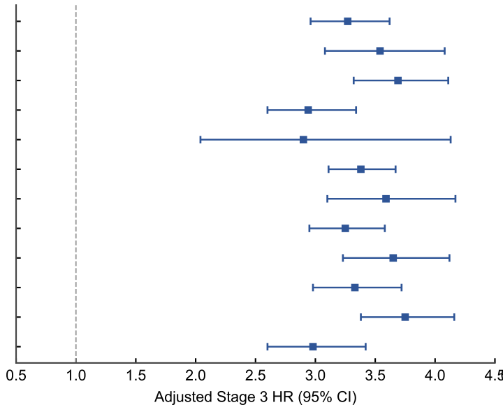
MIMIC-IV
