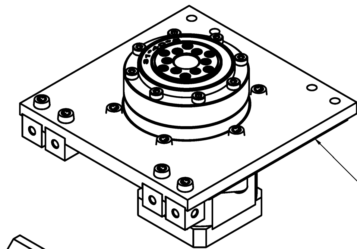
固定到安装板上的DEC轴
