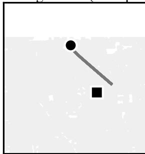
CascadeTraj (Ours)
