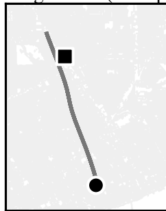
CascadeTraj (Ours)
