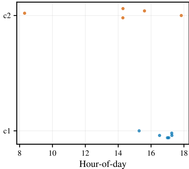
Time vs Top2 (AUC_time=0.57)
