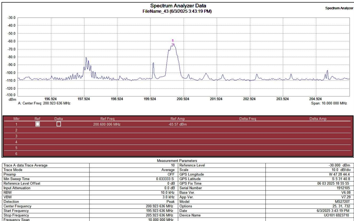
Figura 11 - Emissão em 2ª harmônica em 200,6 MHz sem modulação
