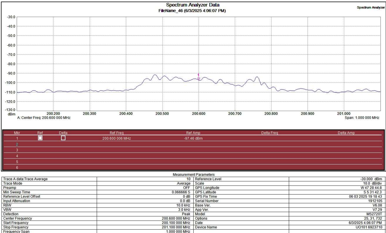
Figura 9 – Emissão em 2ª harmônica em 200,6 MHz (não conforme em relação à fundamental mesmo com modulação)
