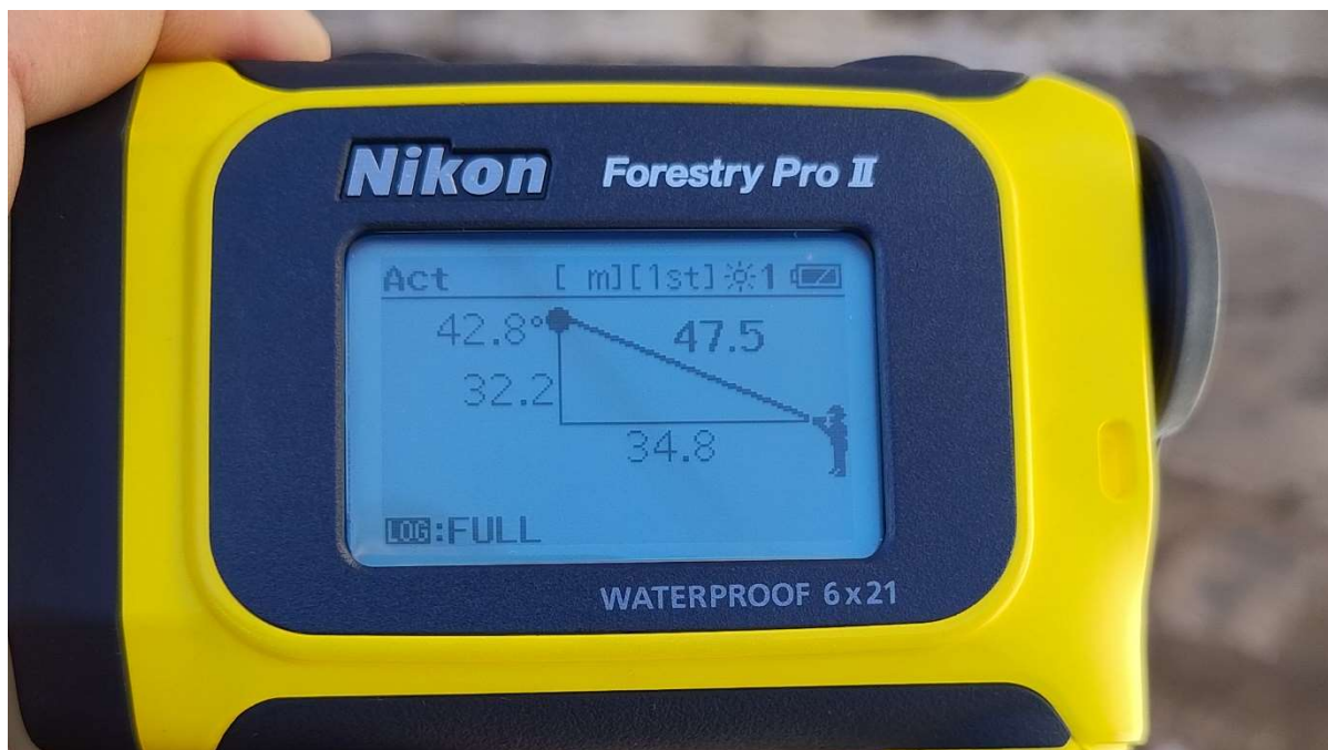
Figura 3 – Altura aproximada do centro geométrico das antenas em 32,2 metros
