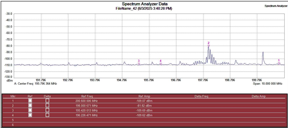
Figura 12 - Espectrograma apresentando sinais espúrios gerados pelo transmissor da entidade fiscalizada (marcas 1, 3 e 4)
