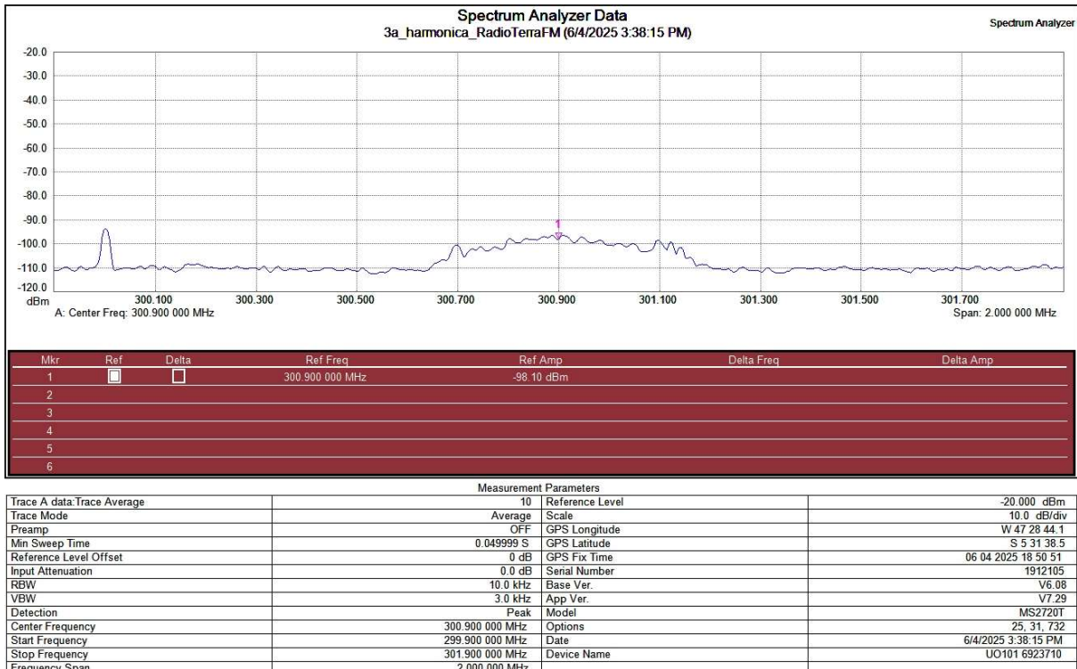
Figura 10 - Emissão em 3ª harmônica em 300,9 MHz (não conforme em relação à fundamental mesmo com modulação)
