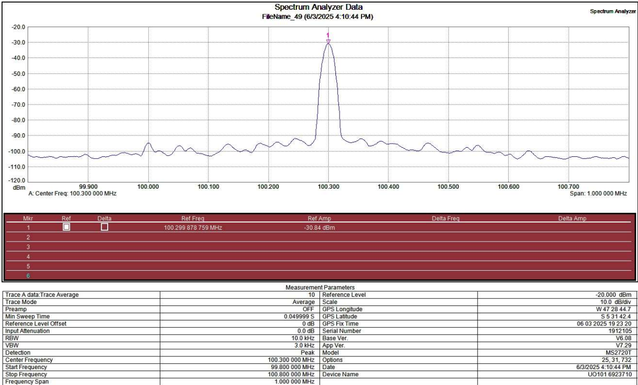
Figura 8 – Espectrograma da frequência central do canal 262 (marca 1, 100,3 MHz)
