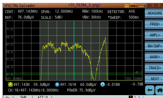
Imagem 4 - Tela do Analisador de Tv Digital Deviser S7200 destacando a portadora da estação.
