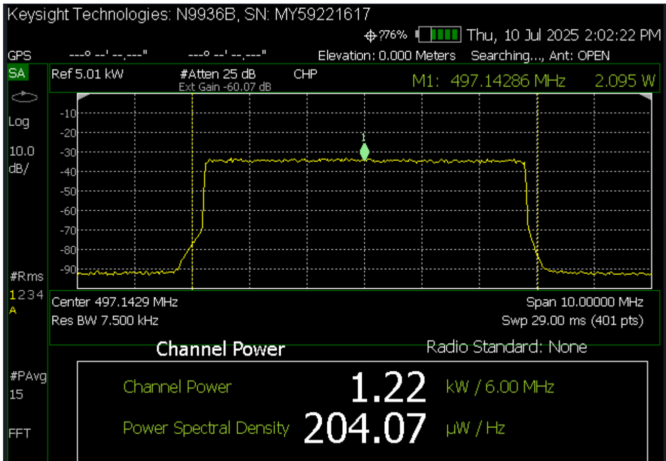
Imagem 1 - Tela do Analisador de Espectro destacando o canal da GTVD centralizado em 497,143 MHz e a potência de operação (1,22 KW) no momento da fiscalização.
