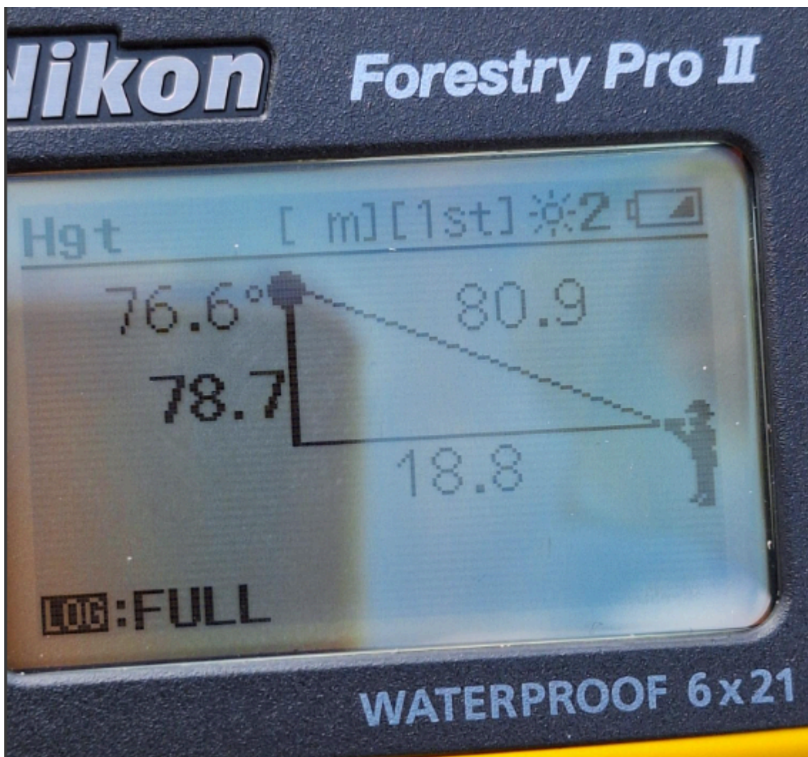
Imagem 2 - Indicação aproximada da altura da Antena Principal.
