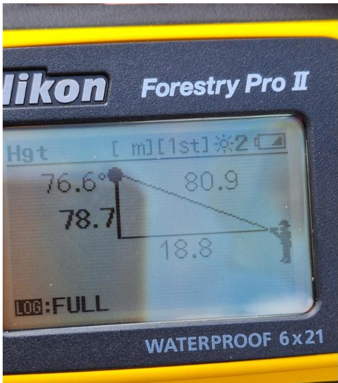
agem 5 – Telêmetro com a medida da altura da antena da estação.
