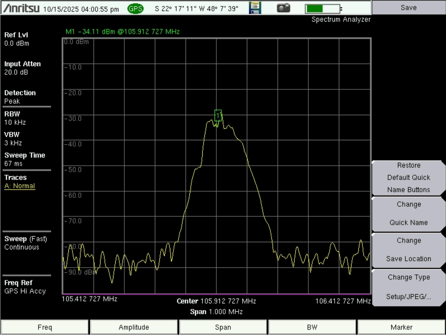
Figura 1 - Tela do analisador de espectro com o marcador na frequência de 105.9 MHz
