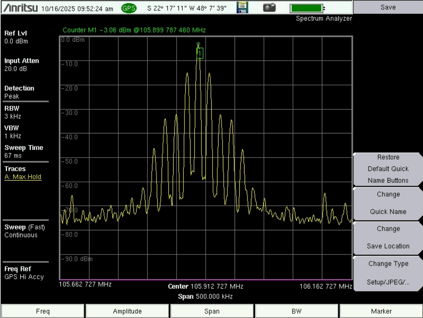
Figura 2 - Tela do analisador de espectro na frequência central de 105.9 MHz indicando desvio de -213 Hz
