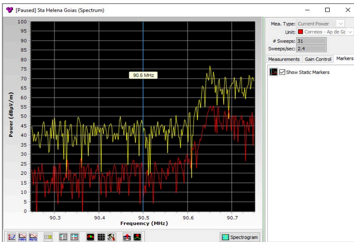
Figura 6 - Monitoração da frequência de 90,5 MHz com as estações da Anatel de Goiânia e Aparecida de Goiânia
