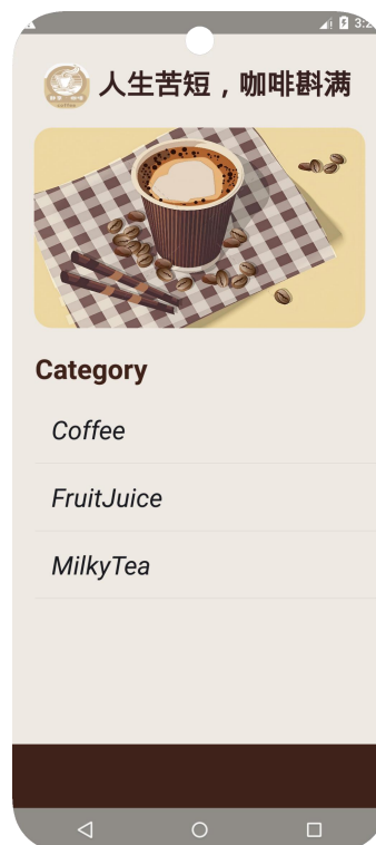
图 1 App 主界面
