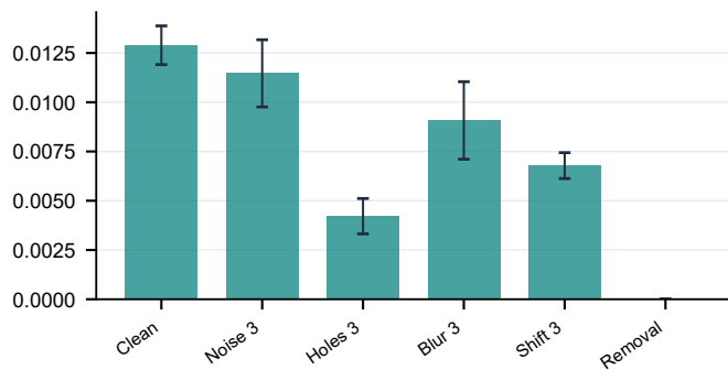
SIP
