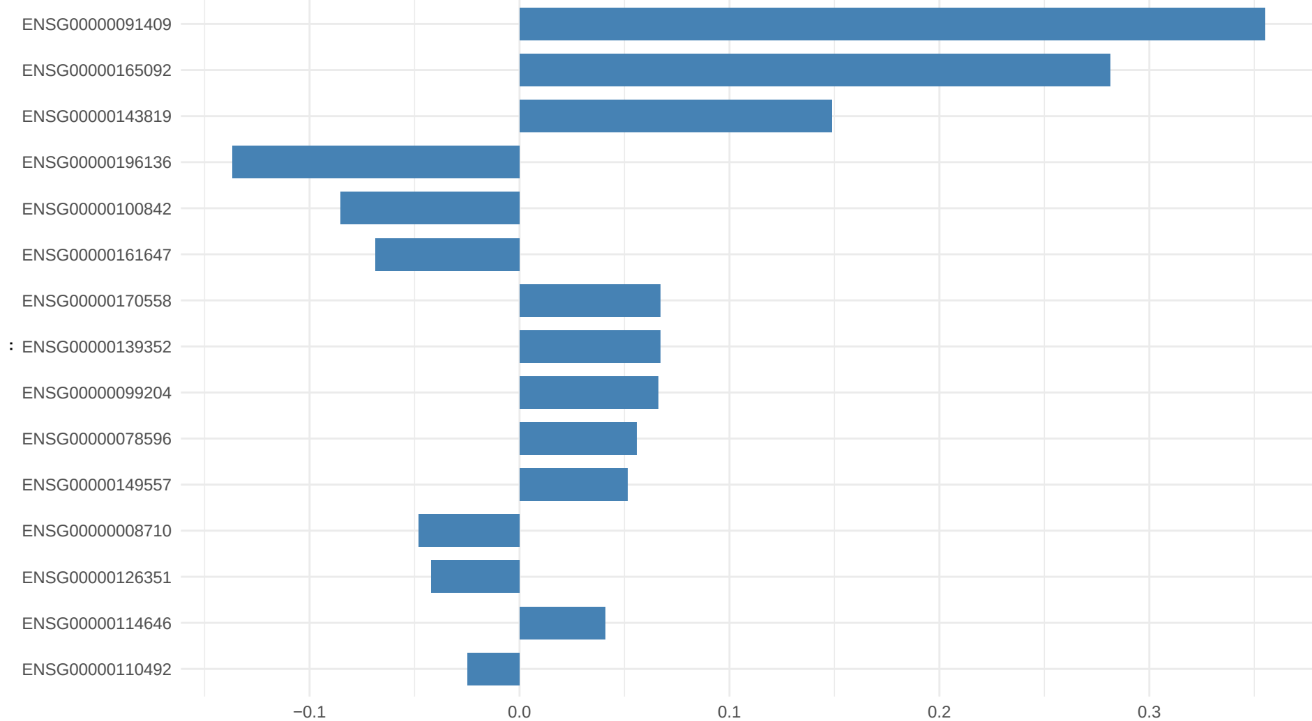
QR Trans-AdLASSO .....15.....JAM2... (t=0.5)
