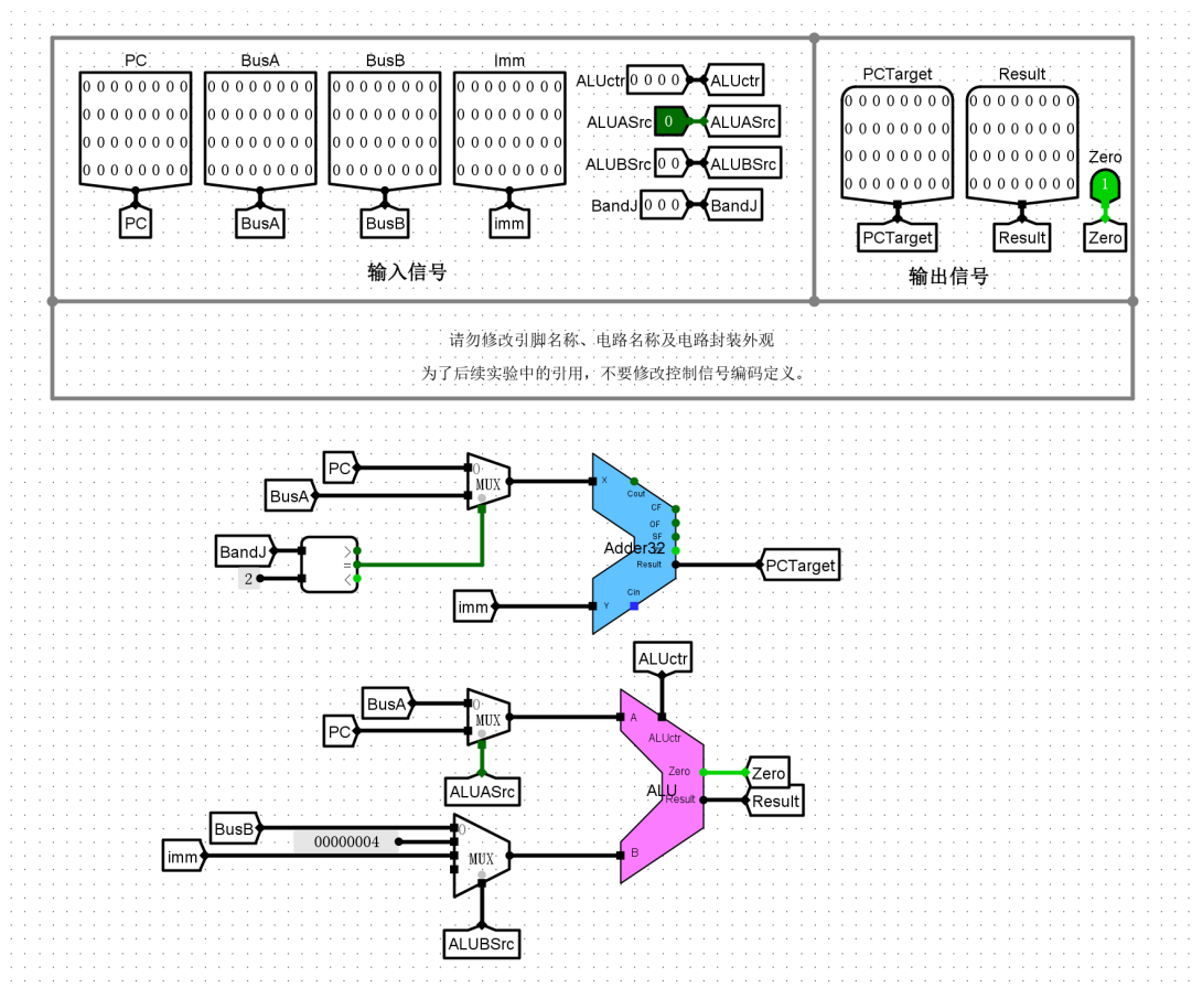
图 6: EU 模块电路图
