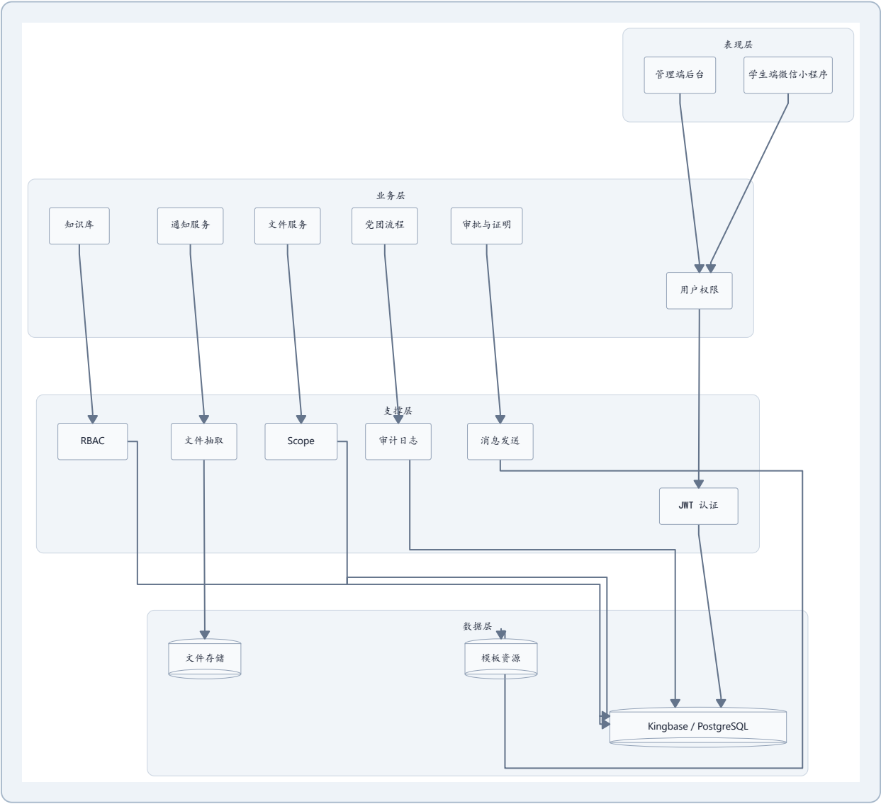
系统上下文图
