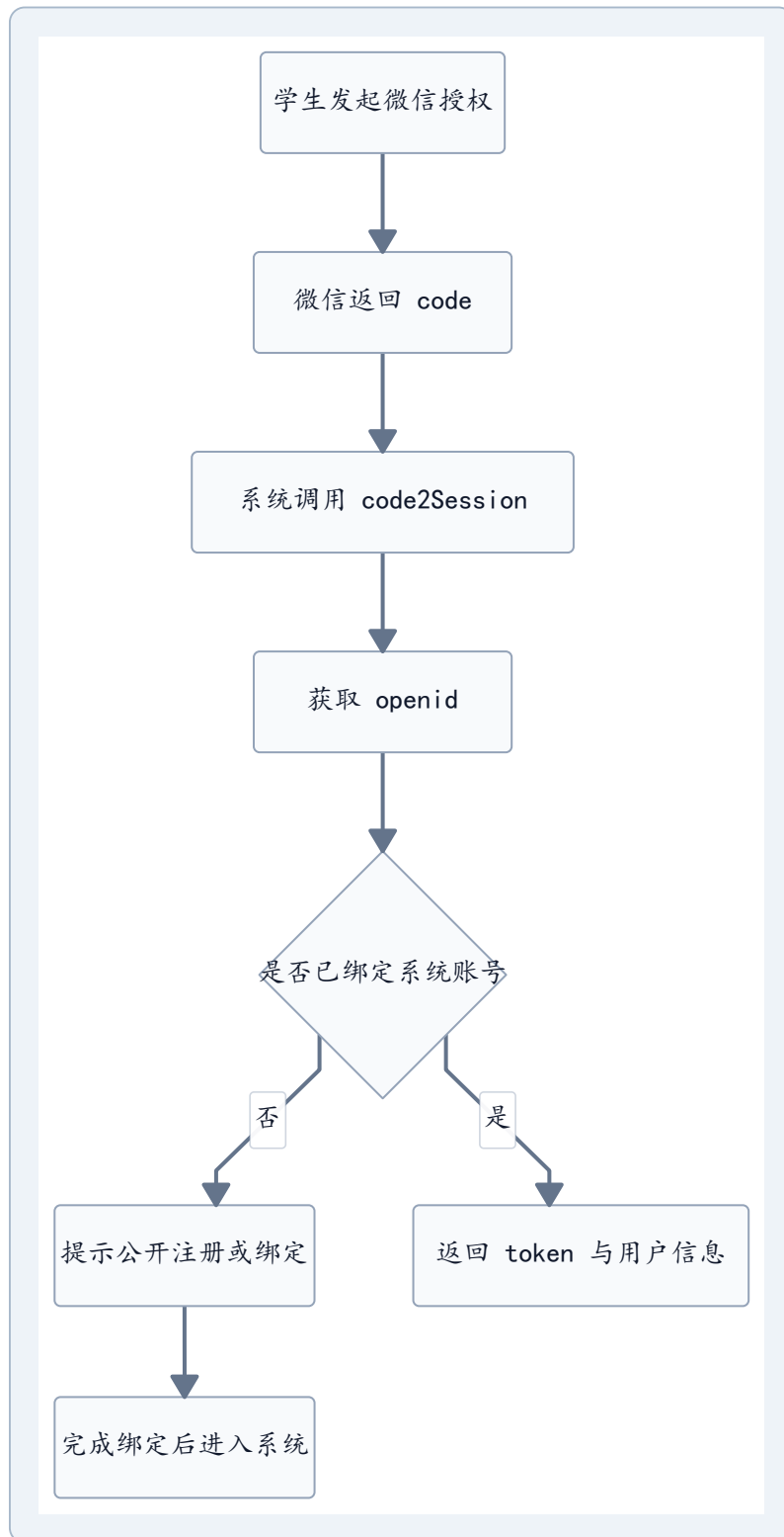
学生注册 / 登录业务流程图
