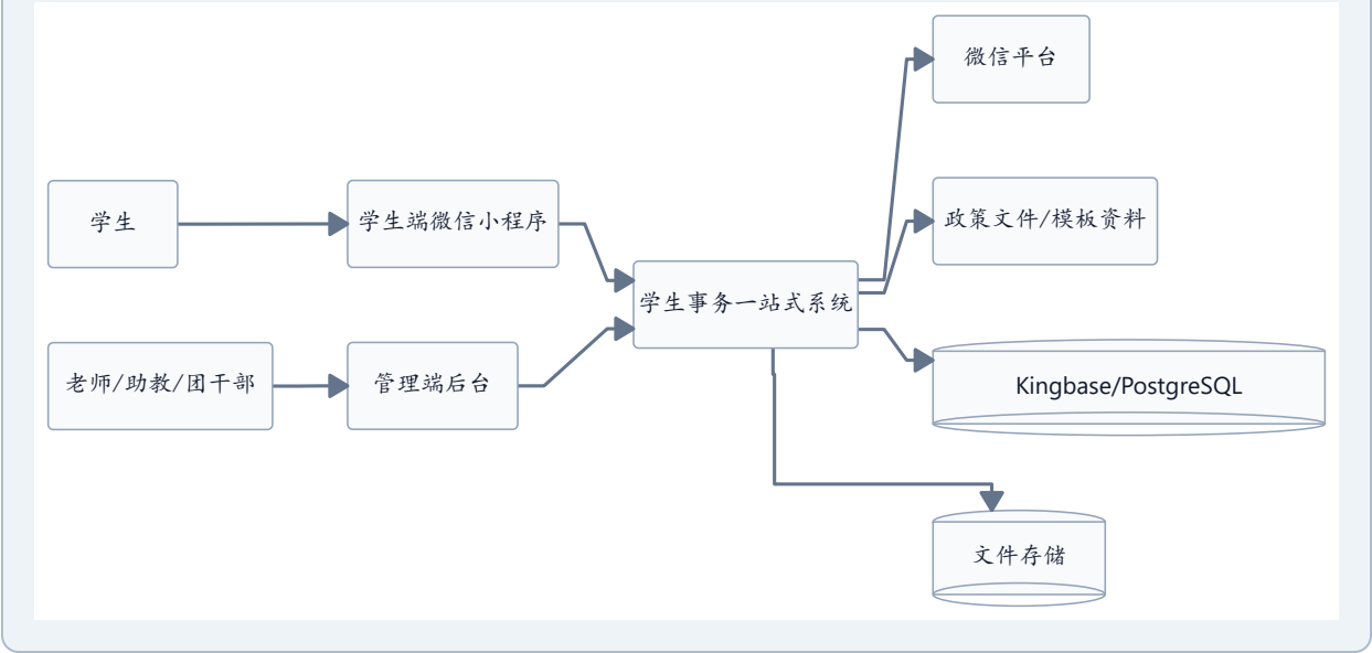
系统上下文图
