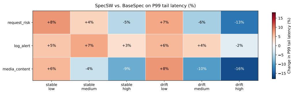
图 5-8 SpecSW 相对 BaseSpec 的 P99 变化热力图
