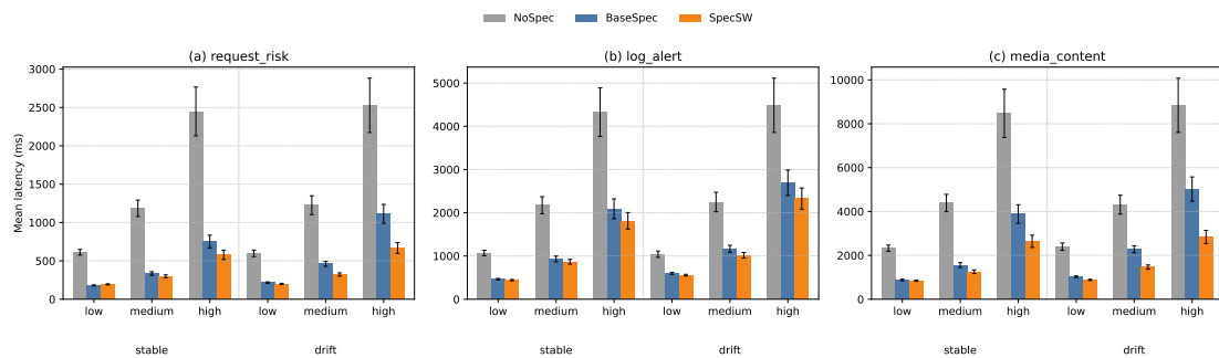
图 5-5 不同工作流与负载条件下三种方法的端到端平均时延比较
