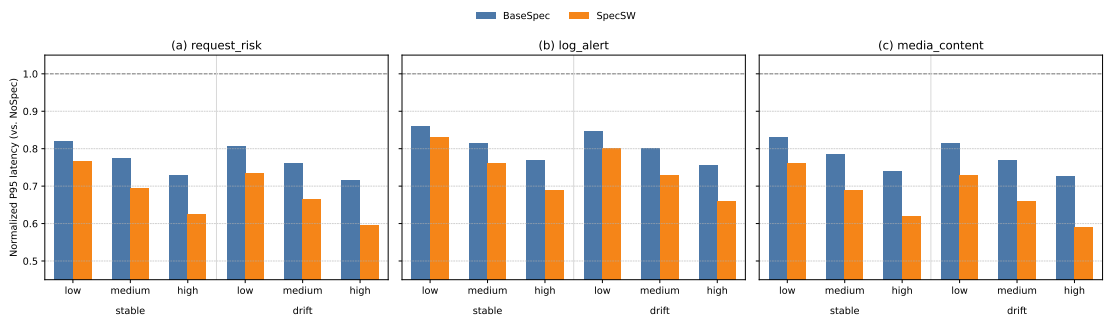
图 5-7 不同工作流与负载条件下三种方法的 P95 归一化时延比较
