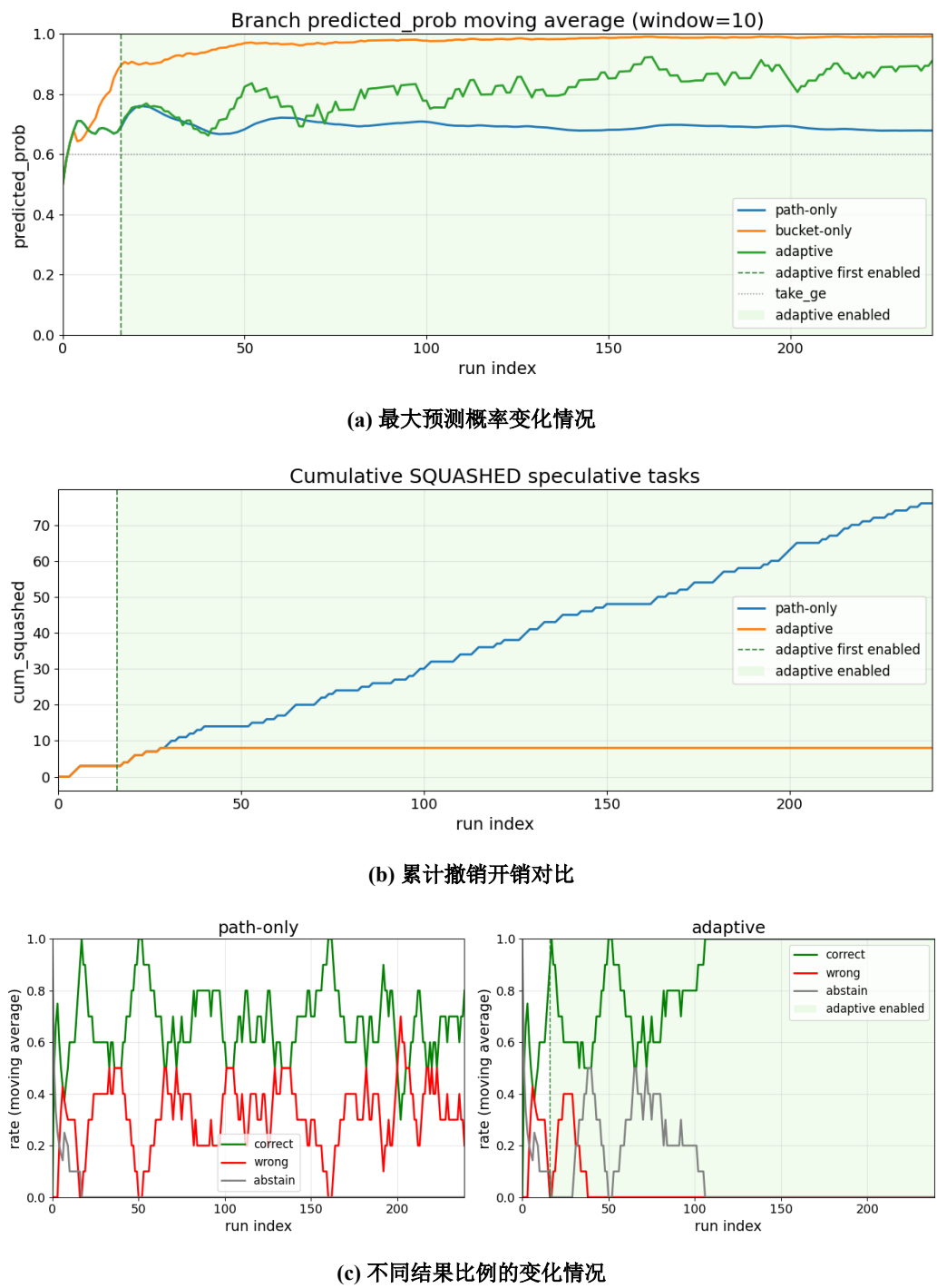
图 5-1 不同输入建模策略在输入驱动分支场景下的对比结果
