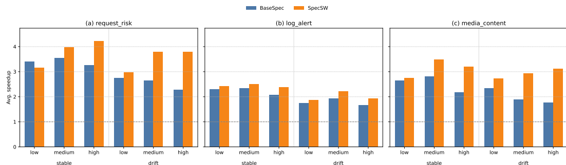
图 5-6 不同工作流与负载条件下投机方法的平均加速比
