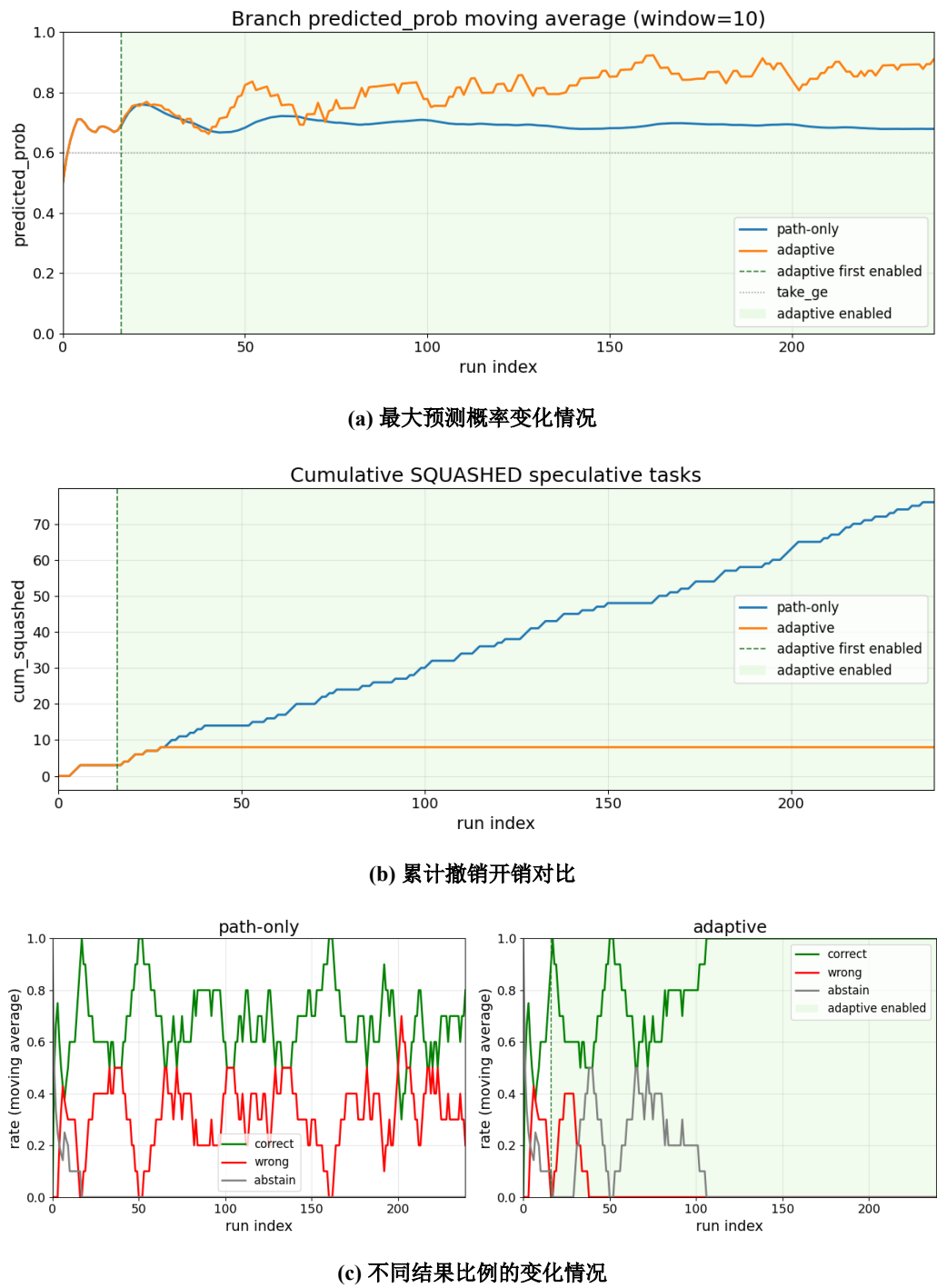
图 5-2 不同输入建模策略在输入驱动分支场景下的对比结果
