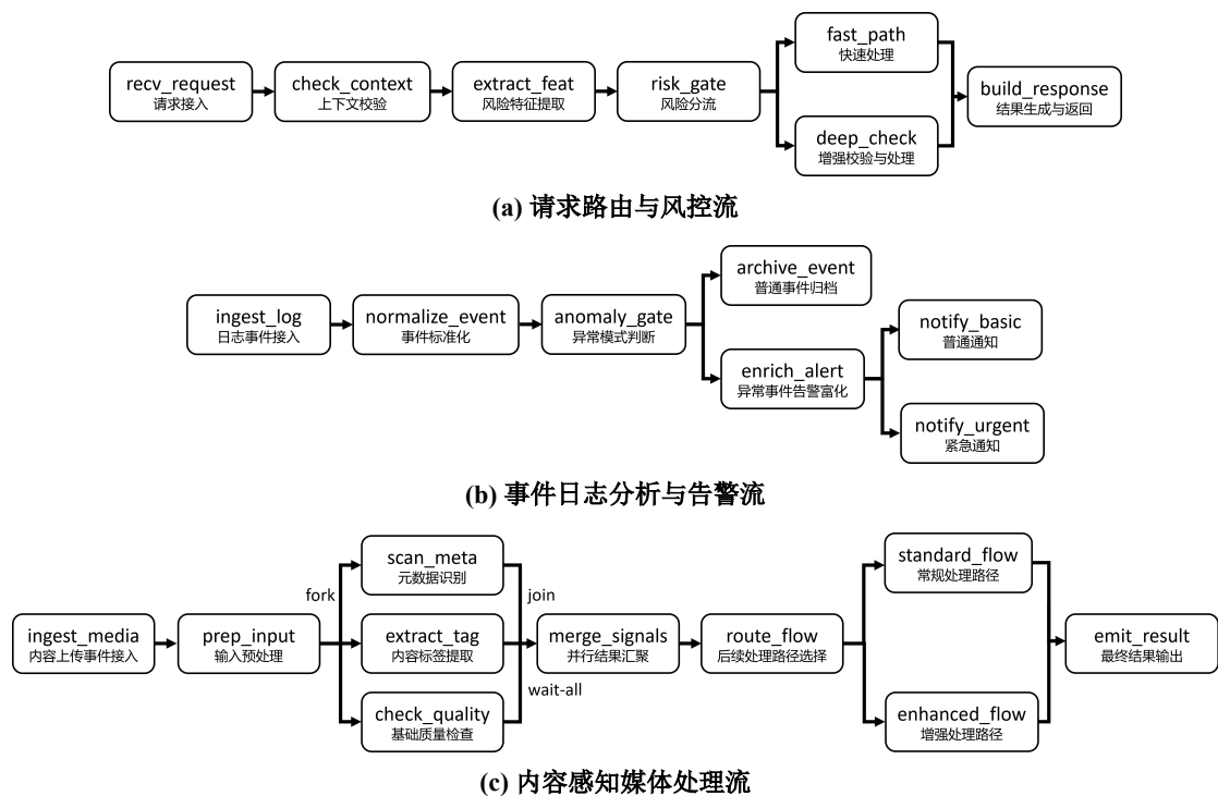
图 5-9 用于端到端性能评估的三类 workflow 结构
