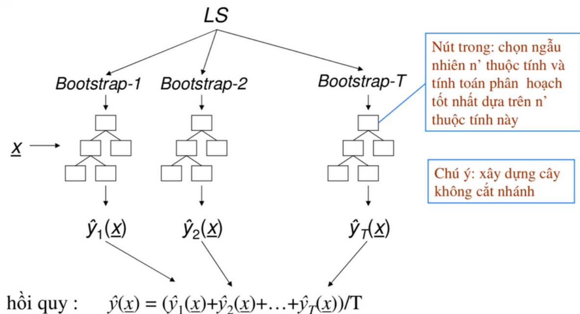
Hình 7: Random Forest
