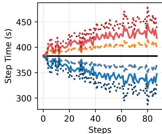
7B Drift Templates
