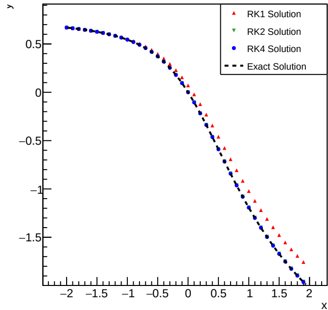
ODE demo
