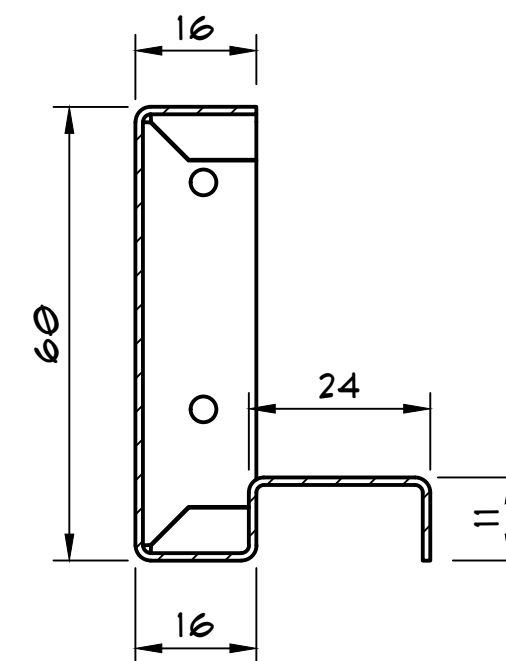
A-A (1:1)
