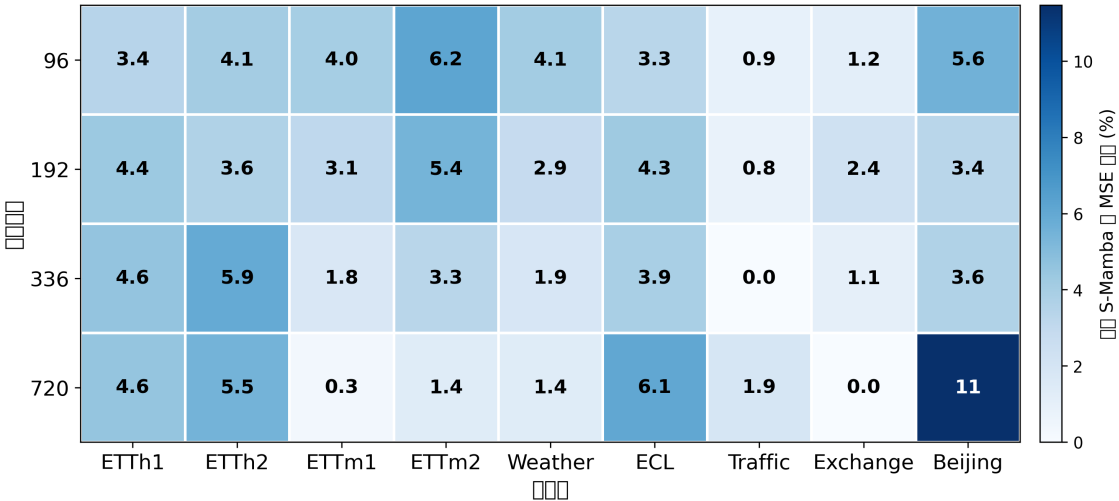
图 1 QCK-M 相对 S-Mamba 的 MSE 降低百分比（%）：行为预测长度、列为数据集，格内数字为降低幅度，颜色仅作参考。
