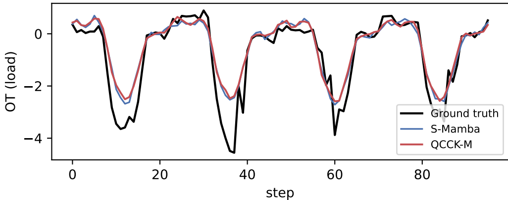
ETTh1, L=96
