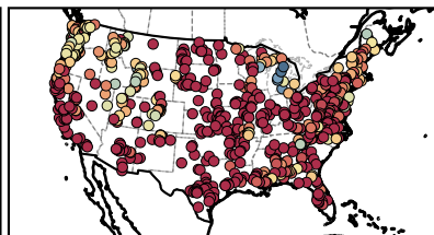
(f) NRMSE
