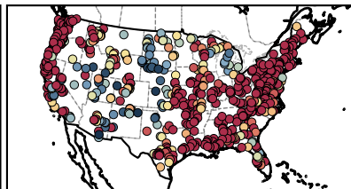
(f) NRMSE
