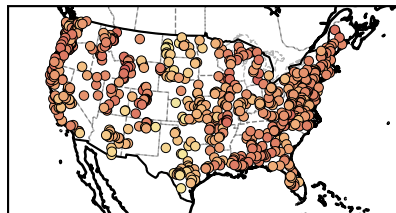
(d) NSE
