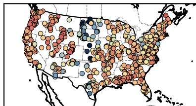
(d) NSE
